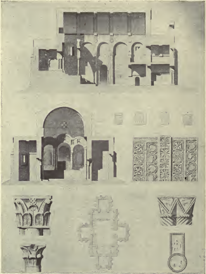
DETAILS OF HERMITAGE OF SANTA CRISTINA (CONCEJO DE LA POLA DE LENA) PROVINCE OF OVIEDO
