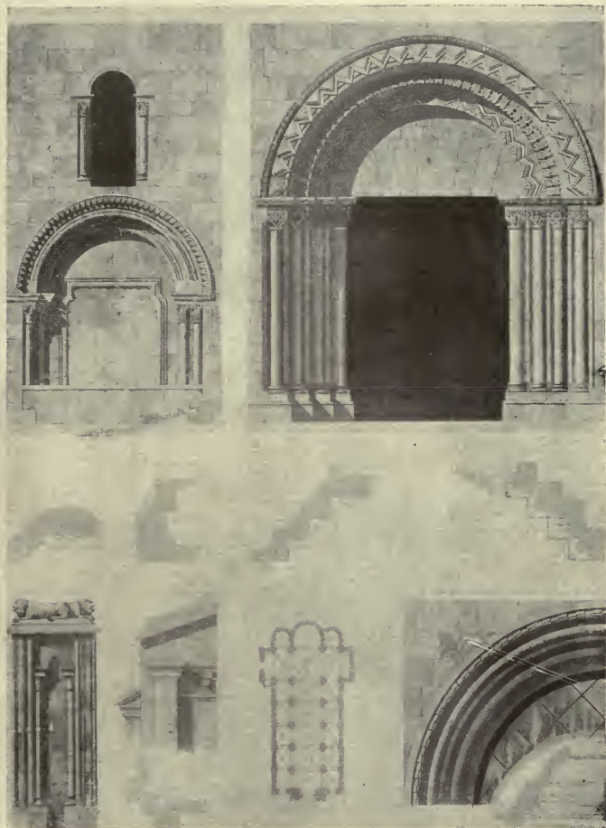
PLAN AND DETAILS OF SANTA MARIA DE VALDEDIOS (CONCEJO DE VILLAVICIOSA) PROVINCE OF OVIEDO
