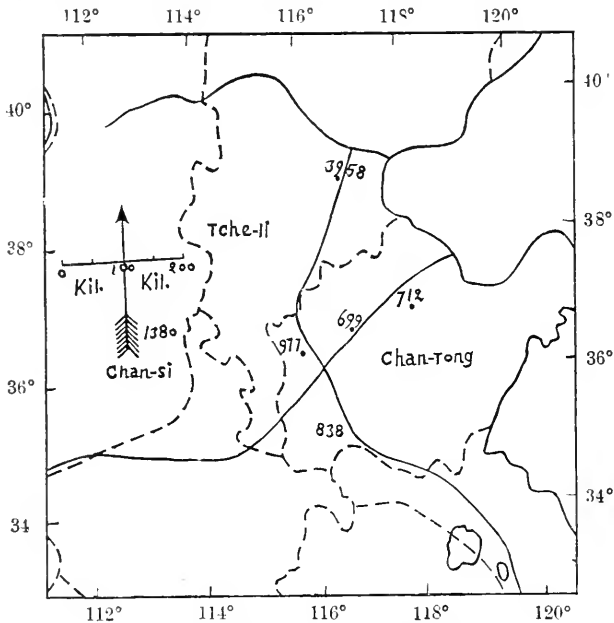
Fig. 114. N o 2934 et 2935. 14 Mai 1830.
