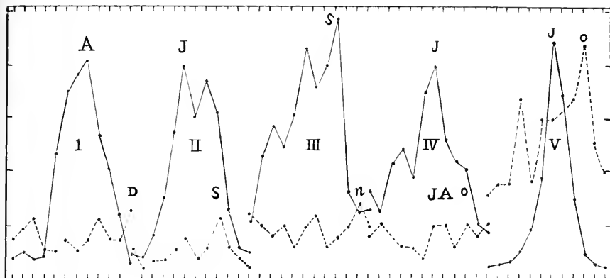
Fig. II. — Pluviosité (en pointillé) et fréquence sismique mensuelles pour: I, Yun-ran F.; II, Hong kong et Canton; III, Fou-tcheou; IV, Chang-hai; V, Pé king.
