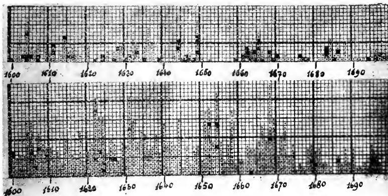
Fig. 72. Le XVII e siècle : activité sismique au Japon et en Chine.
