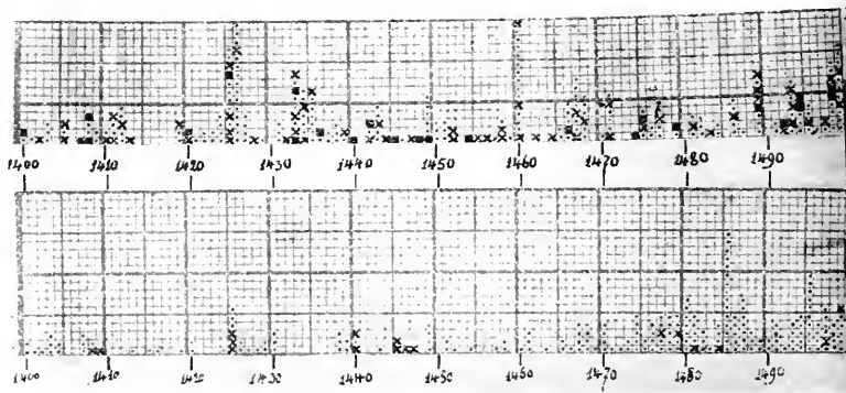
Fig. 13. Le XV e siècle: activité sismique au Japon et en Chine.
