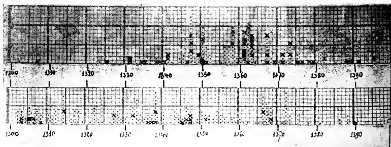
Fig. 36. Le XIV e siècle : activité sismique au Japon et en Chine.
