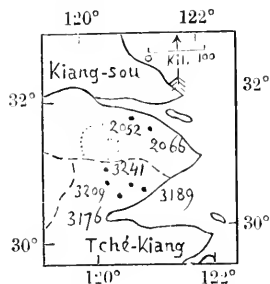
Fig. 51. N o 1031. 5 Octobre 1479.
