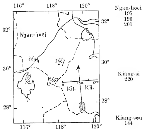
Fig. 105. N° 2694bis. 7 Décembre 1756.
