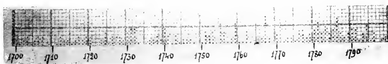
Fig. 93. Le XVIII e siècle : tremblements de terre destructeurs en Italie.
