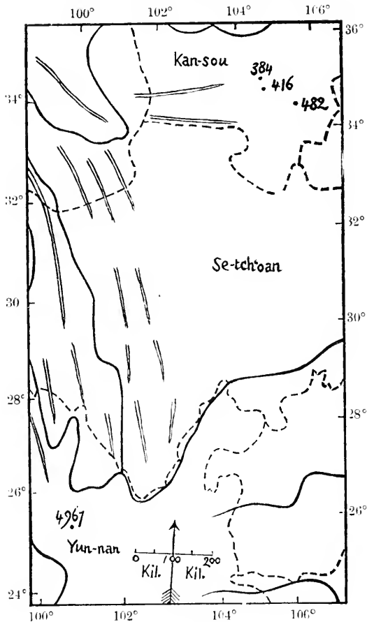
Fig. 38. N° 739. 25 e Juin 1308.
