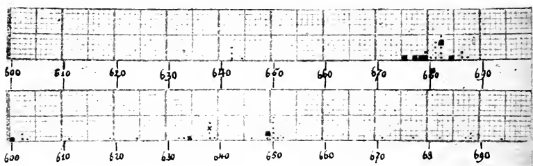
Fig. 7. Le VII e siècle : activité sismique en Chine et au Japon.
