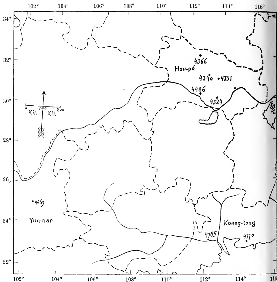
Fig. 75. N° 1894. 5 Mars 1620. (voir page 249.)
