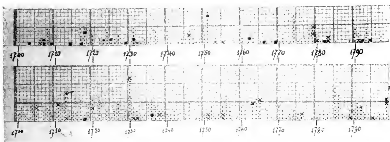
Fig. 92. Le XVIII e siècle : activité sismique au Japon et en Chine.
