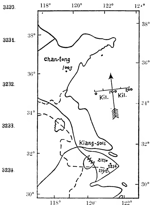
Fig. 134. N° 3228. 23 Octobre 1866 (voir p. 383).
