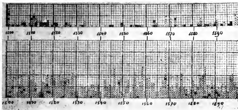
Fig. 57. Le XVI e siècle : activité sismique au Japon et en Chine.
