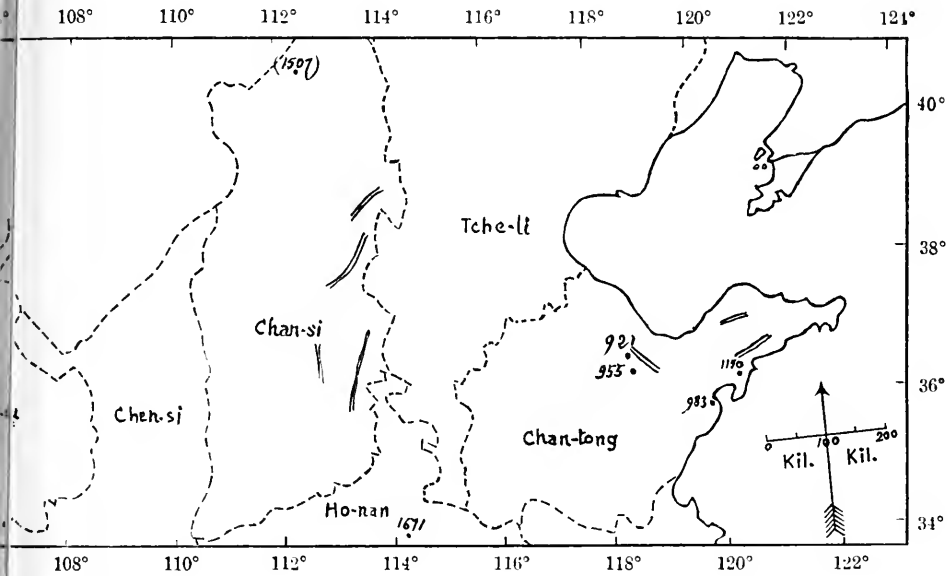
Fig. 1. N° 28. 1 Juin 70 av. J.-C.
