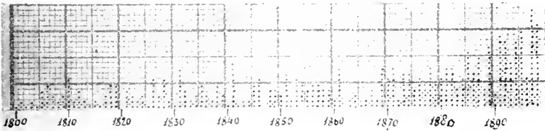
Fig. 110. Le XIX e siècle : tremblements de terre destructeurs en Italie.
