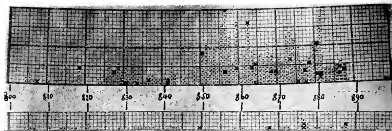
Fig. 16. Le IX e siècle : activité sismique au Japon et en Chine.
