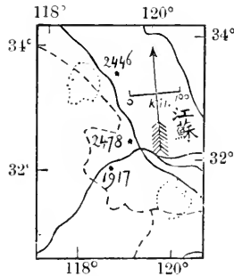
Fig. 55. N° 1088. 28 e Sept. 1491.
