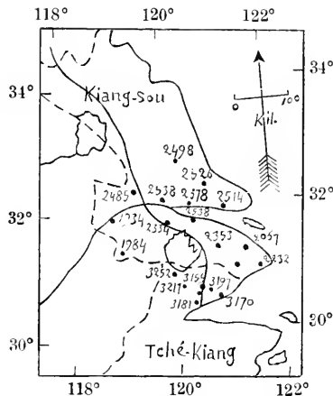
Fig. 76. N° 1945 bis . 10 e Février 1624.
