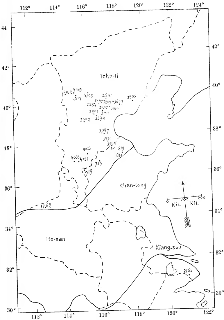
Fig. 89. N° 2438. 2 Septembre 1679. (voir p. 306.)
