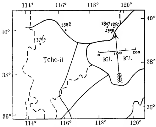
Fig. 87. N° 2412 bis . 18 Octobre 1673.
