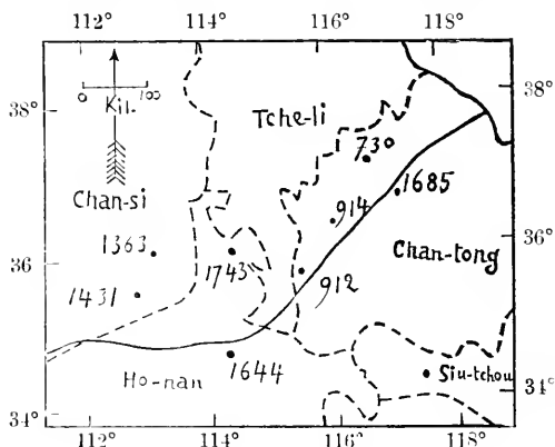
Fig. 60. N o 1149. 17 Octobre 1502.
