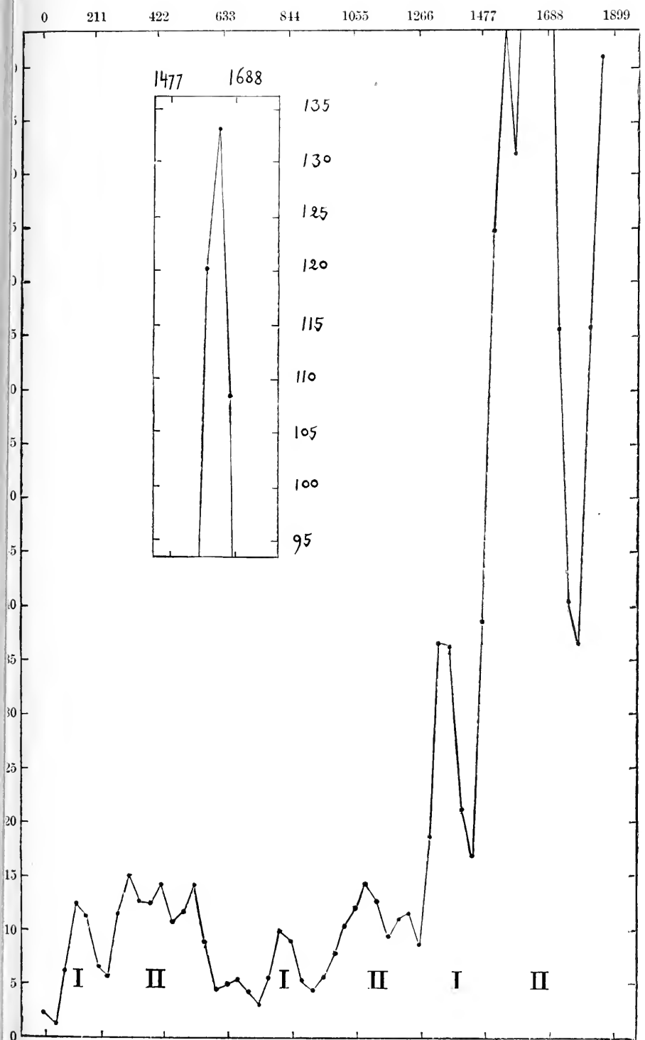
Fig. III. — Fréquence sismique de la Chine, de l'an 1 à 1899 ap. J.-C. (Dans chaque période de 633 ans, I et II marquent respectivement le passage d'une petite, puis d'une plus grande vague).
