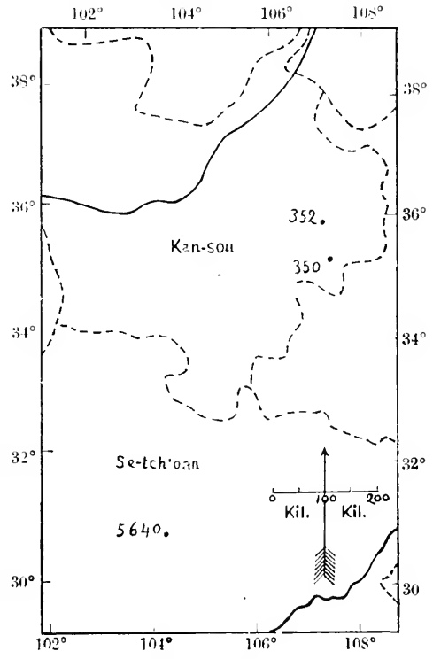
Fig. 25. N° 525 ter , 6 Octobre 1007.
