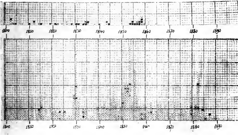
Fig. 109. Le XIX e siècle : activité sismique au Japon et en Chine.
