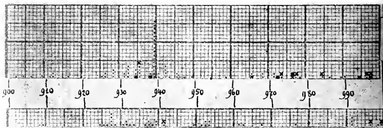
Fig. 20. Le X e siècle: activité sismique au Japon et en Chine.
