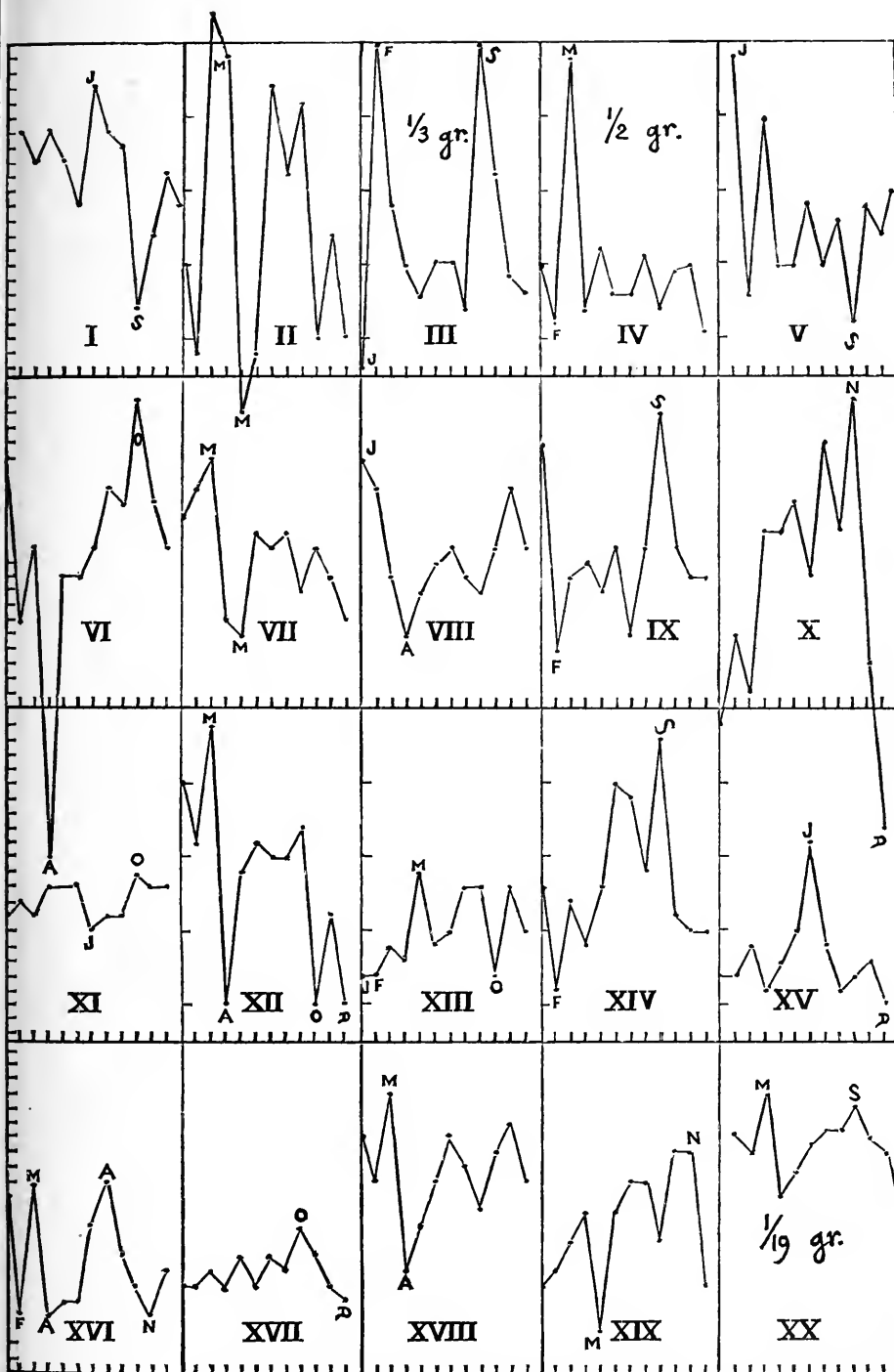
Fig. I. — Sismicité mensuelle : I, Chen-si ; II, Kan-sou ; III, Chan-tong ; IV, Chan-si ; V, Ho-nan ; VI, Kiang-sou ; VII, Ngan-hoei ; VIII, Kiang-si ; IX, Tché-kiang ; X, Tché-li ; XI, Cheng-king ; XII, Hou-pé ; XIII, Hou-nan ; XIV, Koang-tong ; XV, Koang-si ; XVI, Yun-nan ; XVII, Koci-tcheou ; XVIII, Fou-kien ; XIX, Se-tch'oan ; XX, Chine totale. (Les mois remarquables sont signalés par leurs initiales).
