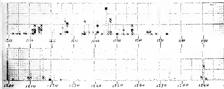
Fig. 33. Le XIII e siècle : activité sismique au Japon et en Chine.
