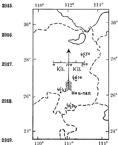
Fig. 111. N° 2912. 5 Déc. 1825. (voir p. 351.)
