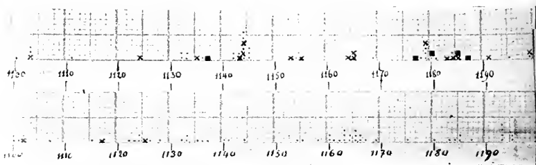
Fig. 29. Le XII e siècle : activité sismique au Japon et en Chine.
