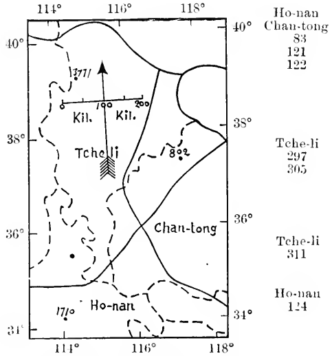
Fig. 90. N° 2462 et 2462 bis . 22 Nov. 1683.
