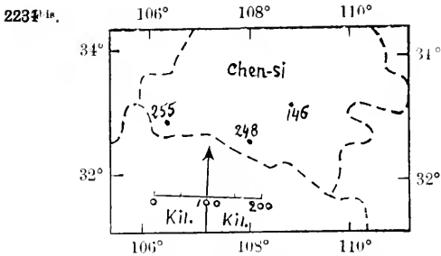
Fig. 80. N° 2234 bis . 22 Juin 1654.
