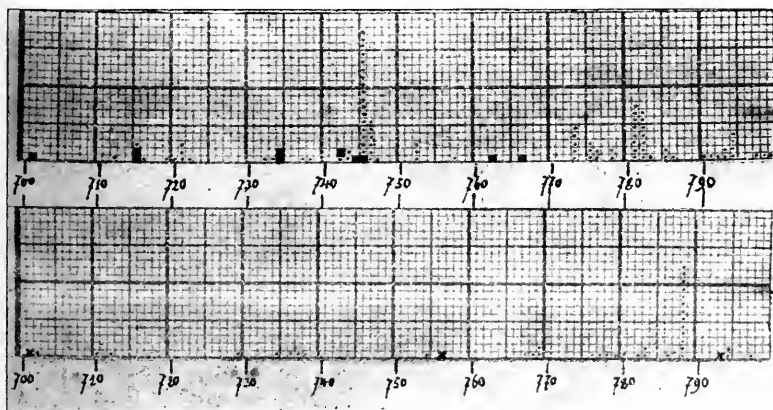
Fig. 10. Le VIII e siècle : activité sismique au Japon et en Chine.
