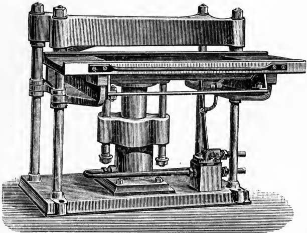
FIG. 35. Cake Moulding Press (Fr. Krupp).
