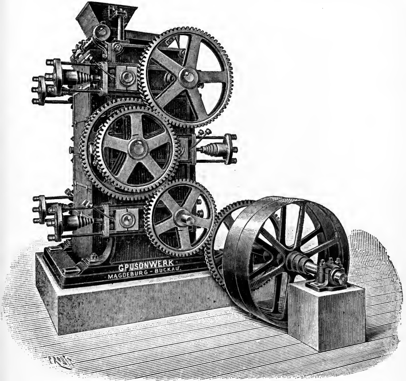
FIG. 23. Roller Mill (Fr. Krupp).
