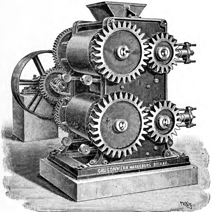
FIG. 24. Two-pair Roller Mill (Fr. Krupp).
