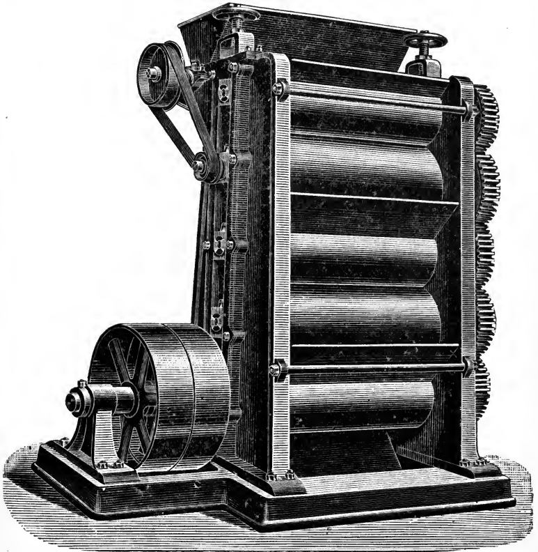
FIG. 21. Seed Crusher (Anglo-American Pattern).
