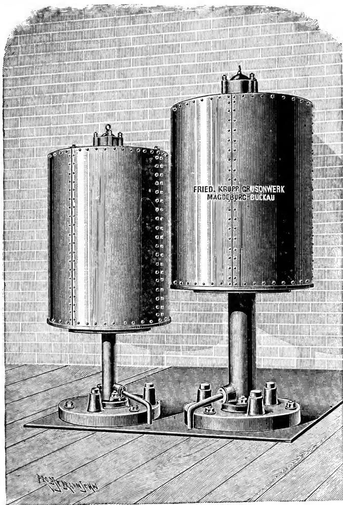
FIG. 34. Accumulators (Fr. Krupp).
