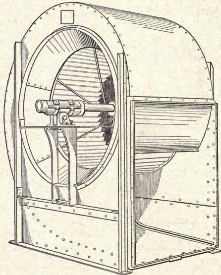
Fig. 138—Multivane Fan
