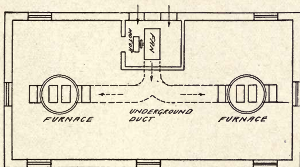
Fig. 129—General Plan
