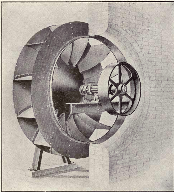
Fig. 53—A Cone Fan
