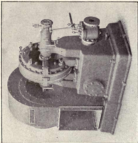
Fig. 65—Turbine Fan
