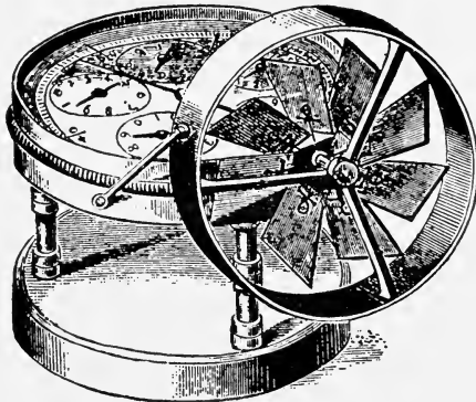
Fig. 6—An Anemometer
