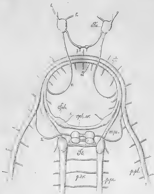
Fig. 4. Nervensystem von Chiton.
