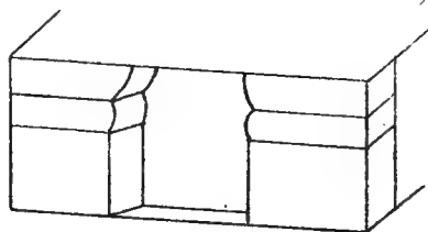
Fig. 2. (bedeelte van het subasfement der Tjandi-toen (Schetssteekening)
