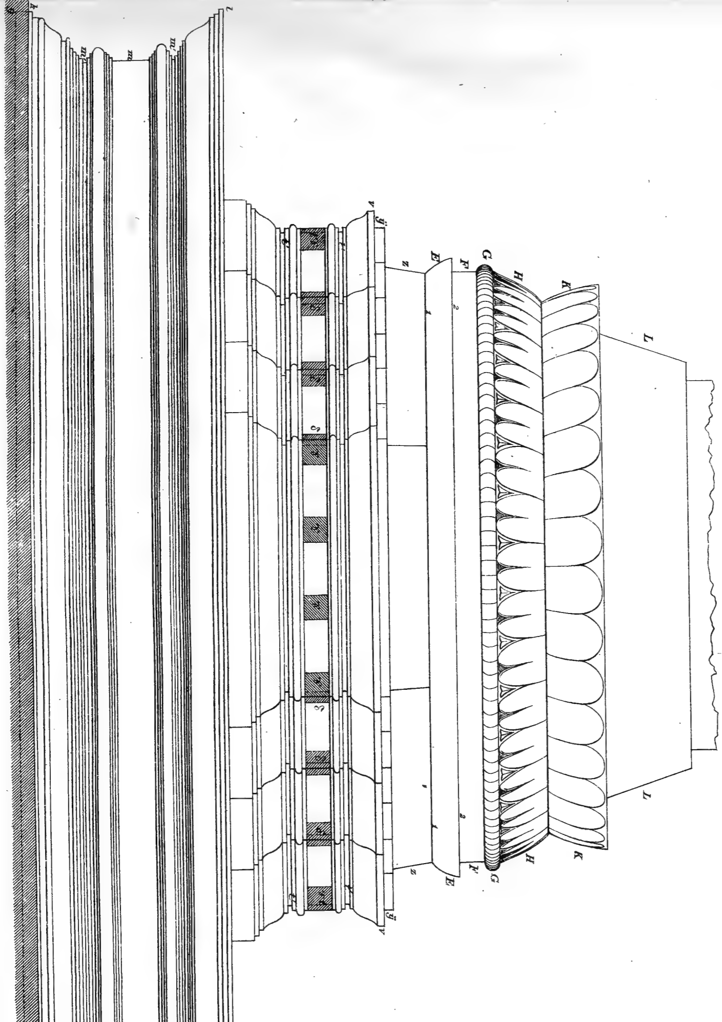
Fig. 5 C. Verticale Projectie, op een vlak evenwijdig aan AC van Fig.
