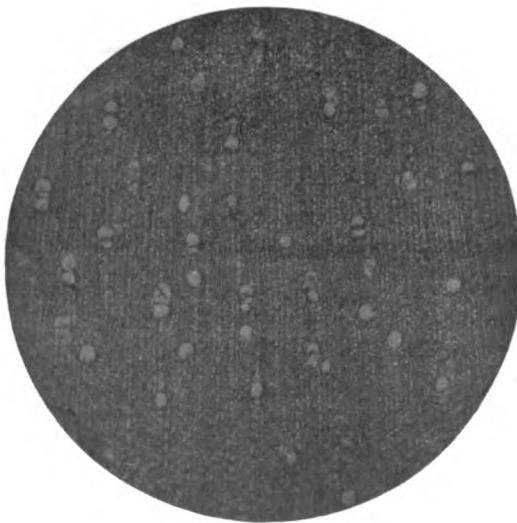
Fig. 35. Kickxia elastica , 5 \frac{1}{2} jährig. Querschnitt, Mikrophotographie.
