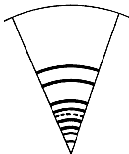
Fig. 59. Hevea brasiliensis Nr. VI. Schematischer Querschnitt oberhalb der Ringelung. Radius 20 mm. 1\frac{1}{2} fach vergr.
