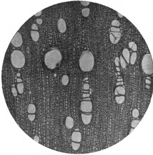
Fig. 31. Strophantus dichotomus . Querschnitt, Mikrophotographie.
