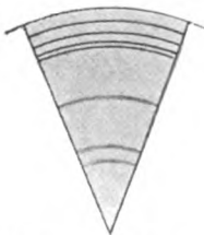
Fig. 22. Coffea arabica ( maragogy ), 8jährig. Querschnittsschematisch. Radius 27 mm. Natürl. Größe.
