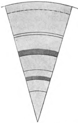
Fig. 16. Coffea aleocuta , 12jährig. Querschnitt schematisch. Radius 55 mm. Natürl. Größe.
