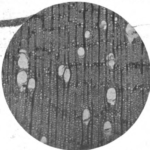
Fig. 39. Palaquium borneense , 5jährig. Querschnitt mikroskopisch.
