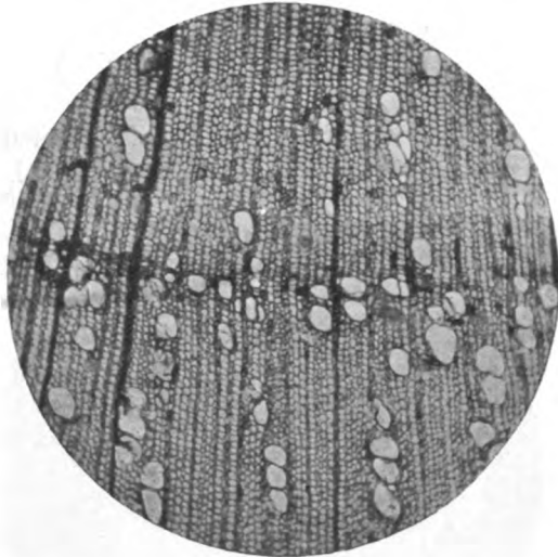
Fig. 37. Palaquium oblongifolium , 10jährig. Querschnitt, Mikrophotographie.
