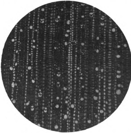
Fig. 21. Coffea arabica ( maragogy ), 8jährig. Querschnitt, Mikrophotographie.
