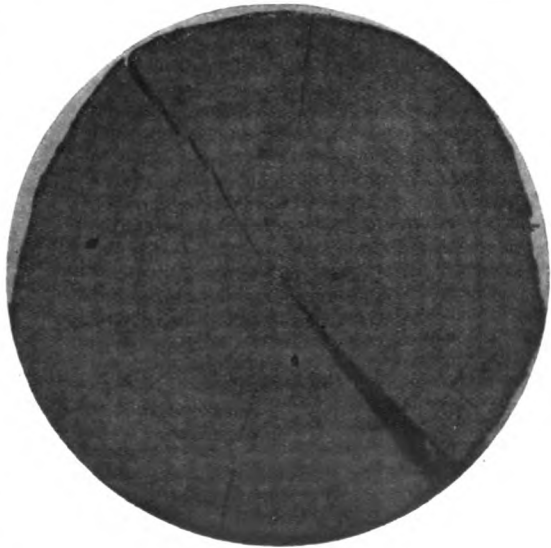
Fig. 8. Coffea aleocuta , 12jährig. Querschnitt makroskopisch.
