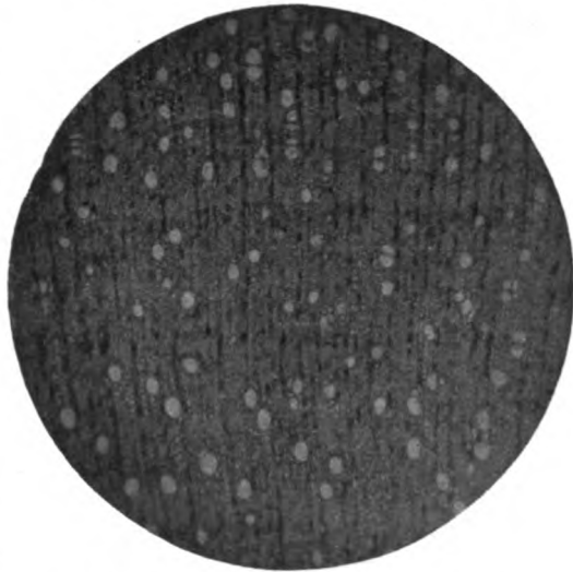
Fig. 2. Erythroxylon coca ; 15jährig. Querschnitt mikroskopisch.
