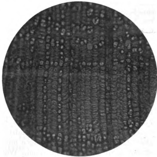
Fig. 46. Hevea brasiliensis , I. Querschnitt mikroskopisch (Zelluloseschicht).
