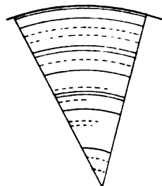
Fig. 4. Erythroxyylon coca , 5 jährig. Querschnitt schemat. Radius 12 mm. 3fach vergrößert.
