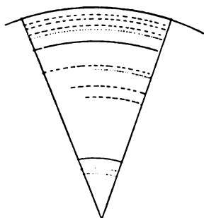
Fig. 5. Erythroxyylon coca , 6jährig. Querschnitt schematisch. Radius 13 mm. 3fach vergrößert.
