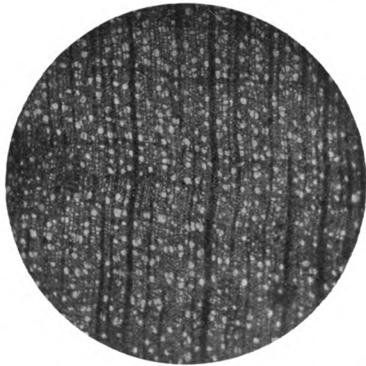
Fig. 26. Thea assamica , 14jährig. Querschnitt, Mikrophotographie.
