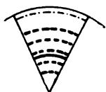
Fig. 54. Hevea brasiliensis Nr. IV (geschnitten), vom oberen Teil des Stammes.
