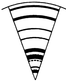
Fig. 47. Hevea brasiliensis I, normal, d. h. ohne Störung gewachsen. Querschnitt schematisch. Radius 17 mm am unteren Teil des Stammes. ■■■■ = Zelluloseschicht.
