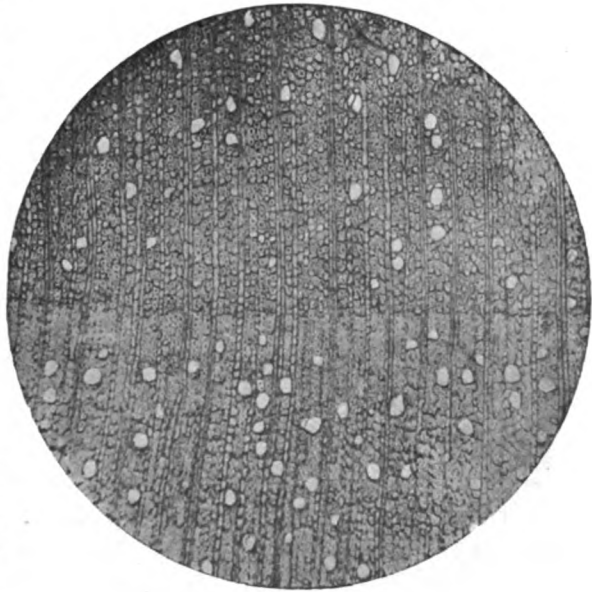
Fig. 15. Coffea aleocuta , 9jährig. Querschnitt, Mikrophotographie.
