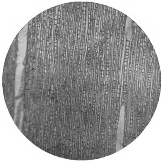
Fig. 30. Strophantus dichotomus . Tangentialschnitt, Mikrophotographie.
