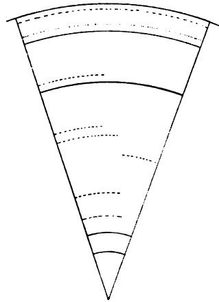
Fig. 7. Erythroxylon coca , 15jährig. Querschnitt schematisch. Radius 28 mm. 2fach vergrößert.
