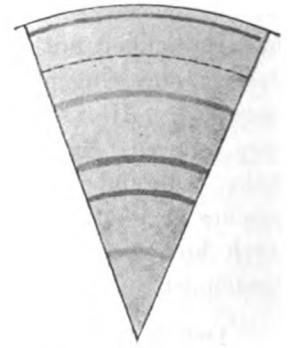
Fig. 18. Coffea quillou , 6jährig. Querschnitt schematisch. Radius 44 mm. Natürl. Größe.
