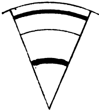
Fig. 13. Coffea Laurentii (robusta) , 6 jährig. Querschnitt schemat. Radius 28 mm. Natürliche Größe.
