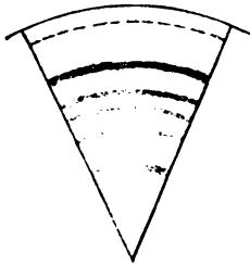
Fig. 23. Coffea excelsa , 5jährig. Radius 31 mm. Natürliche Größe.
