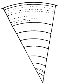
Fig. 3. Erythroxyylon coca , 4 jährig. Querschnitt schemat. Radius 16 mm. 3fach vergrößert.
