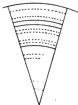
Fig. 6. Erythroxyylon coca , 7jährig. Querschnitt schematisch. Radius 14 mm. 3fach vergrößert.
