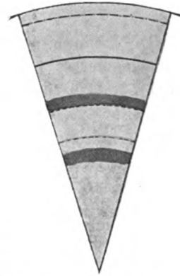
Fig. 14. Coffea aleocuta , 9jährig. Querschnitt schematisch. Radius 50 mm. Natürl. Größe.
