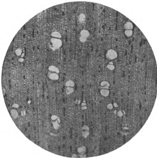
Fig. 28. Theobroma Cacao , 6jährig. Querschnitt, Mikrophotographie.
