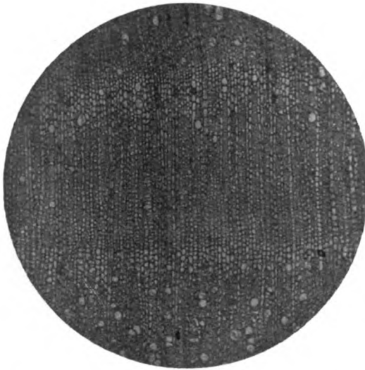
Fig. 9. Coffea stenophylla , 6jährig. Querschnitt mikroskopisch.
