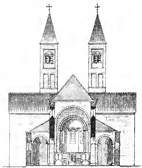
DOORSNEDEN OBER DE BREEDTE.
