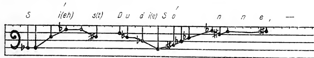
Fig. 44. Sprechmelodien verschiedener Satzformen.
