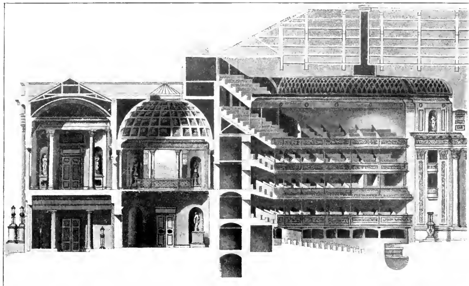
Abb. 72 Das Drury-Lane-Theater in London Querschnitt
