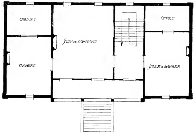
Abb. 205 Casino à l'italienne in Paris Grundriß
