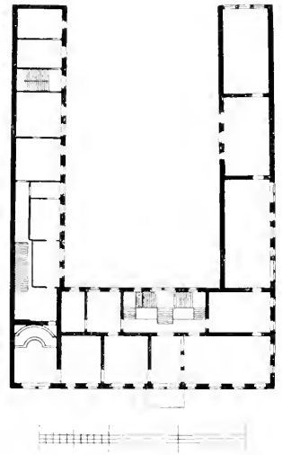
Abb. 213 Palais des Grafen Redern in Berlin Grundriß
