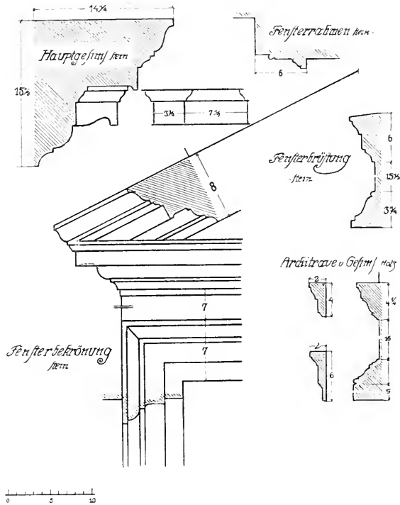
Abb. 229 Architektureinzelheiten in Bath
