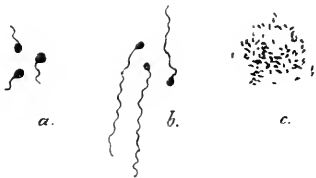
Fig. 23. Salpeterbakterien nach Winogradsky. a Nitrosomonas europaea (Nitritbakterien von Zürich), b Nitrosomonas javanensis (Nitritbakterien von Java), c Nitrobacter (Nitratbakterien aus Quito). Vergr. 1000.
