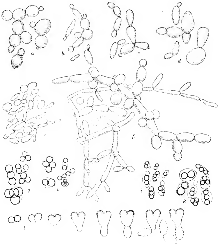
Fig. 25. Saccharomyceten (Sprosspilze). a Saccharomyces cerevisiae Nr. 1. b Sacch. Pasteurianus Nr. III. c Sacch. ellipsoideus (Weinhefe) Nr. 1. d Sacch. ellips. Nr. II. e und f Hautwuchs des Sacch. ellipsoideus Nr. 1 e bei 34—20 oder 6—7°, f bei 15—30° (Sprossmycelium). g—k Sporenhaltige Zellen. g Sacch. cerevisiae 1. h Sacch. Pasteur. 1. i u. k . Sacch. ellipsoid. 1 u. II. l Keimung von zwei freien Sporen des Sacch. Ludwigii bei 18—20° von links ab nach 18, 20, 26, 28, 29, 30 \frac{1}{2} und 33 Stunden. Alle Kulturen in Bierwürze, nach E. Chr. Hansen , Vergr. 1900.
