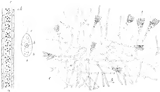
Fig. 15. a Oscillaria tenuis (Cyanophyceae), Fadenstück, ch hohleylindrisches Chromatophor (Farbstoffkörper), c sog. Centralkörper. Hauptmasse des teinvakuoligen Protoplasmas mit stark färbaren Körnern (schwarz). b Polytona uvella . Flagellate mit zwei Geißeln am Vorderende. v kontraktile Vakuole, k Zellkern, h Zellhaut, der Inhalt mit Assimilationsprodukten (kleinen Ringen, Paramylum) erfüllt. c Penicillium glaucum (echter Pilz, Mycomycet). Mycelstück aus einer ausgekeimten Conidie ( a ) entstanden, an besonderen in die Luft ragenden Ästchen neue pinselförmige Conidienträger ( b ) mit Conidienketten. Vergr. a 2250, b circa 600, c (nach Brefeld) 120.
