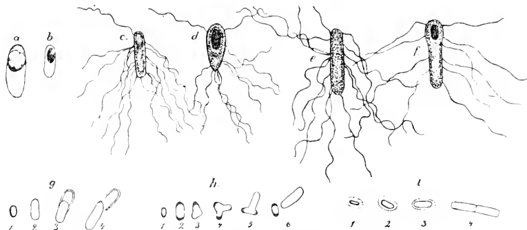
Fig. 11. Sporenentwicklung und Keimung. a Milzbrandbacillus, dessen Inhalt sich zum jungen, noch hautlosen Sporenkörper zusammengezogen hat. b Reife Spore des Milzbrandes, noch eingeschlossen in das Stäbchen, dessen Gestalt während der Sporenbildung sich nicht verändert. c u. d Clostridium butyricum (Prazm.), c vegetatives peritriches Stäbchen, d reife Sporen in der spindelförmig aufgeschwollenen Zelle, deren Inhalt nicht ganz zur Sporenbildung aufgebraucht wird. e u. f Plectridium paludosum , e unverändertes Stäbchen, f kopfig angeschwollen (Kaulquappenform, Stecknadelform) mit reifer Spore im dicken Ende. g Keimung der Sporen von Bacillus Anthracis , das Keimstäbchen streckt sich parallel zur Längsachse der kurzellipsoidischen Spore hervor, h , 4 (nach Prazmowski). h Keimung der Spore von Bacillus subtilis , Streckung des Keimstäbchens senkrecht zur Längsachse der Spore (3—5); wie beim vorigen schlüpft es schliesslich aus der Sporenhaut (6) hervor (nach Prazmowski). c Bacillus leptosporus . Die Spore, von einem zarten Gallerthof (punktiert 1—3) umgeben, streckt sich zum Stäbchen, ohne dass eine besondere Sporenhaut zurückbleibt (4); einfachste Art der Sporenkeimung (nach Klein) Vergr. a 2250, b — f circa 1200. g — i 1000.
