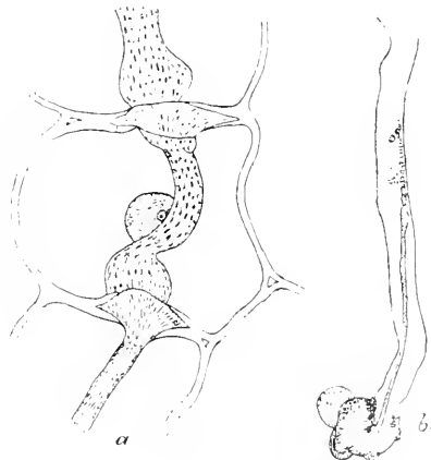
Fig. 21. Einwanderung der Bakterien in die Leguminosenwurzel. a Eine Zelle aus der Wurzelrinde der Erbse mit Zellkern und sog. Infektionsschlauche, einem breiten Strom einer dicht gedrängten Bakterienzooeciole, die durch die Zellwände sich hindurchschiebt (nach Prazmowski ). b Ende eines Wurzelhaares der Erbse, an dessen Spitze einige kleine Erdteilchen (rechts) kleben und Bakterien (links) sich angesammelt haben. Im Innern der Spitze dichtes Protoplasta untermengt mit Bakterien, die als fädige Zooeciole (Intektionstaden) in dem Haar emporenwandern (nach B. Frank ). Vergr. a 650, b 175.
