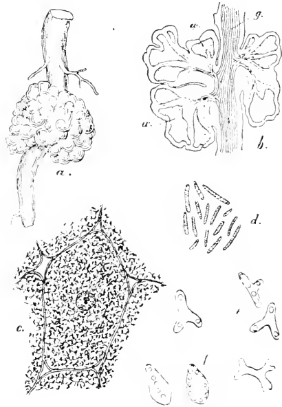
Fig. 19. Wurzelknöllchen der Leguminosen. a Wurzelknöllchen der Lupine in natürlicher Grösse (nach Woronin ). b Längsschnitt durch eine Lupinenwurzel mit Knöllchen; g das Wurzelgefässbündel, von dem aus nach allen Teilen des Knöllchens und seinen bakterienreichen Zellgruppen ( x ) feine Aestchen abgehen (starke Lupinenvergrösserung, nach Woronin ). c Eine Zelle eines Lupinenknöllchens, vollgestopft mit Bakterien (schwarz), zwischen denen ein zarteres Gerüst des Protoplasmas der Lupinenzelle sichtbar ist. Nach einem Mikrotomschnitt (Fixierung mit Flemmingscher Lösung, Färbung nach Gram ). d Knöllchenbakterien der Lupine, noch unverändert. e u. f Bakteroiden von Vicia villosa und Lupinus albus (nach Morck ). Vergr. c 600, d — f circa 1500.
