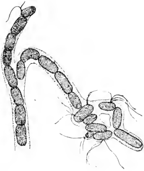
Fig. 12. Cladothrix dichotoma , Schwärmerbildung. Die feinpunktierte Scheide hat sich am linken Aste geöffnet und entlässt einen Schwärmer, am rechten Aste ist eine ganze Gruppe von Fadengliedern in Schwärmer mit je einem seitlichen Geißelbüschel umgewandelt. An diesem Aste ist die Scheide stark aufgelockert, verquollen. Vergr. 1000.
