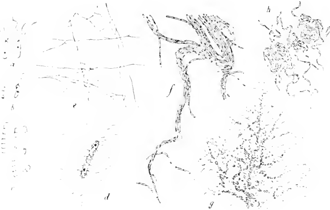
Fig. 22. Fäulnisbakterien. a Bactridium pseudotermo , der Cohnsche Beschreibung des alten Bacterium Termo am meisten entsprechend, b Vibrio aus fauligem Wasser, choleraähnlich, c Bacillus ureae , der häufigste Erreger der Harnfäulnis und wohl dem Micrococcus ureae Pasteurs entsprechend, d–h Bactridium Proteus ( Bacillus vulgaris , Bacterium Zopfi , Proteus vulgaris etc.). d peritriche Stäbchen, e spinnwebig feinfädiger oder mycelartiger Wuchs ( Zoogloea ) auf Gelatine, ganz schwach (50 mal) vergrössert, f stärker (300) vergrösserte gewundene Fäden und Fadenbänder solcher mycelartiger Massen, g schöner Bäumchenwuchs auf Gelatine mit knorrigen und wurstförmigen Anschwellungen, 50 mal vergrössert, h Stücke des vorigen Bildes 300fach vergrössert, um die Verschlingung der Fäden zu den Anschwellungen der mycelartigen Zoogloea zu zeigen. Vergr. a–d circa 1500, e u. g 50, f u. h 300.
