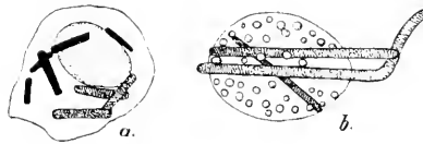
Fig. 29. Phagocytose nach Metschnikoff . a Leukoeyt aus Taubenblut mit Milzbrandbazillen, die zum Teil noch intakt sind und sich kräftig färben (schwarz), zum Teil mehr oder weniger verändert und blass (punktiert), der locker punktierte Körper ist der Zellkern. b Ein lebender Taubenleukoeyt, Bazillen in sich aufnehmend. Vergr. 1000.
