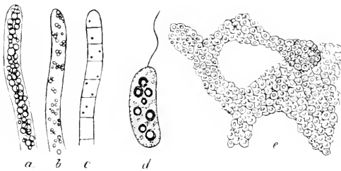
Fig. 17. Schwefelbakterien. a—c Beggiatoa , derselbe Faden, a dick mit Schwefel (schwarzen Ringen) vollgestopft, b teilweise entschwefelt durch 24stündiges Liegen in Brunnenwasser, c Fast ganz schwefelfrei nach weiteren 24—48 Stunden in schwefelwasserstofffreiem Wasser, d Chromatium Okenii , schmutzig-rosae Purpurschwefelbakterie, e Stück einer durchlöchernten Zoogloea von Lamprocystis roseo-persicina . Vergr. a—c 1000, d 900, e , 500; a—c nach Winoogradski, d , e nach Zopf.
