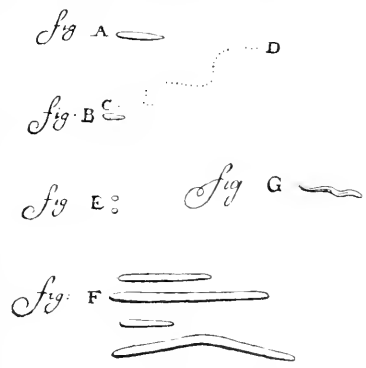
Fig. 1. Älteste Abbildung echter Bakterien (Mundbakterien) nach Leeuwenhoek . A u. F gehören zu dem heutigen Bacillus maximus buccalis , B dürfte ein Vibrio buccalis sein, dessen Bewegung bis D Leeuwenhoek verfolgte. E stellt Kokken dar und G ist wohl ein Spirillum sputigenum . (Man vergl. auch Fig. 26.)
