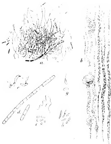
Fig. 26. Bakterien der Mundhöhle und der Zähne. a Bakterienhäuten (nach Miller). b Zahnbeinkanälchen teils mit Kokken, teils mit Stäbchen vollgestopft und erweitert (nach Miller). c Spirillum sputigenum . d Bacillus maxim. buccalis , mit Granulosereaktion. e Kokken. f Spirochaete dentium . g Vibrio buccalis . h Stäbchen, wahrscheinlich Milchsäurebakterien ( Bac. acidi lactici ). Vergr. a circa 250, b 400, c-h circa 1200.
