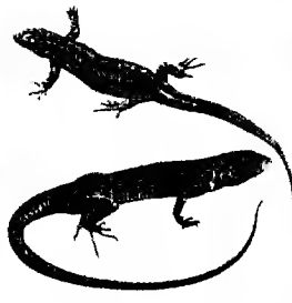
عظاية
