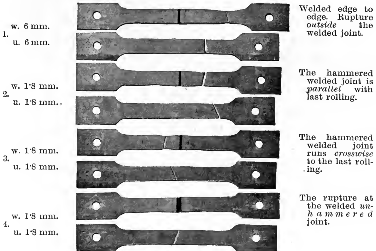
FIG. 19.—Aluminium.
