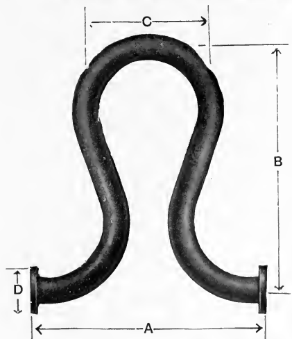
FIG. 74.—“Horseshoe” Type.
