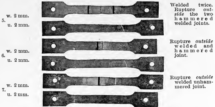
FIG. 20.—Magnalium.
