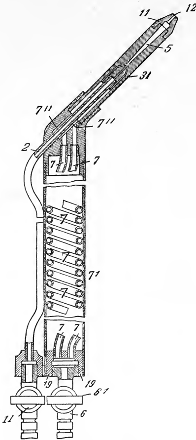
FIG. 85.—Fouché Blowpipe.
