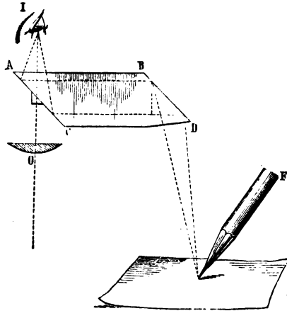
Fig. 56.—Camera Lucida.
