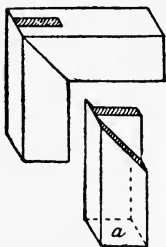
Fig. 74.—Mitre Bridle Joint.
