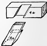
Fig. 33.—Oblique Halving.
