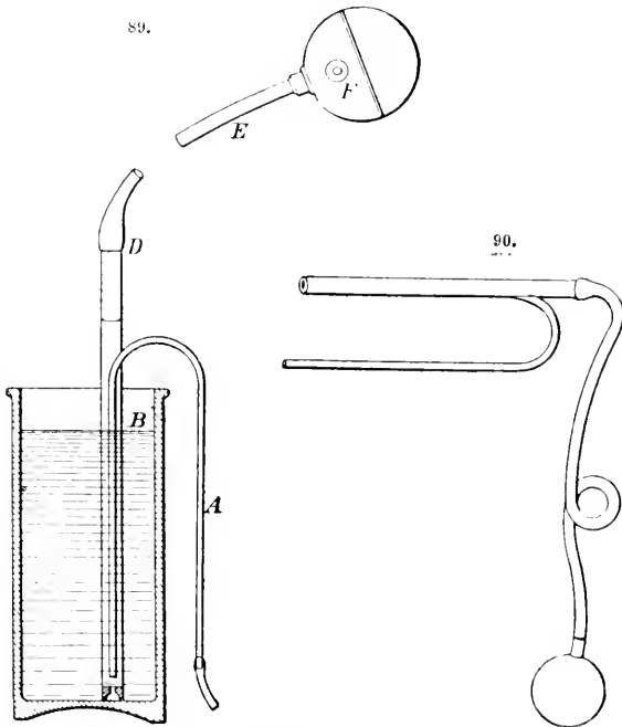
Radiguet's siphon.
