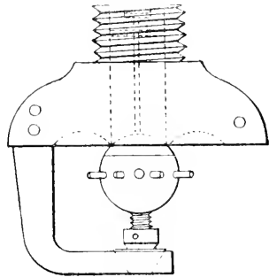
Jolin sprinkler.
