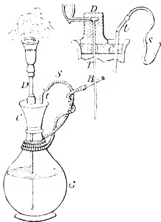
Hookah.
