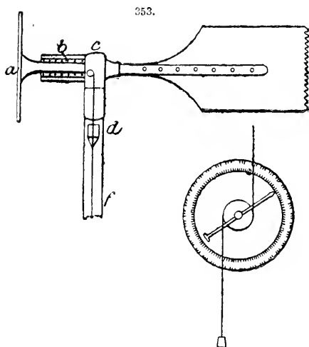
Simple anemometer.
