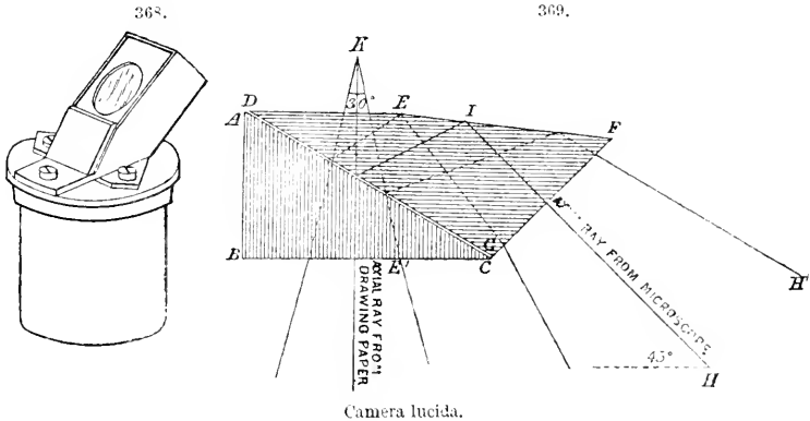
Camera lucida.
