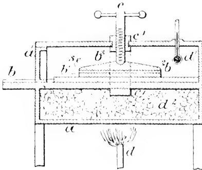
Selenium element.
