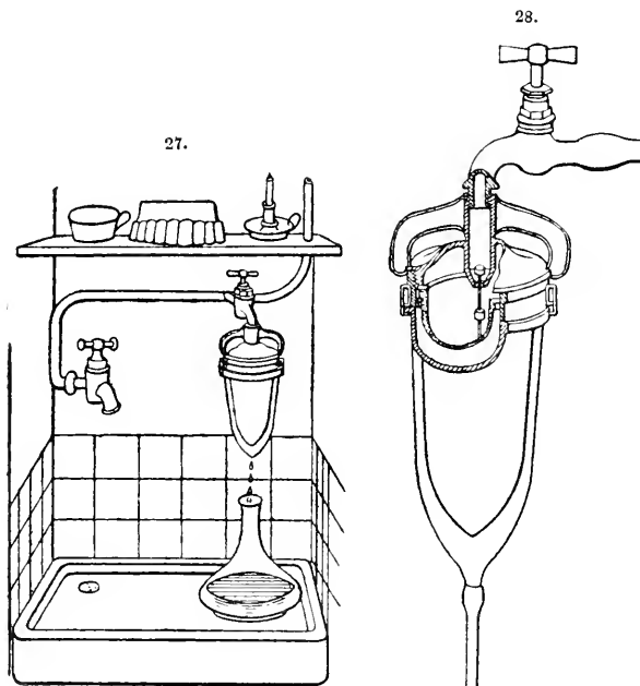
Mallié filter.
