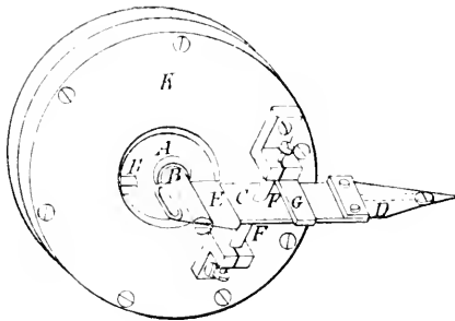
Registering apparatus.
