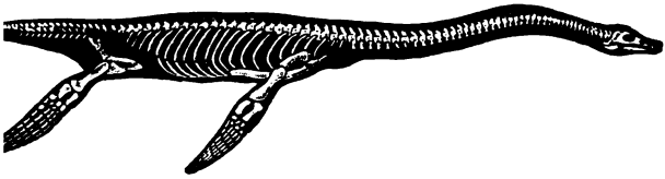
PLESIOSAURUS.
