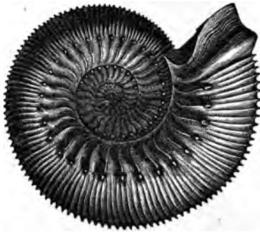
AMMONITES.
