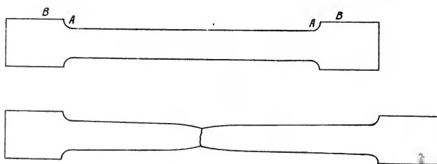
Fig. 1.—Test Pieces.
