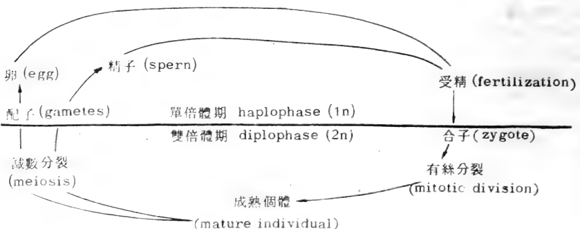
圖 37. 高等動物與某些藻類 (algae) 的雙倍體生活週期 [ 仿自 Cook , 1965 ]。
