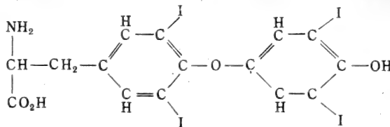
甲狀腺素
