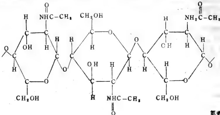
氯氮苯醇
