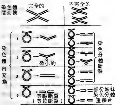
圖 21. 完全和不完全染色體變異之更重要形式的起源，一如在體細胞產生變異的“內交換模式”所解釋。在有絲分裂中期所觀察之變異形式由黑線表示〔仿自 Revell, 1959〕。
