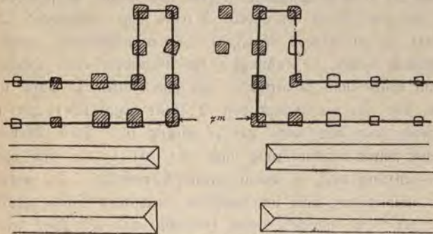
Abb. 5. Thores des großen Lagers in Haltern. 1 : 500
