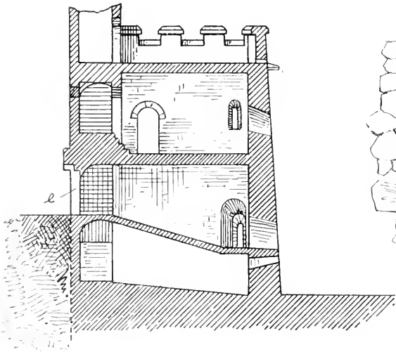
Schnitt B-A
