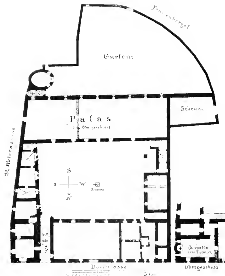
Fig. 1. Der Salzburger Hof. Grundplan von Jahre 1810.
