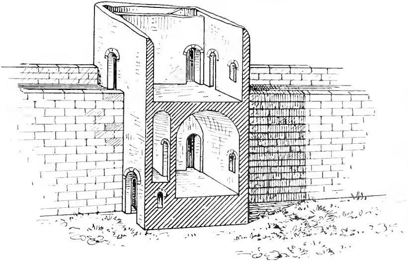
Perspektivischer Schnitt.
