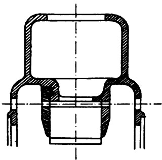
Fig. 9. (Maschine b.)
