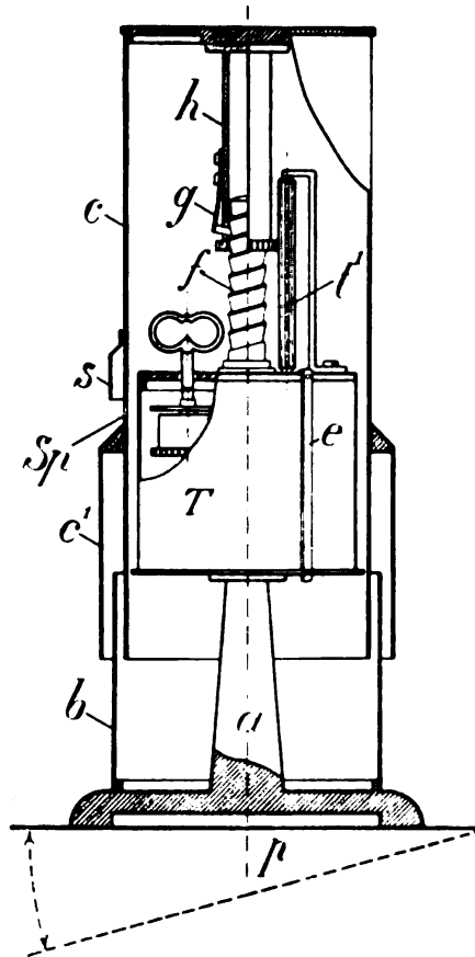
Fig. 1. Apparat zur Lichtmessung.
