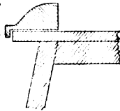
Profil des Plombs mit Halteleiste auf dem Arbeitstisch aufgelegt. Verkleinerung \frac{1}{10} .
