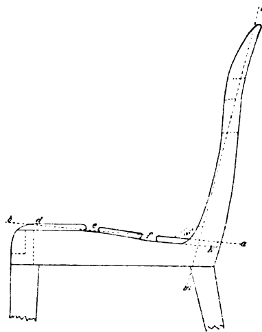
Profil des Stuhls in Verkleinerung auf \frac{1}{15} . a b Totalneigung. l m Profillinie der Lehnenmitte. Uebrigbe Bezeichnungen s. im Text.
