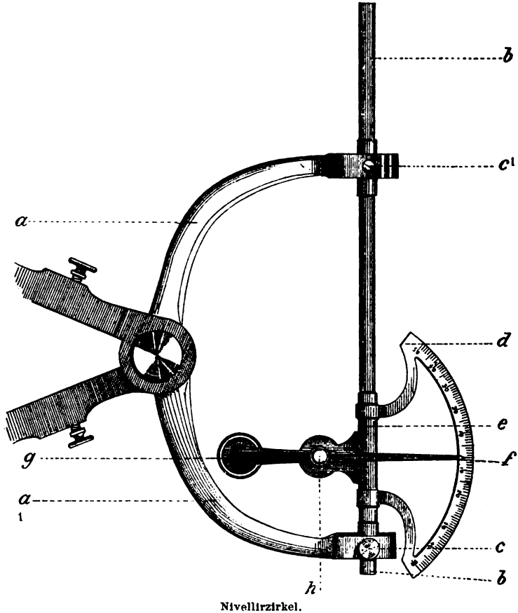
Nivellirzirkel.
