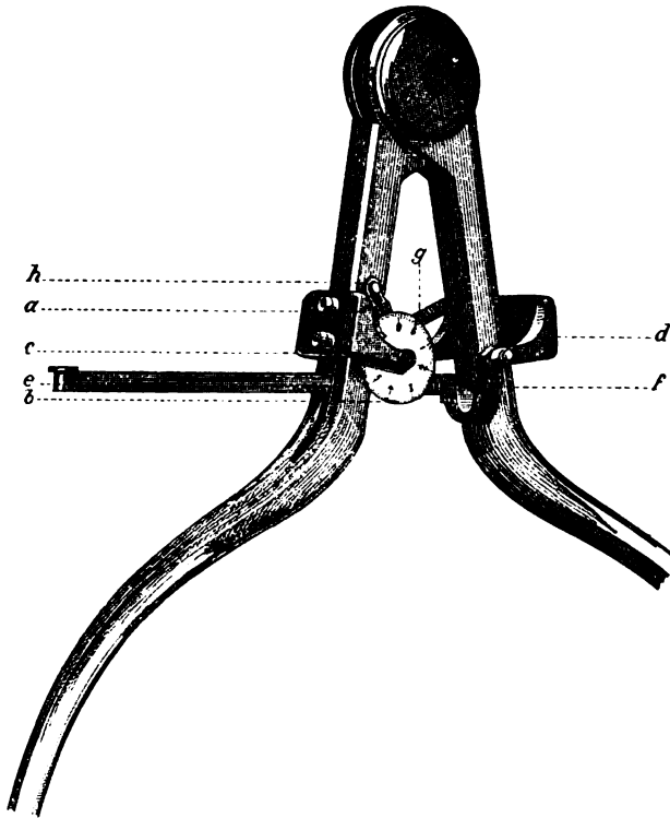
Verbesserter Tasterzirkel.
