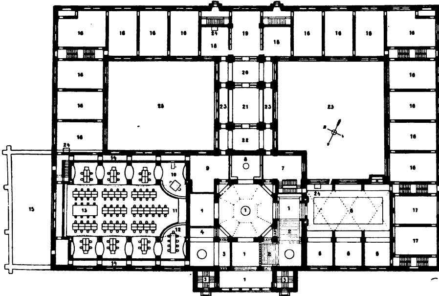
Königliche Bibliothek in Kopenhagen. Abb. 2. Hauptgeschoss.
