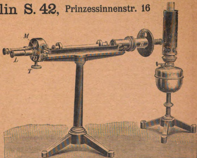
Halbschatten-Polarisationsapparat neuester Konstruktion zur Harnanalyse.
