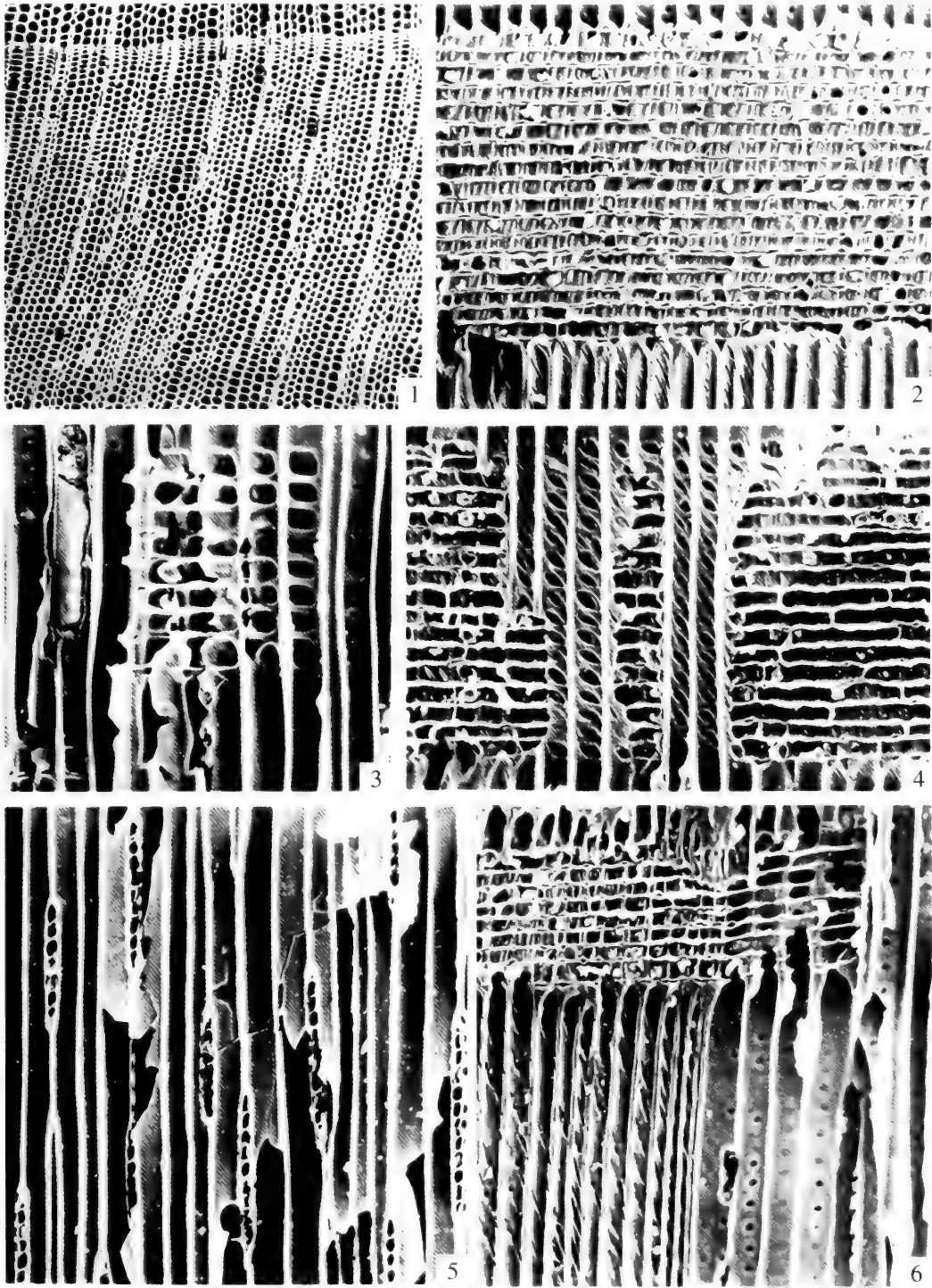
1 横切面, 示生长轮 \times 36 ; 2 径切面, 示射线内壁 \times 190 ; 3 径切面, 示管胞 \times 210 ; 4 径切面, 示交叉场 \times 140 ; 5 弦切面, 示射线 \times 150 ; 6 径切面, 示管胞径壁纹孔和交叉场 \times 160
