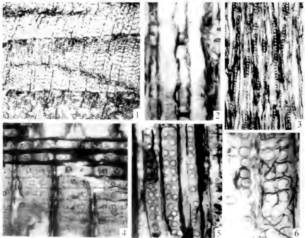
1 径切面，示生长轮 × 25；2 径切面，示轴向薄壁细胞 × 150；3 弦切面，示射线及管胞弦向壁纹孔 × 40；4 径切面，示交叉场纹孔 × 250；5 径切面，示管胞径壁纹孔及眉条 × 170；6 径切面，示管胞内的菌丝 × 350
