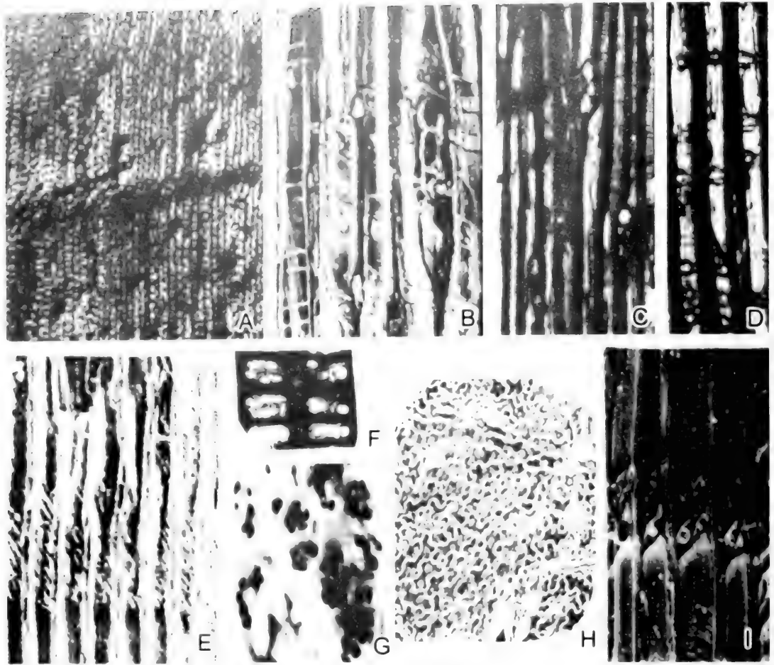
A. 横切面, \times 68 ; B. 弦切面, 示管胞壁上的螺旋, 扫描电镜照片, \times 460 ; C. 弦向面, \times 162 ; D. 径向面, \times 220 ; E. 径向面中部排列整体的纹孔为交叉场纹孔, \times 330 , 扫描电镜照片; F. 示交叉场的具缘纹孔, \times 240 ; G. 筛域的扫描电镜照片, \times 3200 ; H. 树干表皮角质层的扫描电镜照片; I. 径切面管胞外壁及交叉场, 扫描电镜照片, \times 400
