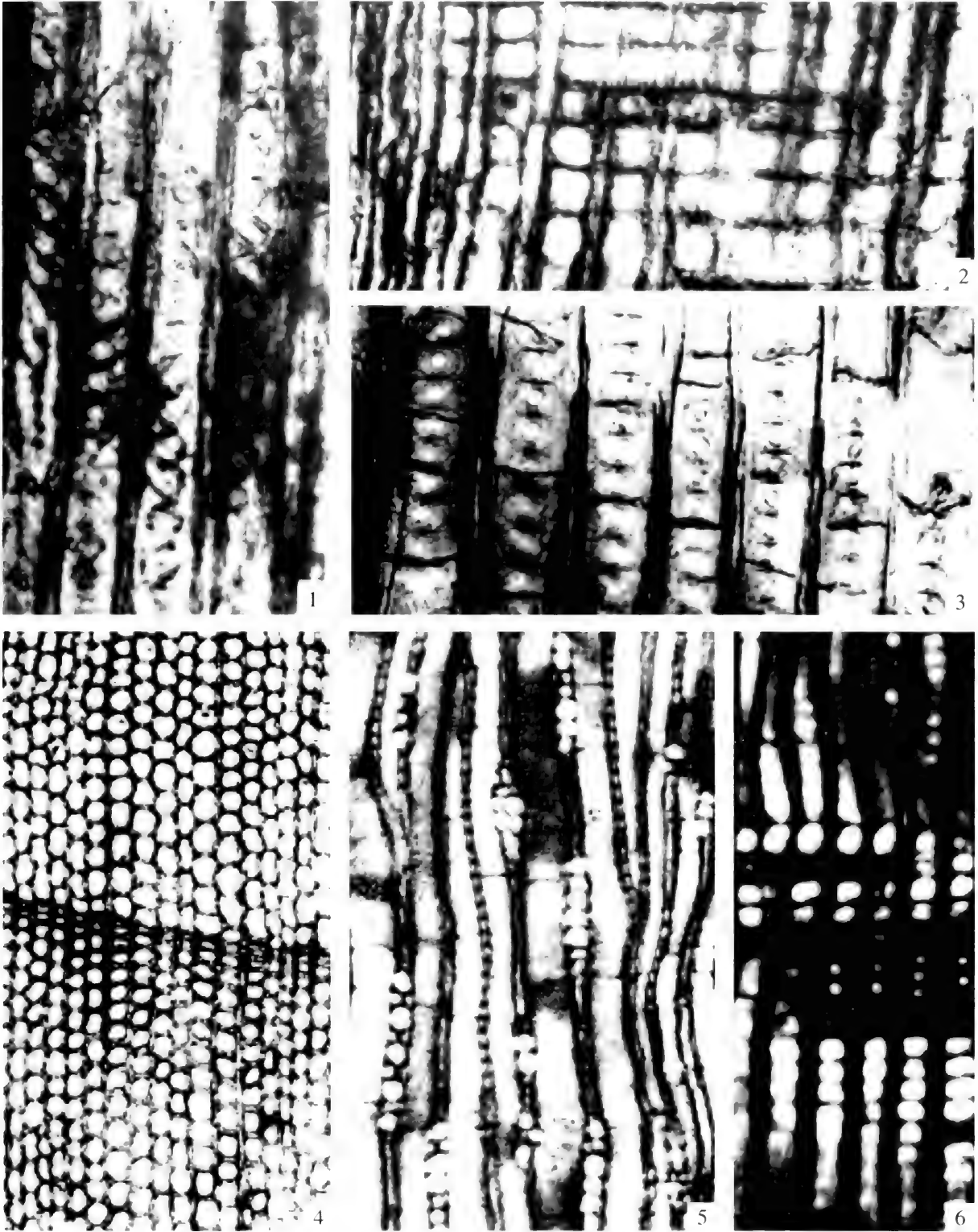
图版6-28 金刚山原始罗汉松型木 Protopodocarpoxyton jingangshanense Ding 及 弗兰肯原始叶枝杉型木 Protophyllocladoxylon franconicum Vogellehner (引自丁秋红, 2000)
