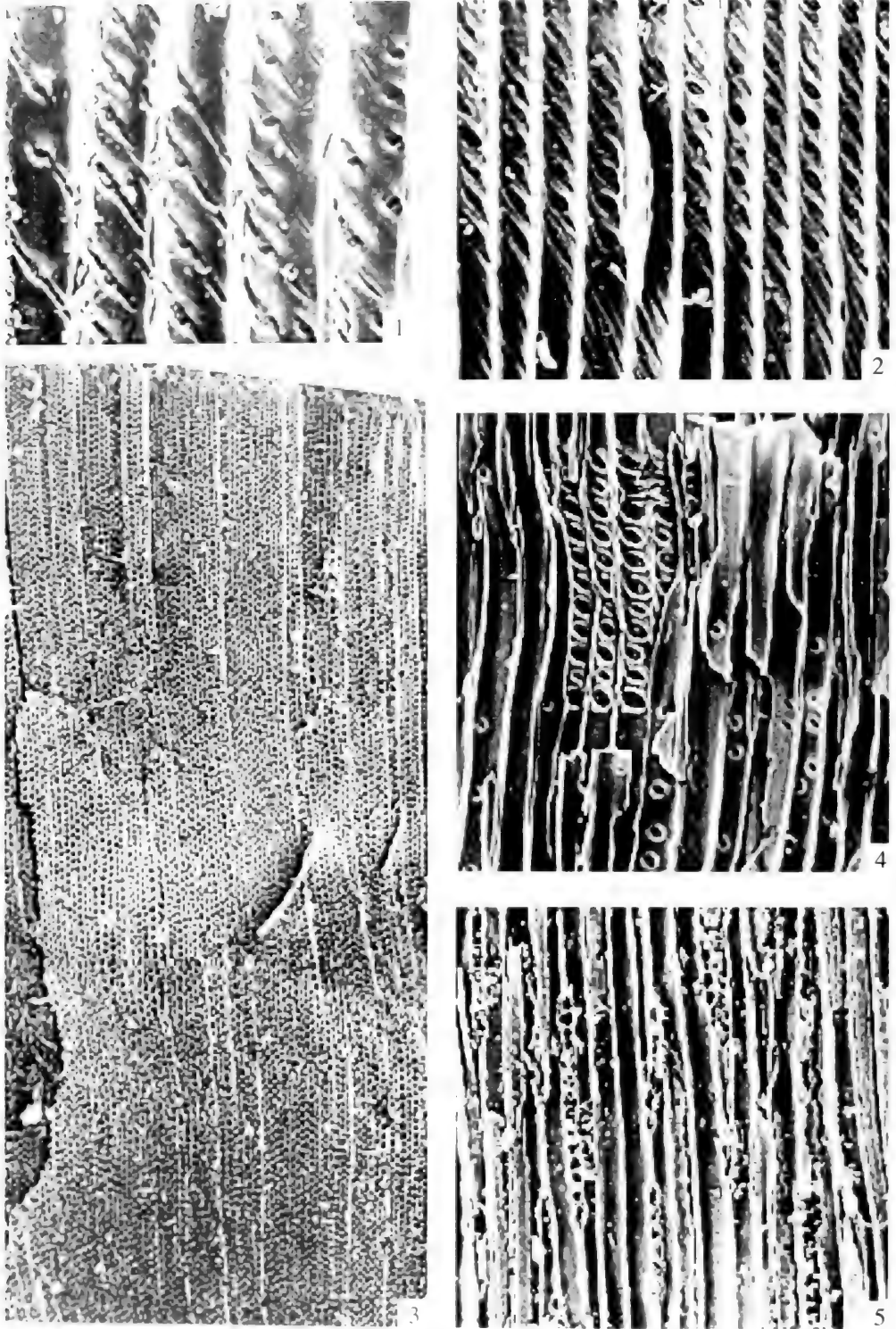
1 弦切面, 示射线和带纹导管 \times 325 ; 2 径切面, 示交叉场纹孔 \times 255 ; 3 横切面, 示生长轮 \times 235 ; 4 径切面, 示射线和带纹导管 \times 235 ; 5 弦切面, 示射线 \times 130
