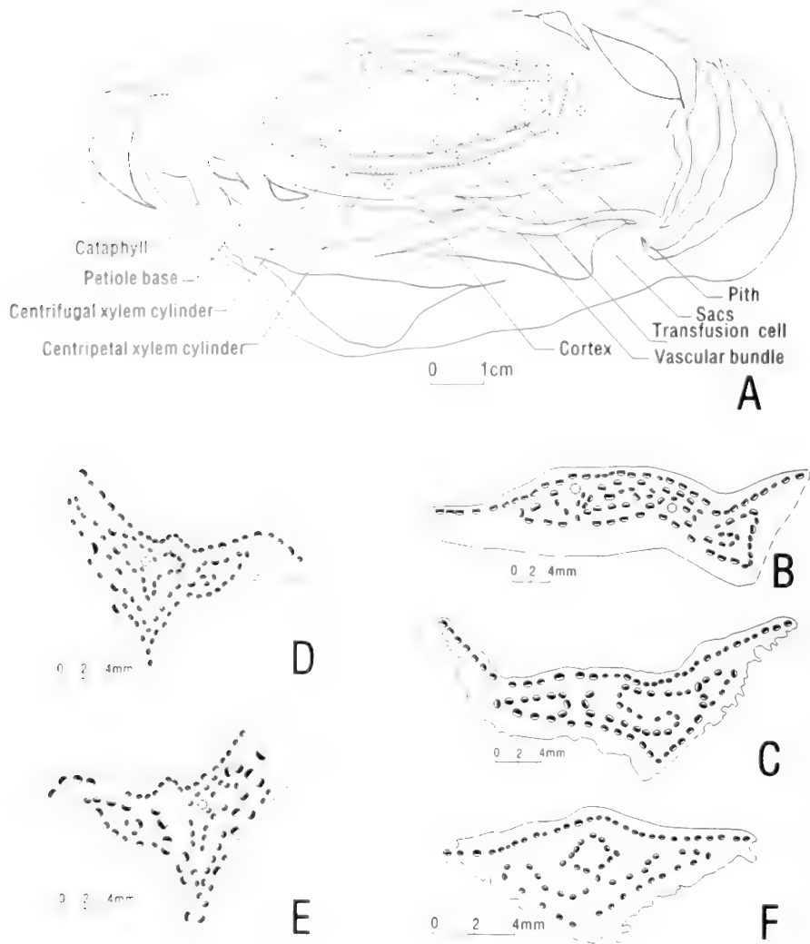
A. 茎干横切面示意图，示髓，两个木质部轮，皮层，叶柄基和鳞片基，髓射线束，粘液腔及运输细胞； B-E. 叶柄基的横切面图，示维管束的分布情况 注：维管束的黑色和白色部分分别代表初生和次生木质部； F. 鳞片基的横切面，示两轮维管束 注：在图B-F中，维管束有两种系列：一列排列沿着近轴缘排列为单个的弧曲形，另一列排列为在叶基部不甚发育的Omega型或者不规则型。
