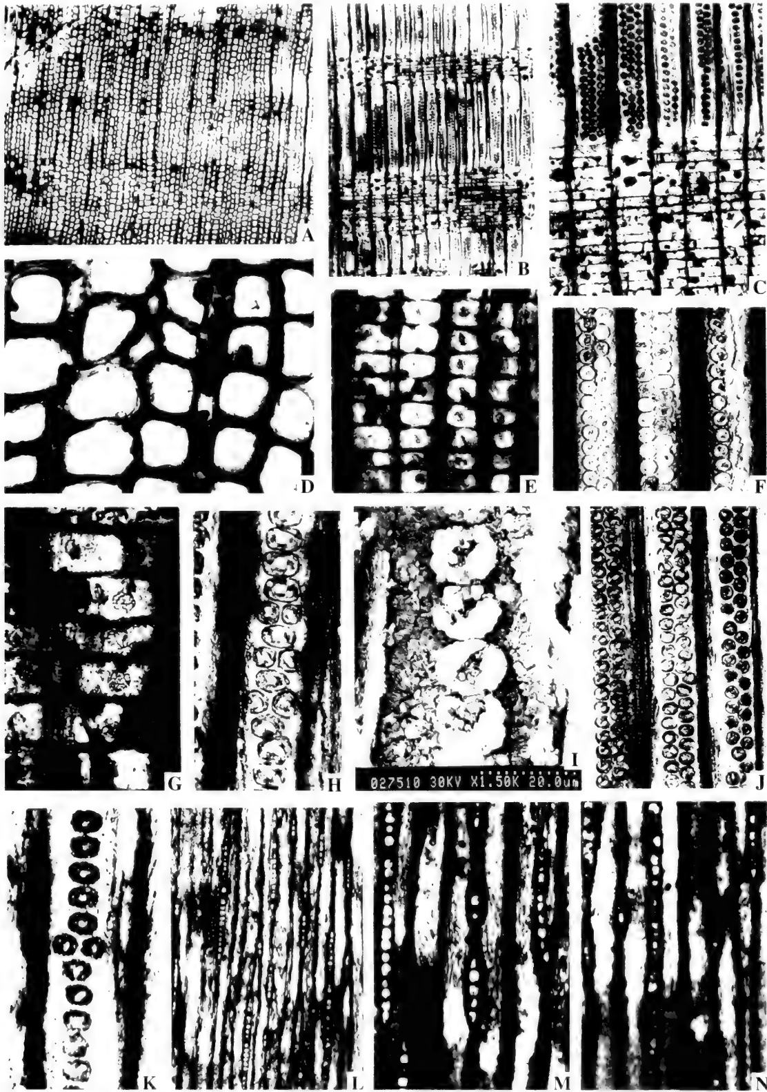
A, D. 横切面, 示管胞形态轮廓, A×20, D×200; B-C, E, G. 径切面, 示在每个交叉场中为一个柏木型纹孔, B×36, C×90, E, G, ×360; F, J. 径切面, 示径向壁两列互生纹孔, ×180; H, K. 径切面, 示径向壁在单列分离或接触纹孔中有双列对生纹孔, ×360; I. 径切面, 示管胞径壁单列具缘纹孔; L-N. 弦切面, 示单列、局部双列射线和管胞的弦向壁具孔, L×45, M, N, ×90
