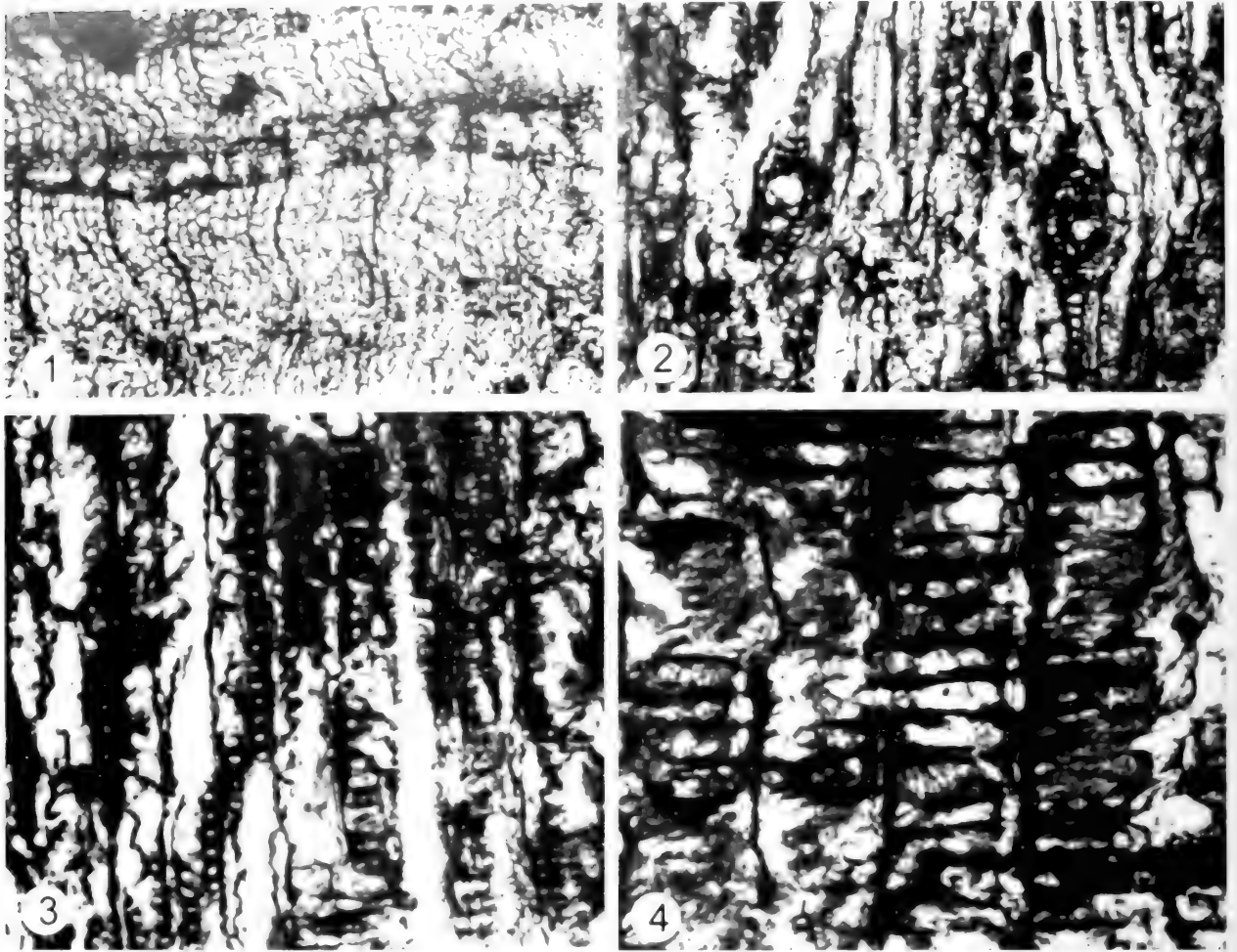
1 横切面, 示生长轮明显, 创伤树脂道丰富, \times 100 ; 2 弦切面, 示射线形态, \times 240 ; 3 径切面, 示管胞壁纹孔, \times 400 ; 4 径切面, 示交叉场纹孔, \times 480
