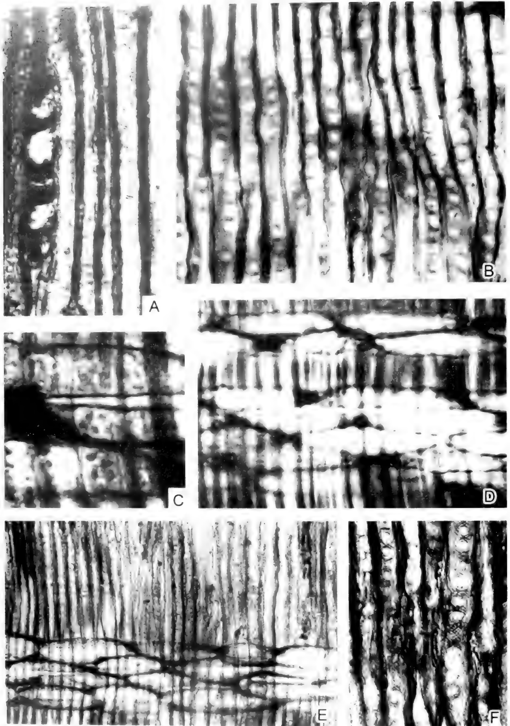
图 3 1. 管胞形态及弦向管胞壁上的具缘纹孔, \times 350 ; B, F. 径切面, 示管胞径壁纹孔式, \times 350 ; C. 横切面, 示具缘纹孔, \times 700 ; D. 横切面, 交叉场木射线形态、交叉场纹孔和细胞两端暗色树脂沉积物, \times 700 ; E. 径切面, 示交叉场木射线细胞形态及纹孔的斜列方式, \times 200
