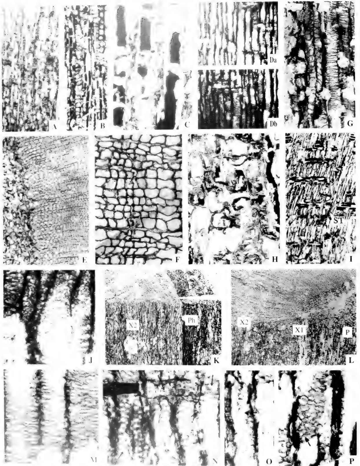
A. \times 20 , B. \times 50 , C. \times 200 ; Da, Db. 径切面, 示次生木质部同一管胞的管胞壁加厚; E. 横切面, 示次生木质部与髓之交界, \times 50 ; F. 横切面, 示次生木质部与髓之交界, 原生木质部的环纹管胞、螺纹管胞
