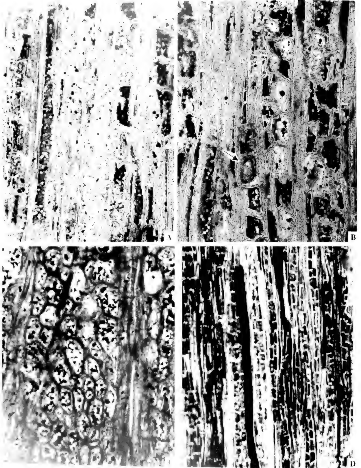
图 69: B 示射线细胞 1—3 列, 具孔, 个别的 C 示射线细胞, 示很高的多列木射线和长方形—多 列木射线 (模式图存于沈阳地质矿产研究所)
