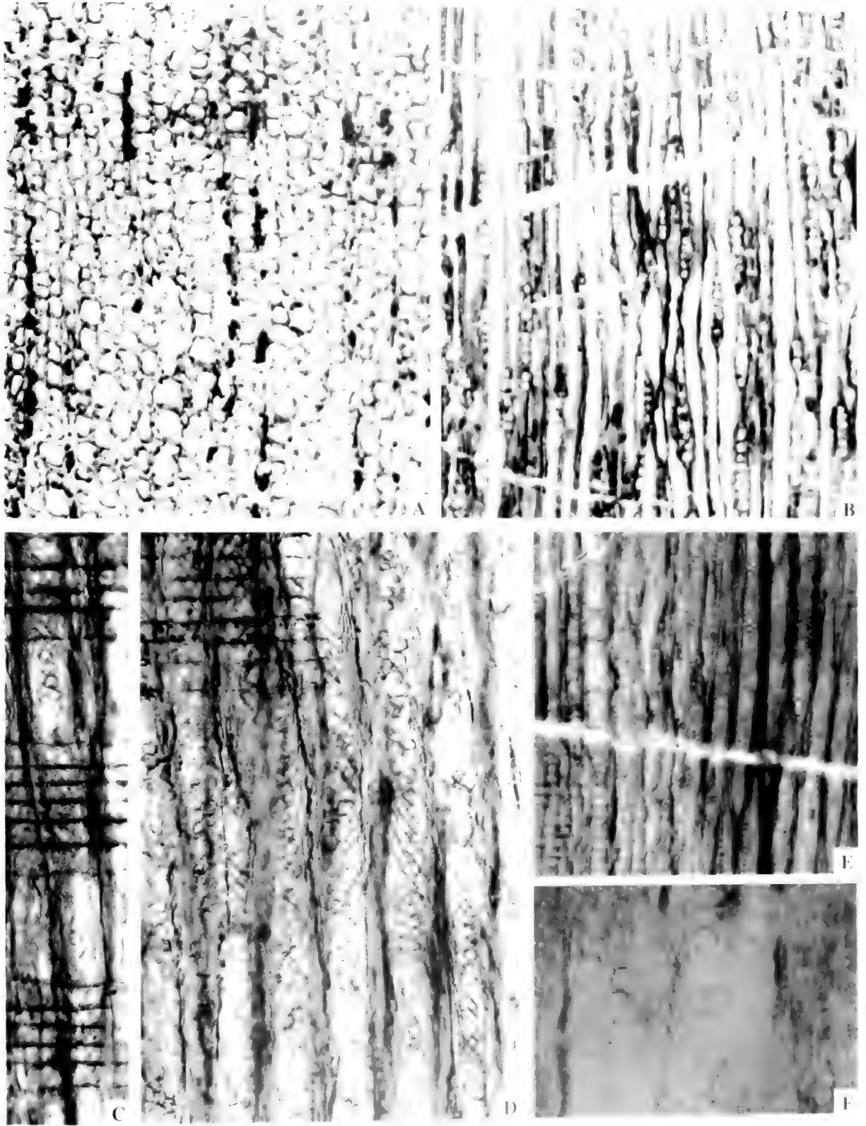
A. 横切面, 示管胞形态轮廓及不整齐的孔, \times 66 ; B. 弦切面, 示平孔, 与管胞孔不连续, \times 165 ; C. 径切面, C. 示管胞径向壁单列纹孔; D. 示管胞径向壁单列纹孔及交叉的螺旋纹孔, \times 165 ; E. 示轴向木薄壁组织, \times 71 ; F. 示管胞弦切面, 示平孔及管胞孔不连续, \times 329 ; 标本号: GJ6-22 (标本与薄片保存在北京)
