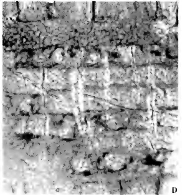
图 1. A. 射线, \times 70 ; C-D. 径切面, D. \times 350
