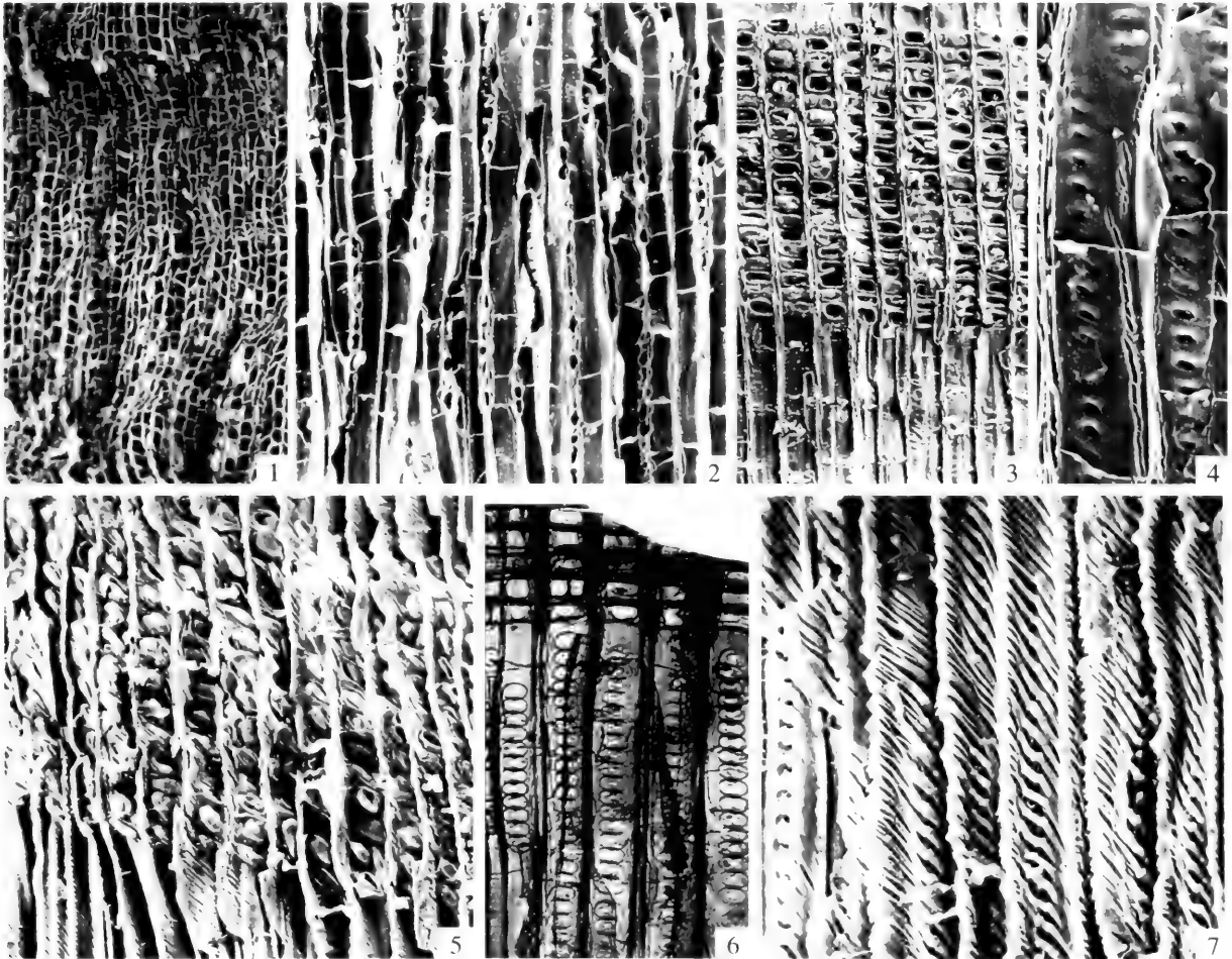
1 横切面, 示生长轮不明显 \times 67 ; 2 弦切面, 示木射线 \times 120 ; 3, 5 径切面, 示交叉场纹孔 \times 312, \times 310 ; 4, 6 径切面, 示管胞径壁纹孔 \times 312, \times 138 ; 7 径切面, 示管胞壁条纹增厚和紧挤的纹孔 \times 310
