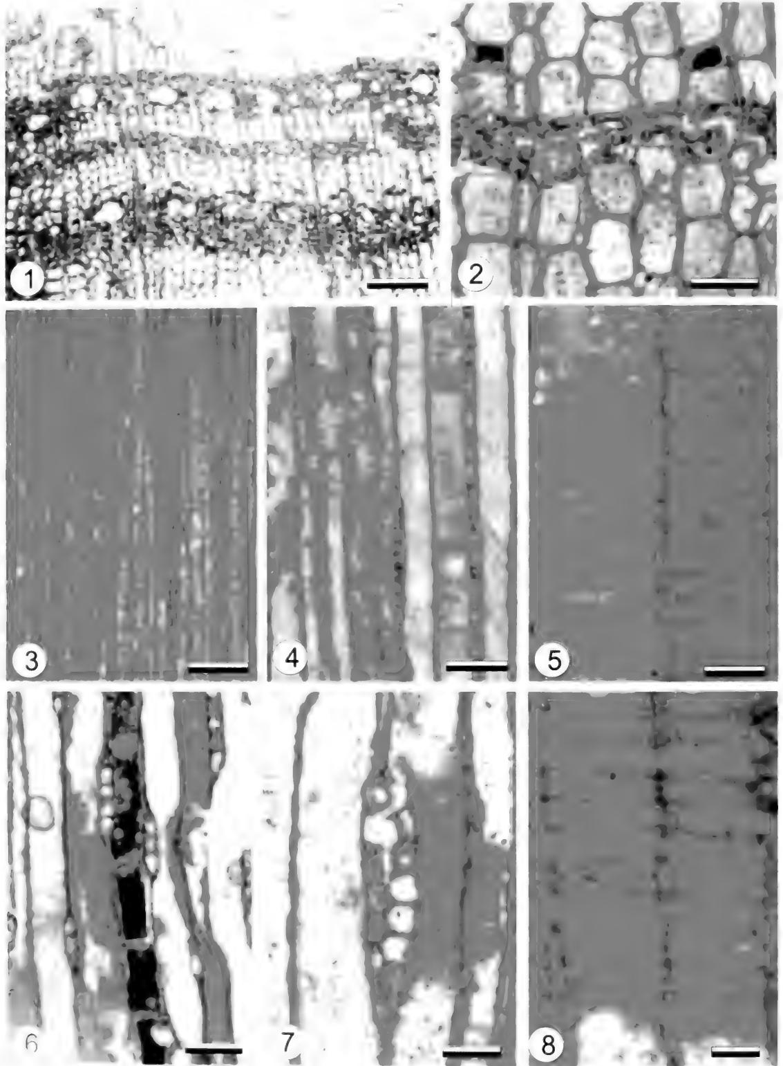
1 茎纵切面，创伤树脂道，标尺0.4 mm；2 横切面，示晚材带窄，星散状轴向薄壁组织细胞，标尺0.4 mm；3 纵切面，示射线高度，标尺代表0.4 mm；4 弦切面，示射线细胞形态，标尺代表200 μm；5 纵切面，示轴向薄壁组织壁细胞端壁平滑，标尺100 μm；6 弦切面，示轴向薄壁组织壁细胞端壁平滑，标尺100 μm；7 纵切面，示缘纹孔，标尺50 μm；8 径切面，示交叉场纹孔柏木型，标尺50 μm
