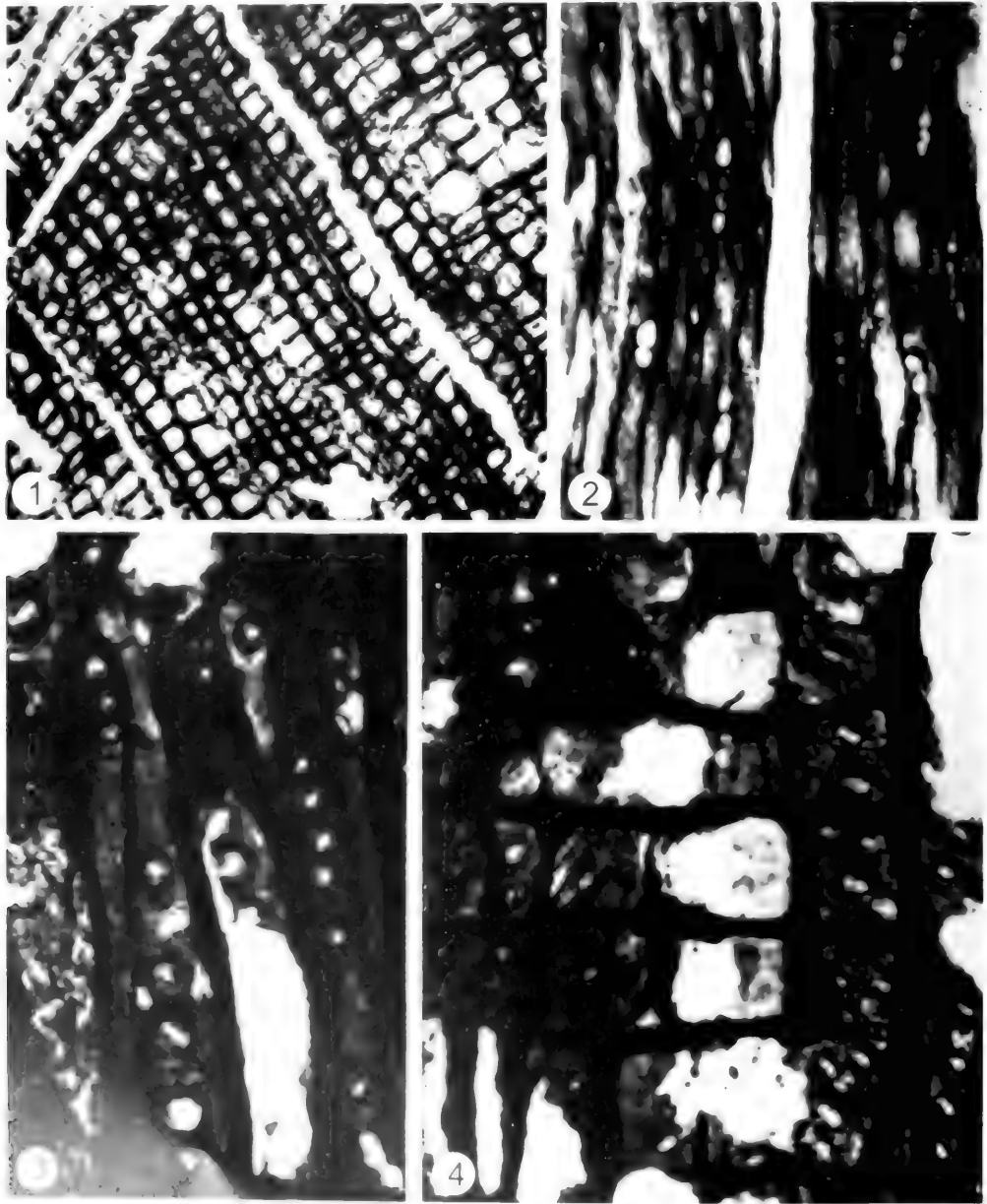
1 材切面， \times 180 ；2 弦切面，示射线形态， \times 120 ；3 径切面，示管胞 4 径切面， \times 500
