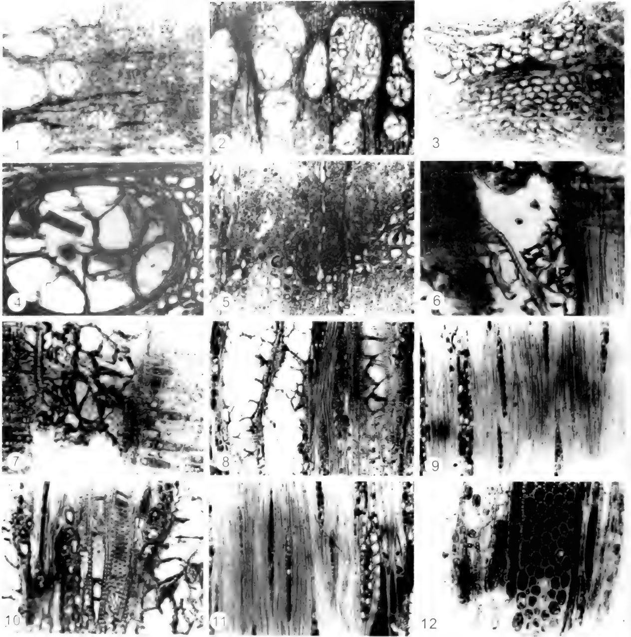
1 横切面, 示生长轮, 呈散材, \times 100 ; 2 横切面, 示环孔材, \times 100 ; 3 横切面, 示管孔弦向薄壁组织, \times 200 ; 4 横切面, 示导管内腔填充体, \times 200 ; 5 横切面, 示波浪环薄壁组织, \times 200 ; 6 弦切面, 示斜向排列的管胞, \times 100 ; 7 径向面, 示导管节及射线, \times 200 ; 8 弦切面, 示倾斜穿孔板, \times 100 ; 9 弦切面, 示单列和多列射线, \times 100 ; 10 弦切面, 示单列和多列射线, \times 100 ; 11 弦切面, 示薄壁细胞上的纹孔, \times 200 ; 12 弦切面, 示宽6列细胞的射线, \times 200
