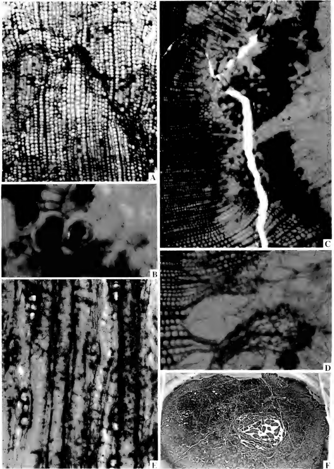
A、D、E 为切向，A 示管胞的形态特征， \times 31 ；B 示管中分泌细胞群， \times 156 ；C 示（右）中薄壁细胞分泌细胞群与木栓层与次生木质部交界， \times 31 ；D 示管边缘的撕裂状破坏， \times 62 ；E 示髓、髓中木栓化射线与次生木质部， \times 14 ；F 为切向，示木射线 1~2 层，射线细胞壁具孔、管胞弦壁具孔和木纤维的排列， \times 156 ；A、E 标本编号：NU-5。
