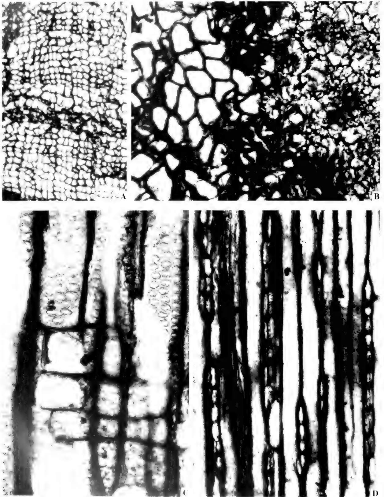
A、B. 横切面，A. 髓部，B. 髓部（右边）和初生木质部（左边）的管胞充满黑色物质， \times 52 ；C. 径切面，示管胞纹孔和交叉场纹孔， \times 350 ；D. 弦切面，示管胞螺旋纹孔， \times 350 。
