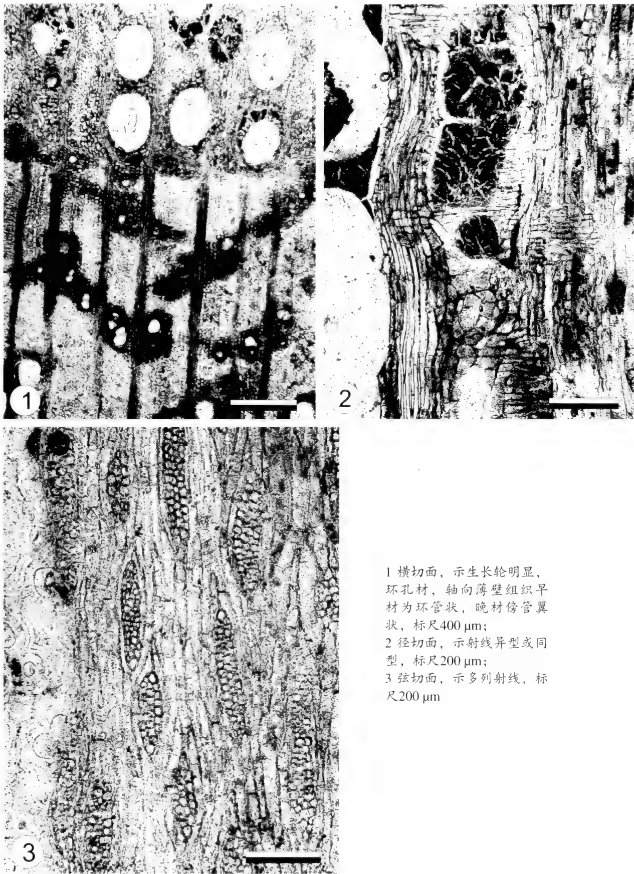
图版7-28 武汉榉木 Zelkova wuhanensis
