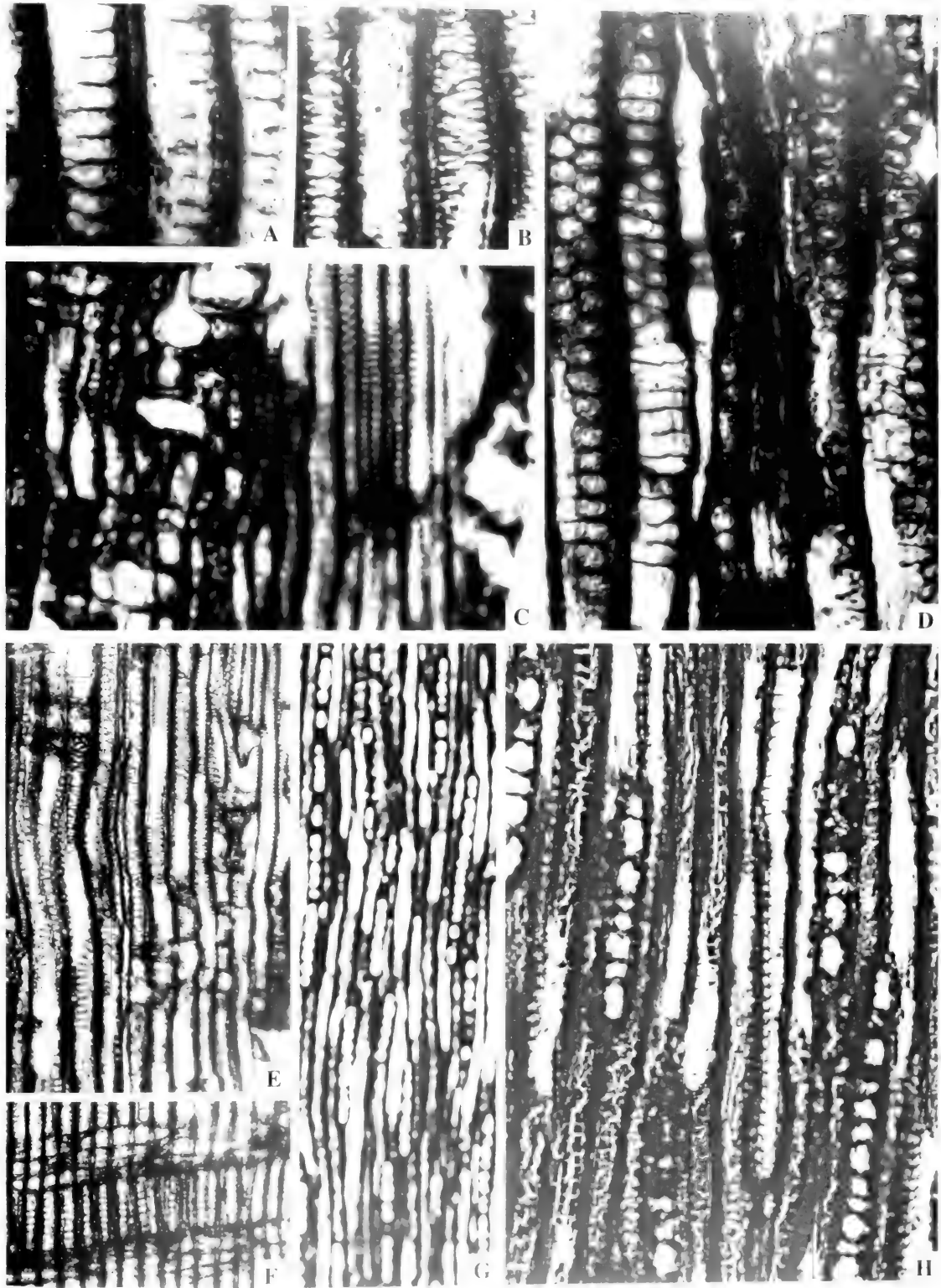
A-F. 径切面, A. 示管胞径向壁厚及螺旋加厚, ×312; 标本编号: NH11; B. 示次生木质部中管胞具网纹加厚, ×312; 标本编号: NH11; C. 生长轮, 左侧为初生木质部, 右侧为次生木质部 (中部) 和次生木质部, 在生长轮处有管胞具螺旋加厚, ×312; 标本编号: NH11; D. E. 示管胞具螺旋加厚, D. E. ×312; F. ×156; 标本编号: NH11; G. H. 示管胞具螺旋加厚和木薄壁, G. H. ×156; 标本编号: NH11。
