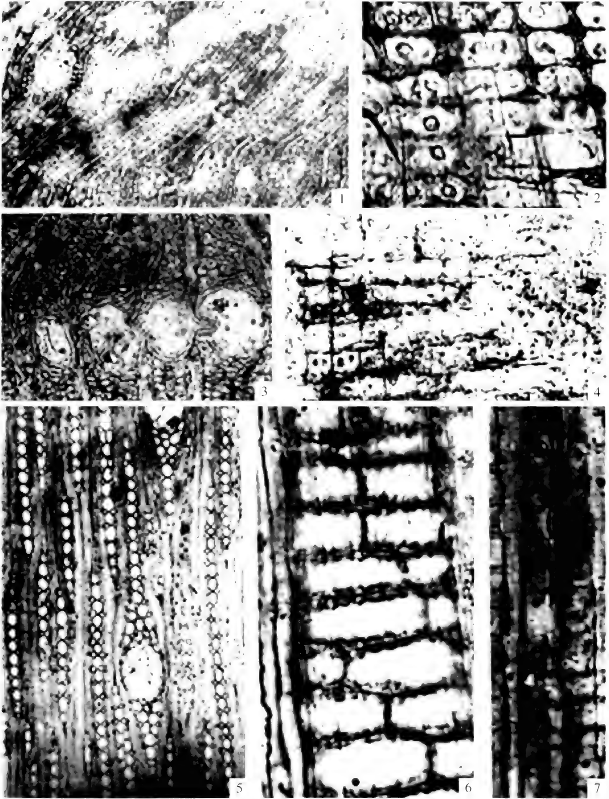
1 横切面, 示生长轮、轴向正常树脂道和创出树脂道 \times 70 ; 2 径切面, 示柏木型交叉场纹孔 \times 350 ; 3 横切面, 示创伤树脂道 \times 175 ; 4 径切面, 示冷杉型交叉场纹孔 \times 350 ; 5 弦切面, 示单列射线和具树脂道的纺锤形射线 \times 70 ; 6 径切面, 示节状加厚 \times 700 ; 7 径切面, 示管胞径壁的具缘纹孔 \times 175
