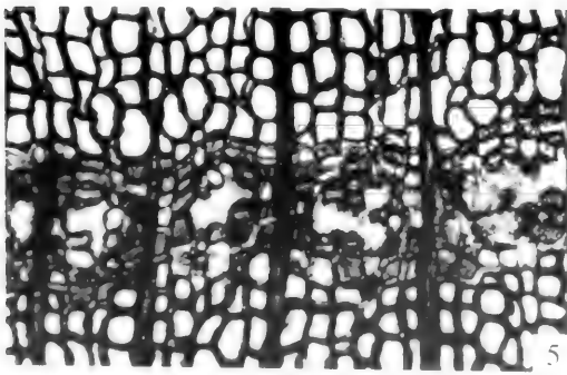
1 纵切面, 示清晰明显的生长轮和假生长轮 \times 5 ; 2 横切面, 示早材到晚材的渐变, 排列整齐的早材管胞 \times 100 ; 3 横切面, 示早材中构成假生长轮的厚壁管胞 \times 100 ; 4 横切面, 示管胞端壁的具缘纹孔 \times 400 ; 5 纵切面, 示管胞的排列 \times 100 ; 6 弦切面, 示单列射线、丰富的轴向薄壁细胞和其中的黑色颗粒状物 \times 100 。
