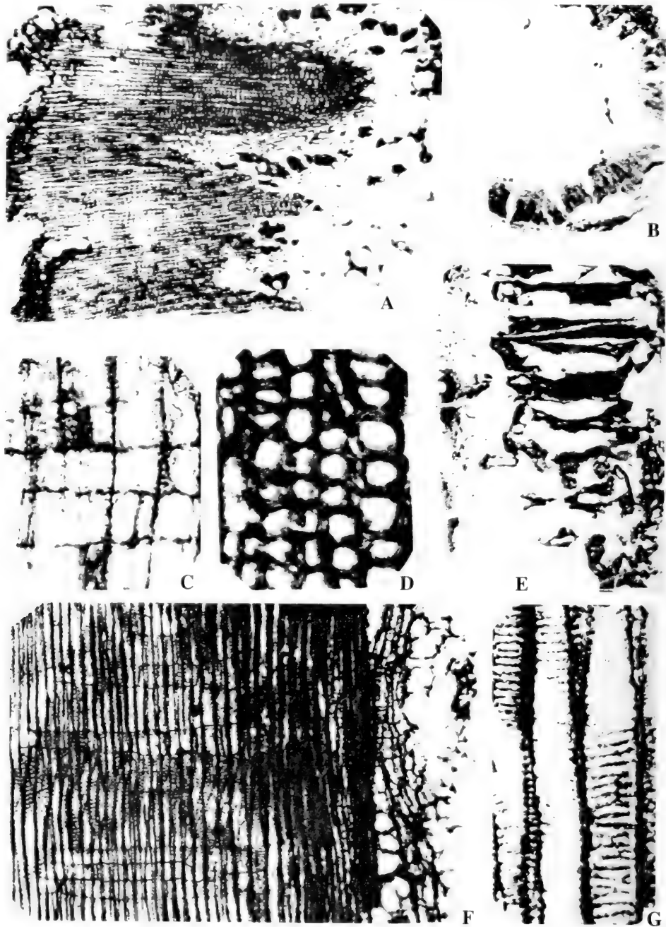
3-11 猴头庙科达木 Cordiaoxylon houtoumiaense (Zhang et Zheng) Wang
