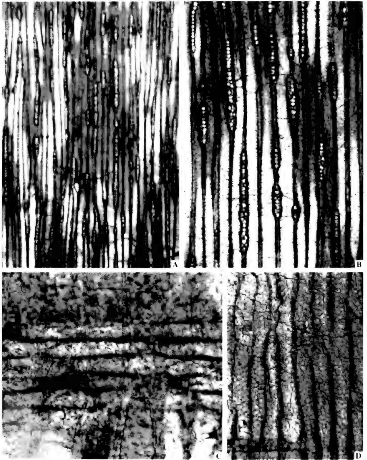
A、B. 弦切面，示管胞壁螺旋加厚1~2列，A×33，B×67；C. 径切面，示交叉场纹孔1~2个，大的、斜或平的简单纹孔，D. 径切面，示管胞晚壁纹孔1~2列，紧挤，圆—多角形，×167。（标本与薄片保存在中国科学院植物研究所）
