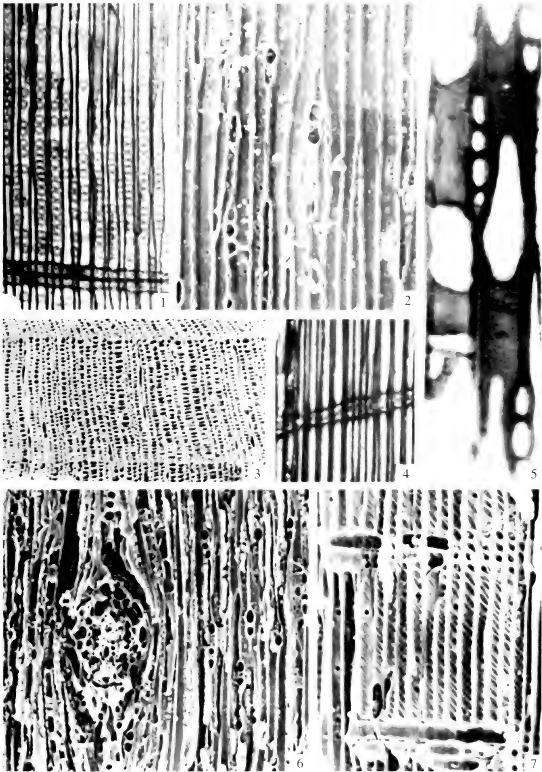
1 径切面, 示管胞径壁纹孔 \times 150 ; 2 弦切面, 示射线 \times 365 ; 3 横切面, 示生长轮 \times 95 ; 4 径切面, 示木薄壁细胞 (左侧) \times 226 ; 5 弦切面, 示木薄壁细胞水平壁节状 \times 380 ; 6 弦切面, 示发达的射线 \times 350 ; 7 径切面, 示径壁纹孔和交叉场 \times 350
