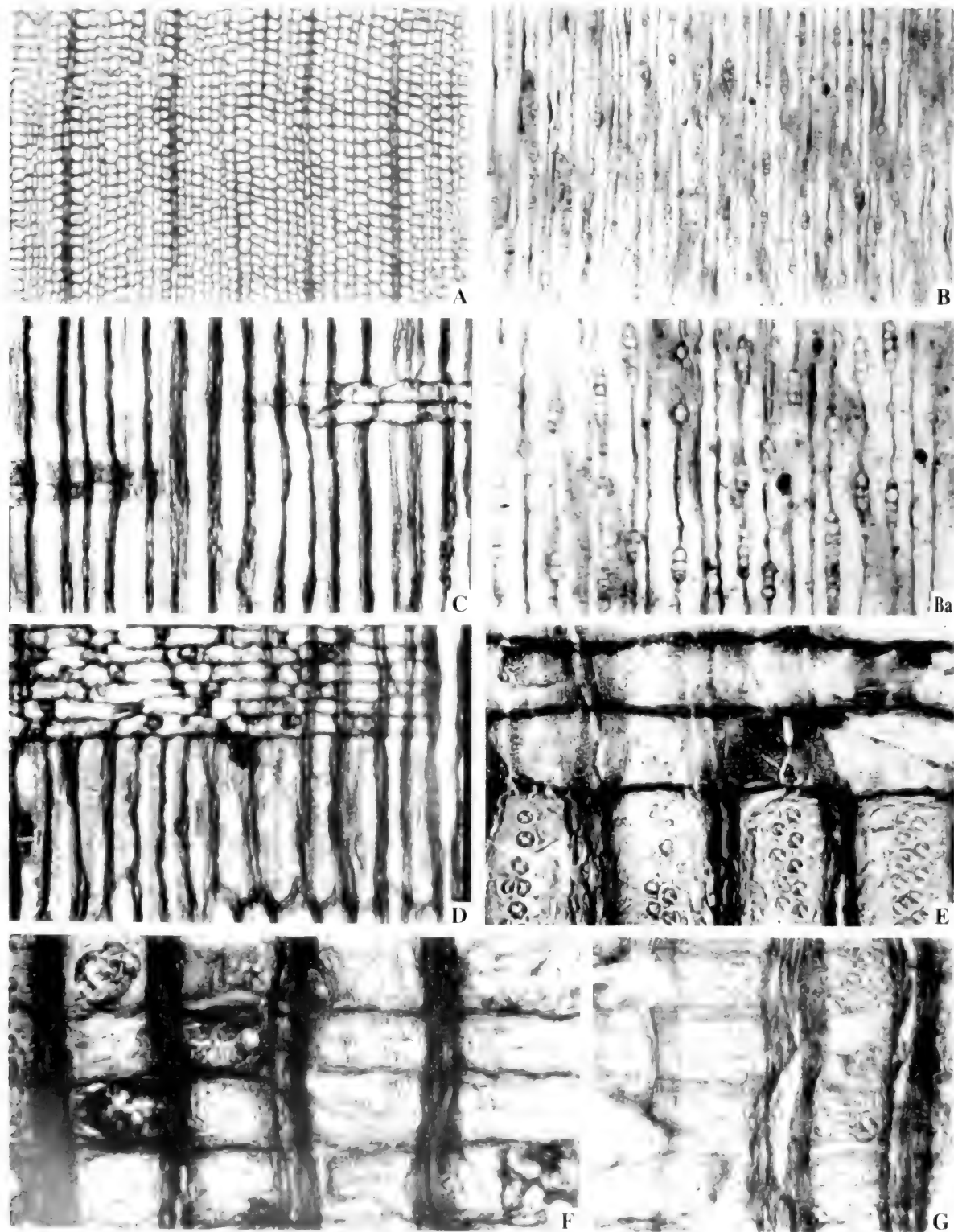
A. 径切面，示管胞和射线， \times 35 ；B. 弦切面，示射线单列、稀局部双列， \times 35 ；Ba为B的部分放大，示射线细胞壁具纹孔， \times 60 ；C-E，径切面，示管胞径向壁具缘纹孔和交叉场纹孔，径向壁纹孔圆形，分列于管胞角隅处，纹孔口针；交叉场纹孔7~11个，偶尔有大的球形体被保存，C-D \times 100 ，E \times 350 ；F-G，弦切面，示交叉场纹孔，在图F左侧有三个球形体， \times 350
