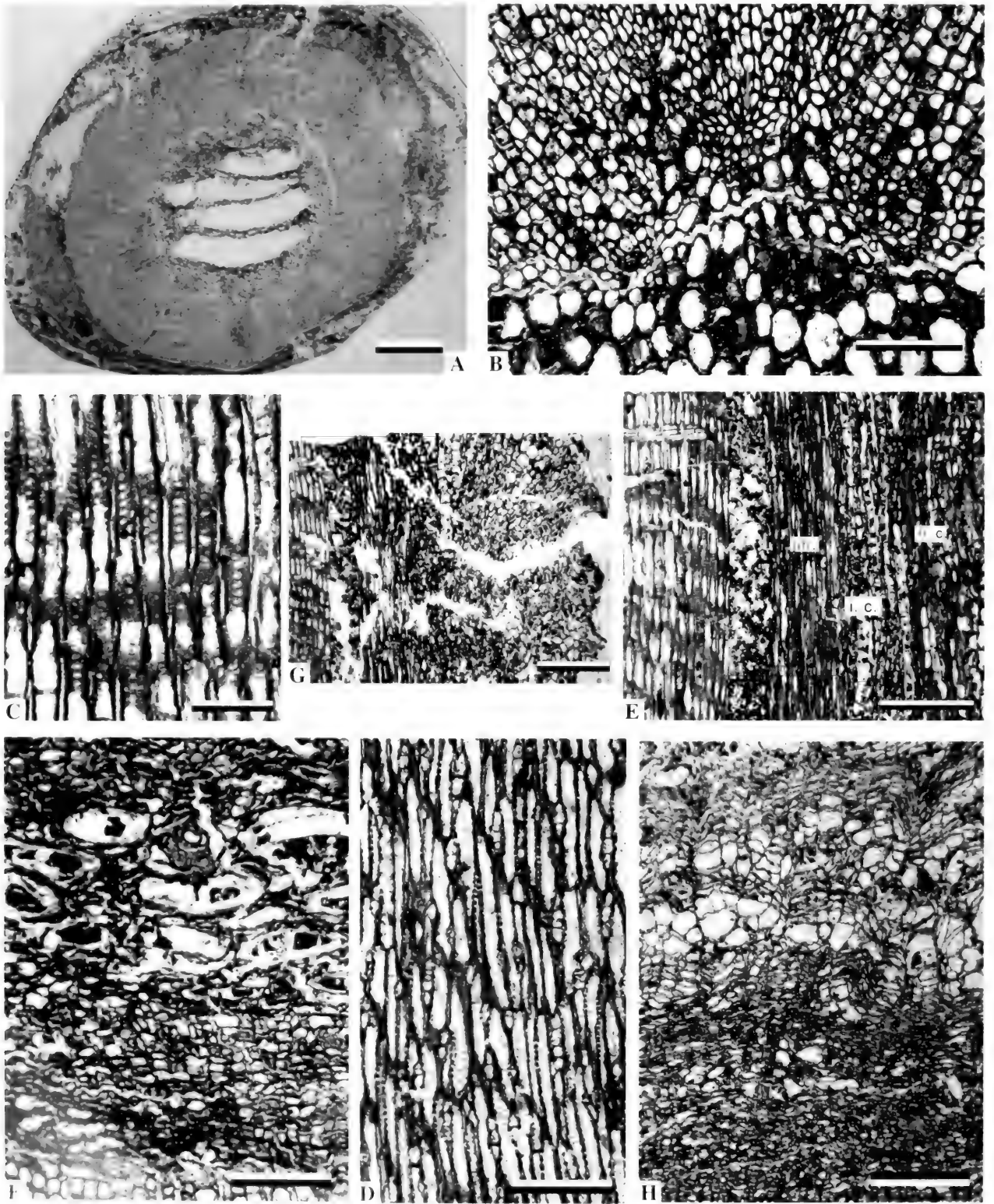
A. 纵切面, 示髓及管胞, 标尺 3 mm; B. 横切面, 示两侧内始式维管束及中间的内始式单叶迹 (箭头所指), 标尺 200 \mu\text{m} ; C. 径切面, 示管胞壁上所具双列互生具缘纹孔, 纹孔口斜卵形, 标尺 100 \mu\text{m} ; D. 径切面, 示次生木部内射线情况, 标尺 200 \mu\text{m} ; E. 纵切面, ph 韧皮部, ic 内皮层, oc 外皮层, 标尺 400 \mu\text{m} ; F. 横切面, 示各部分组织构造, 标尺 200 \mu\text{m} ; G. 径切面, 示皮孔, 标尺 400 \mu\text{m} ; H. 横切面, 示周皮构造, 标尺 400 \mu\text{m}
