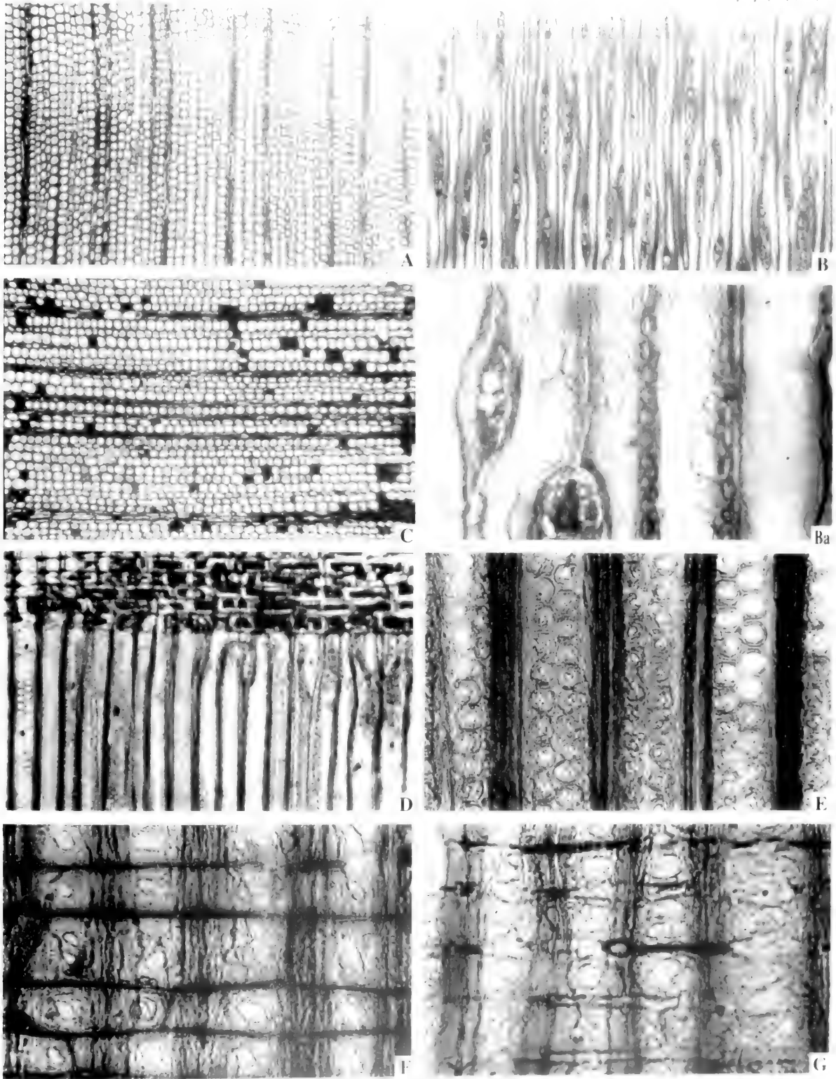
A. 横切面，示直径缩小的一个带，像假轮， \times 35 ；B. 同一标本的横切面，示生长轮缺失， \times 35 ；C. 弦切面，示单列的和局部双列的木射线， \times 35 ；D. 为B的局部放大，示弦向壁偶尔出现具缘纹孔， \times 350 ；E. 径切面，示木射线的一部分为双列，射线细胞中充满黑色物质， \times 100 ；F. 径切面，示径切壁，具圆形-亚圆形，2列互生，孔口钝， \times 350 ；G. H. 径切面，示每个交叉处均有纹孔1个，稀2个，呈卵圆形，简单， \times 350
