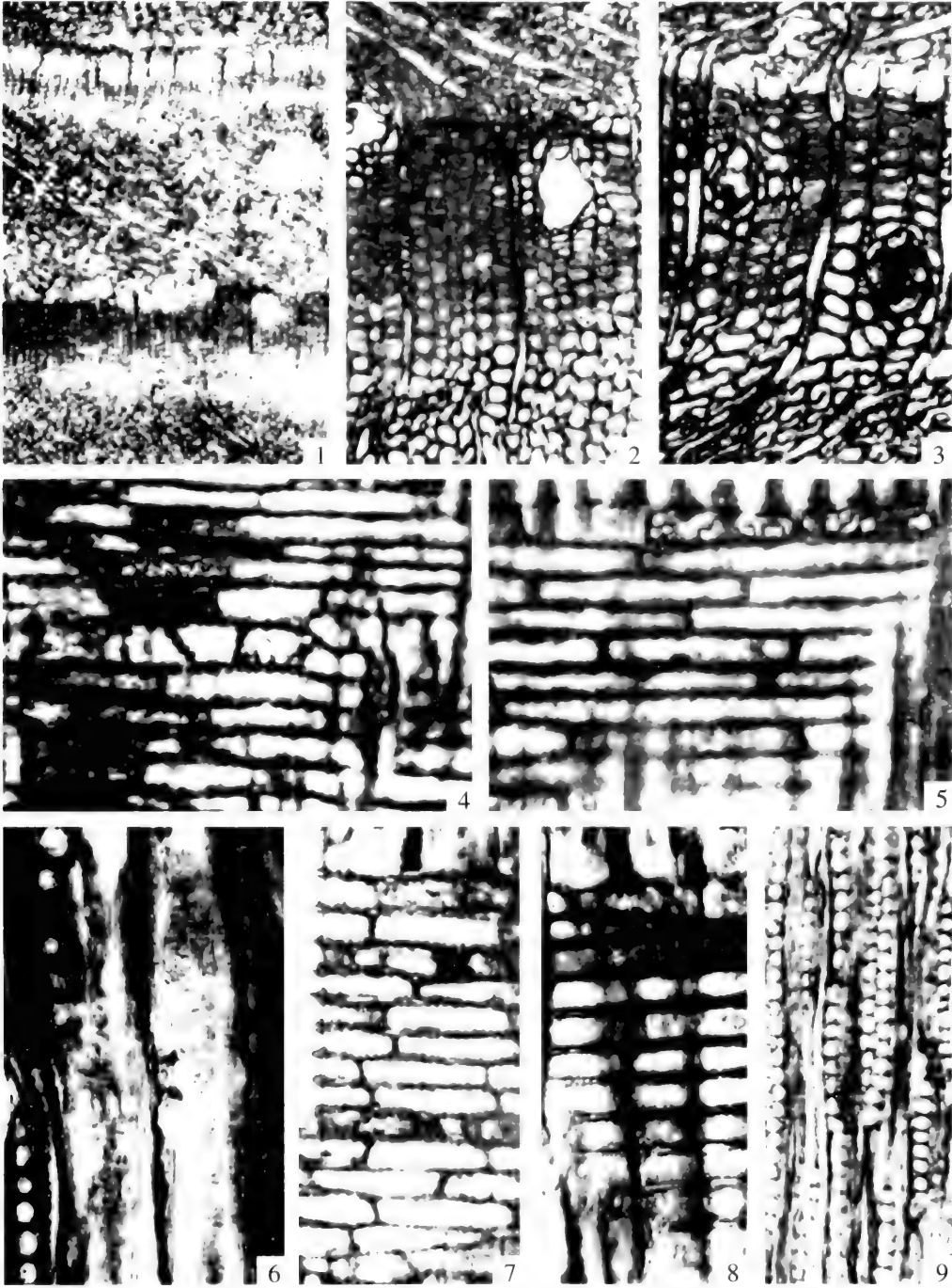
1 横切面, 示生长轮、轴向创伤树脂道和正常树脂道 \times 30 ; 2 横切面, 示管胞和正常轴向树脂道 \times 90 ; 3 横切面, 示轴向树脂道及侵填体 \times 90 ; 4 径切面, 示射线细胞弦壁节状加厚 \times 180 ; 5 径切面, 示射线细胞内的晶状充填物 \times 180 ; 6 径切面, 示管胞径壁纹孔及眉条 \times 360 ; 7 径切面, 示射线细胞横壁纹孔和边缘细胞外壁波浪形 \times 180 ; 8 径切面, 示交叉场纹孔 \times 180 ; 9 弦切面, 示木射线 \times 90
