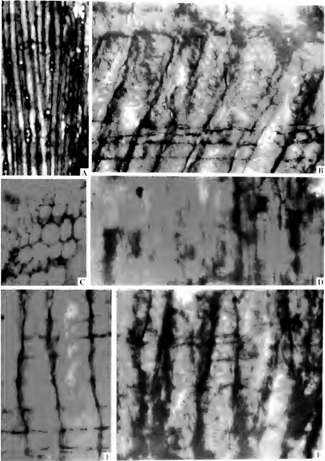
A. 弦切面，示单列射线， \times 63 ；B. 径切面，示1~3列径壁纹孔和射线细胞水平壁具孔， \times 315 ；C. 横切面，示初生木质部管胞（左上）和次生木质部管胞（右部）的梯状加厚， \times 158 ；D. 径切面，示初生木质部管胞（右）具梯状加厚和其中纵向生长纹孔， \times 158 ；E. 径切面，示次生射线细胞和射线细胞水平壁具孔， \times 315 ；F. 横切面，示射线， \times 158 。
