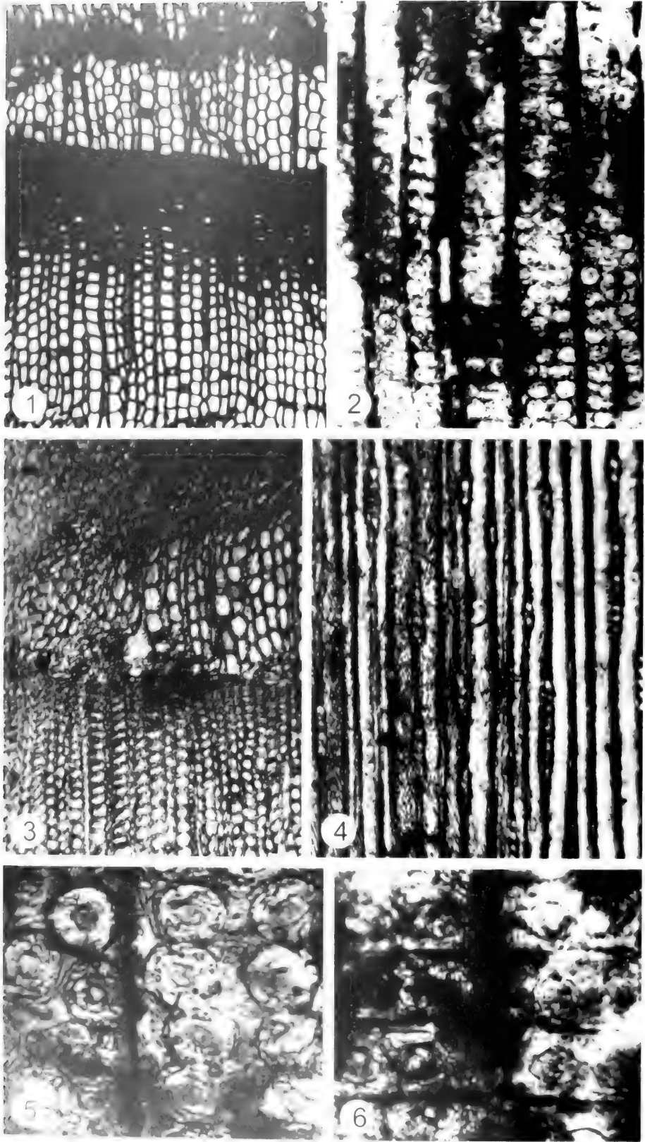
1 横切面, \times 80 ; 2 径切面, 示管胞壁具缘纹孔2-3列, \times 200 ; 3 横切面, 示细胞形态, \times 120 ; 4 径切面, 示射线形态, \times 120 ; 5 径切面, 示射线, \times 1000 ; 6 径切面, 示射线, \times 1000
