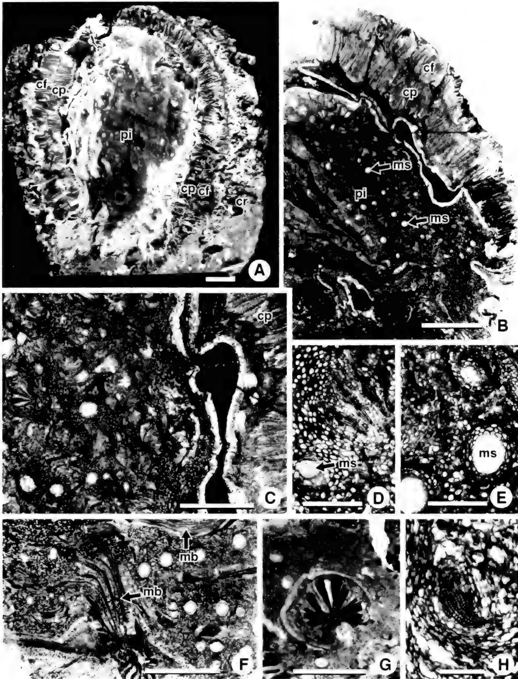
图版5-2 辽宁李氏木 Lioxylon liaoningense Zhang, Wang, Saiki, Li et Zheng
