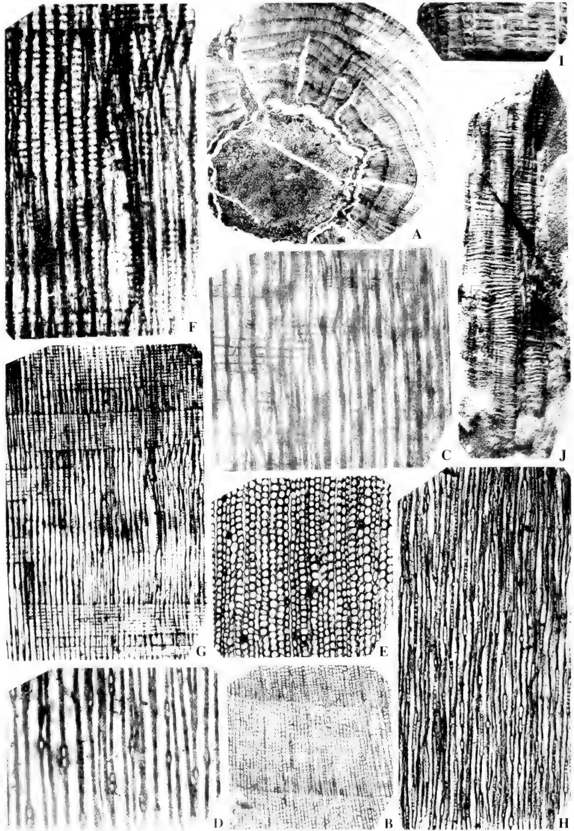
3-17 李氏南洋杉型木 Araucarioxylon leei (Sze) Wang I. 径切面，示管胞径向壁纹孔单列， \times 102 ；G. 径切面，示木管胞壁厚，1~22个细胞高， \times 36 ；H. 径切面，示木管胞壁厚，1~22个细胞高， \times 36 ；F. 径切面，示管胞径向壁纹孔单列， \times 102 ；E. 径切面，示管胞径向壁纹孔单列， \times 102 ；D. 径切面，示管胞径向壁纹孔单列， \times 102 ；C. 径切面，示管胞径向壁纹孔单列， \times 102 ；B. 径切面，示管胞径向壁纹孔单列， \times 102 ；A. 径切面，示管胞径向壁纹孔单列， \times 102 。
