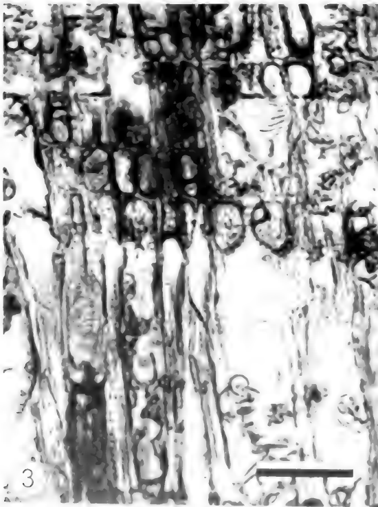
图 1 Phellodendron chinense 纵切面
