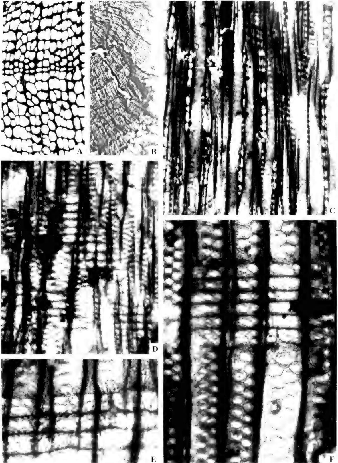
A-B. 横切面，示管胞形态轮廓和微弱的生长轮，A×66，B×13；C. 弦切面，示单列射线和伸长的射线细胞，×165；D-F. 径切面，示径向壁纹孔紧挤、多角形和交叉场纹孔，每场1~4个，简单，不具缘，D×165，E-F×329（标本与薄片保存在沈阳地质矿产研究所）
