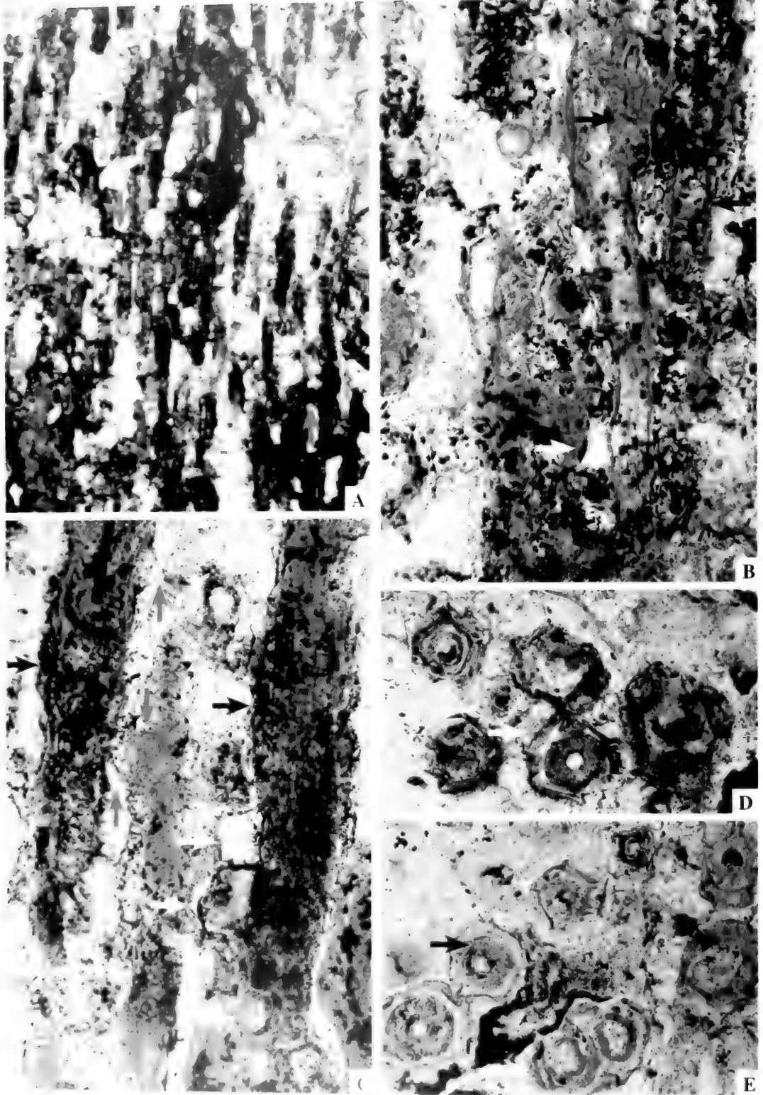
图 1 菌丝之间的横向通道 (红色箭头所指), \times 305 ; A-B. 纵切面, 示菌丝和其外的多角形厚壁细胞 (白色箭头所指), \times 152 ; C. 纵切面, 示菌丝之间的横向通道 (红色箭头所指), \times 305 ; D-E. 横切面, 示厚壁细胞 (白色箭头所指), \times 305 , A-E 标本编号:
