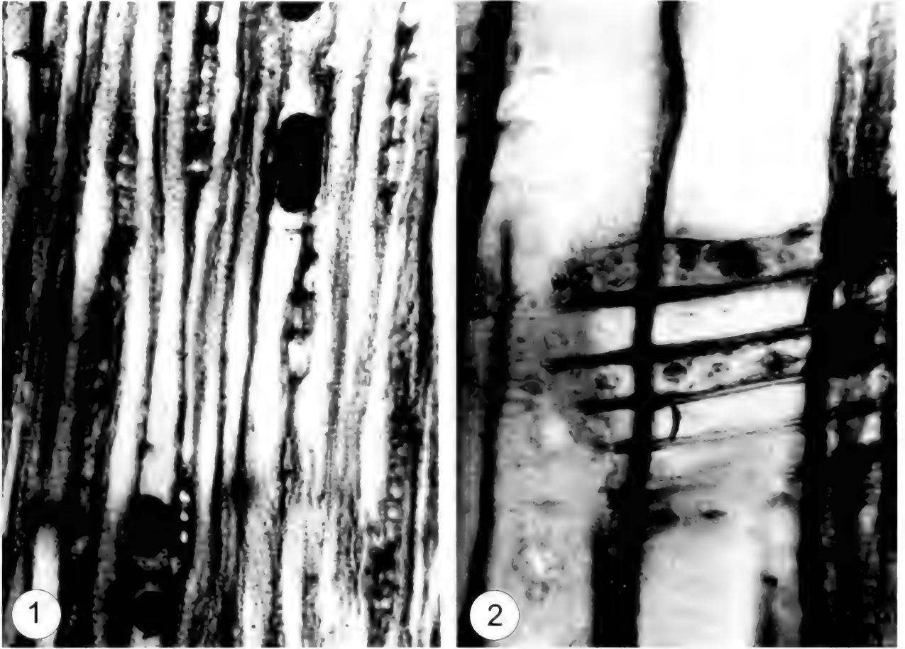
1 弦切面，示射线高度及轴向薄壁细胞端壁平滑， \times 100 ；2 径切面，示交叉场纹孔杉木型， \times 350
