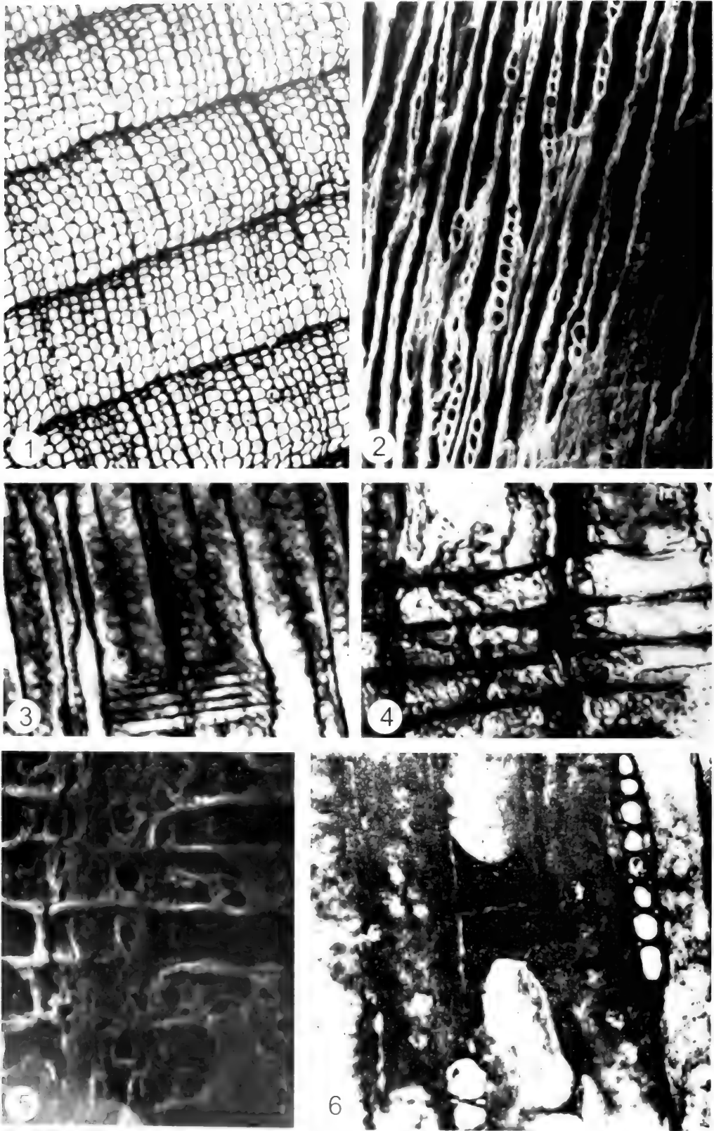
图 1 茎横切面, \times 80 ; 2 弦切面(SEM), 示射线高度, \times 360 ; 3 径切面, 示维管束排列, \times 120 ; 4 径切面, 示维管束排列, \times 120 ; 5 径切面(SEM), 示交叉场纹孔柏木型, \times 300 ; 6 茎横切面, 示维管束排列, \times 120
