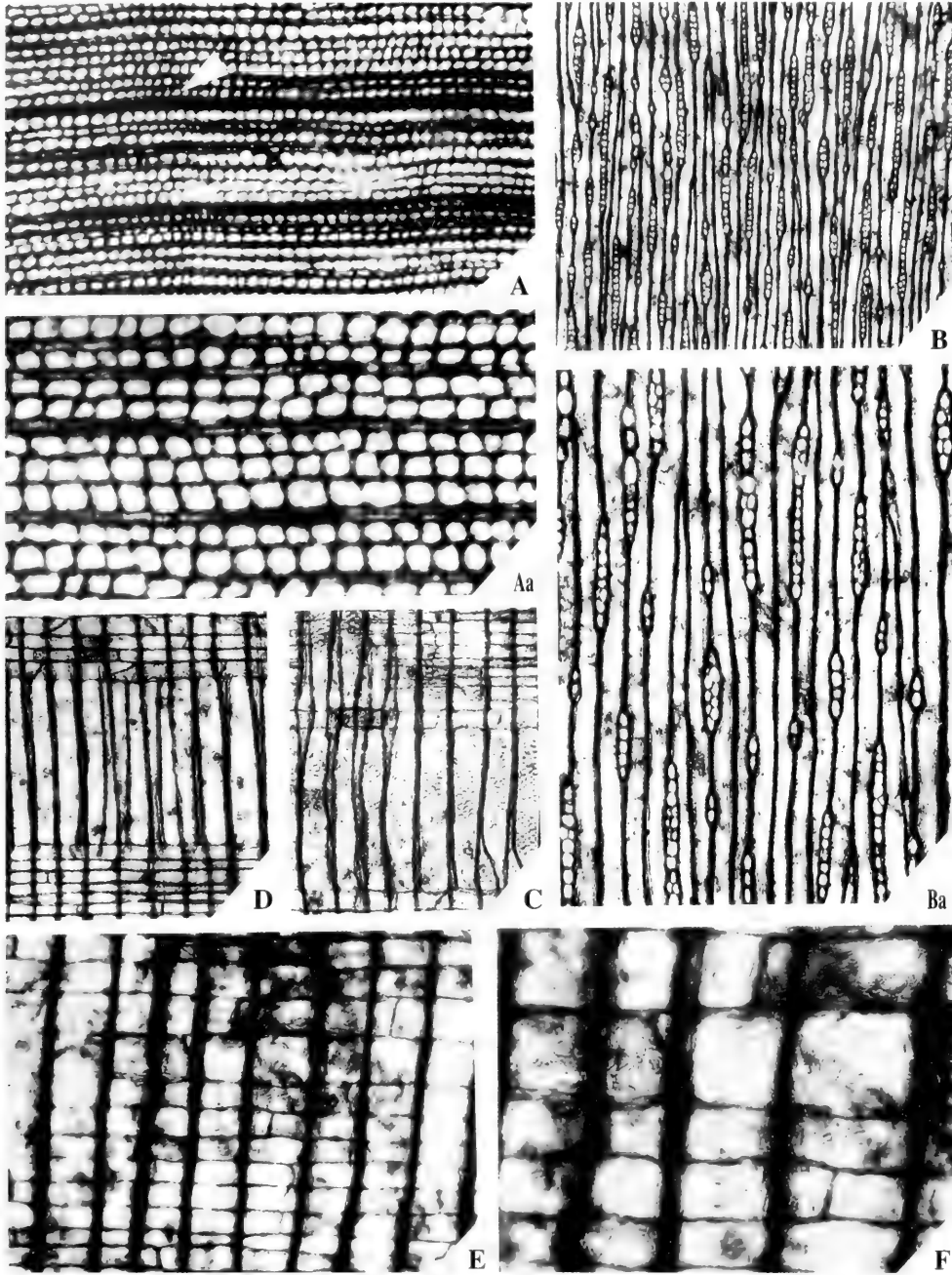
3-17 特尔哈德查普曼木 Chapmanoxylon? teilhardii (Sze) Wang
