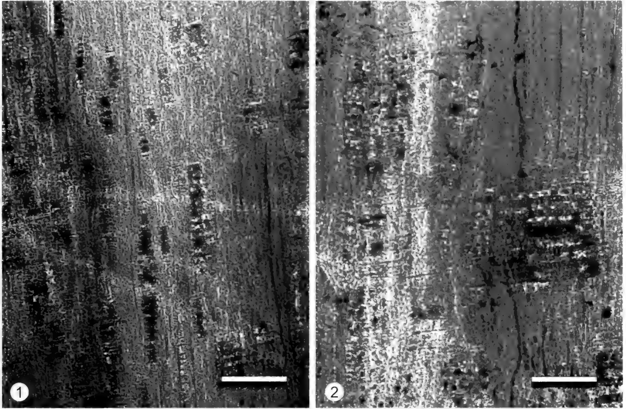
1 弦切面，示射线形态，标尺400 μm；2 径切面，示射线和交叉场，标尺200 μm。
