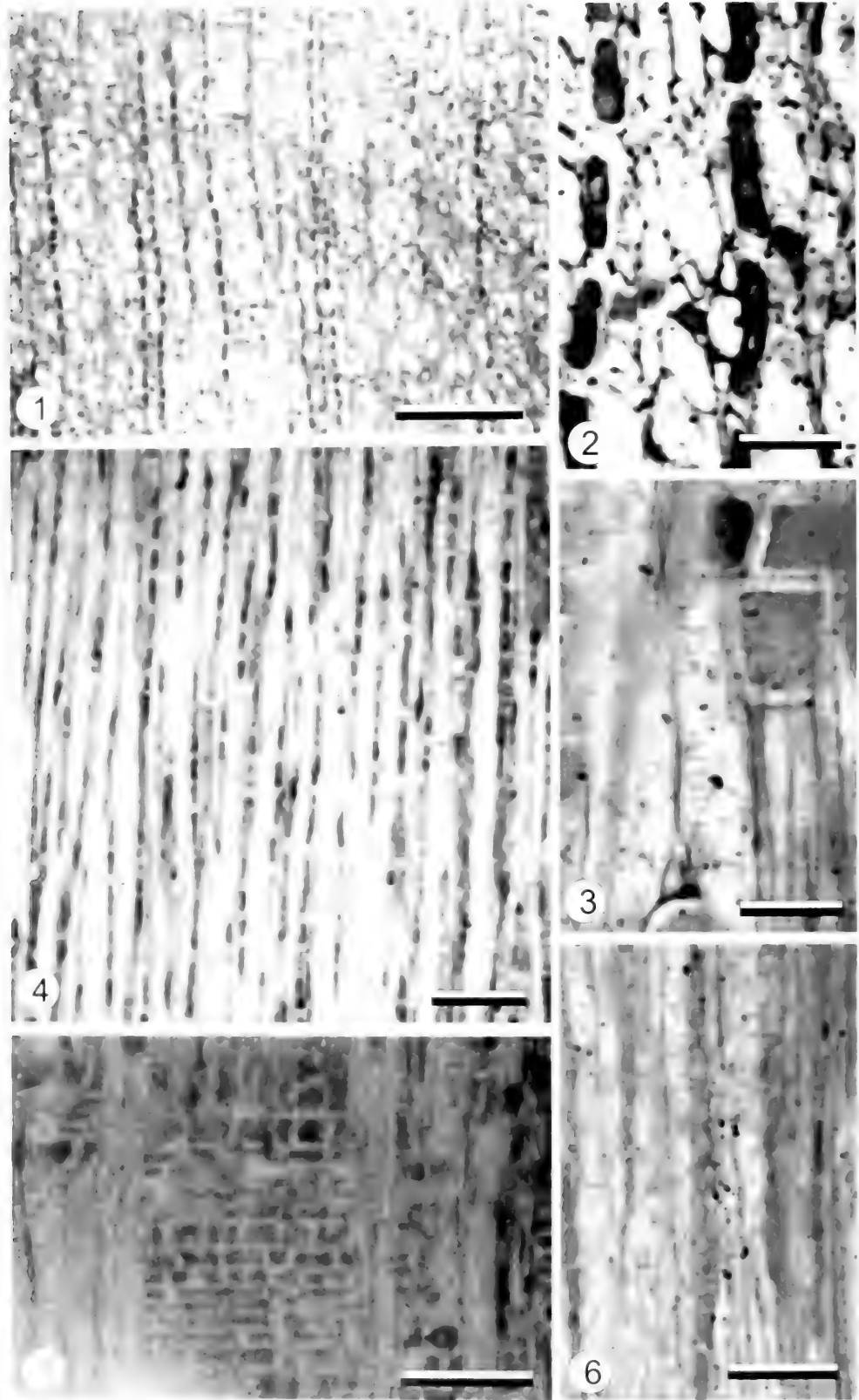
1 茎纵切面，示维管束分布，标尺0.4 mm；2 横切面，示导管被挤压，轮廓多角形，标尺50 μm；3 茎纵切面，示射线单列，2列，极少3列，标尺0.4 mm；4 茎纵切面，示射线单列，2列，极少3列，标尺0.4 mm；5 径切面，示射线单列，2列，极少3列，标尺100 μm；6 茎纵切面，示多列射线多数宽于单列射线，100 μm
