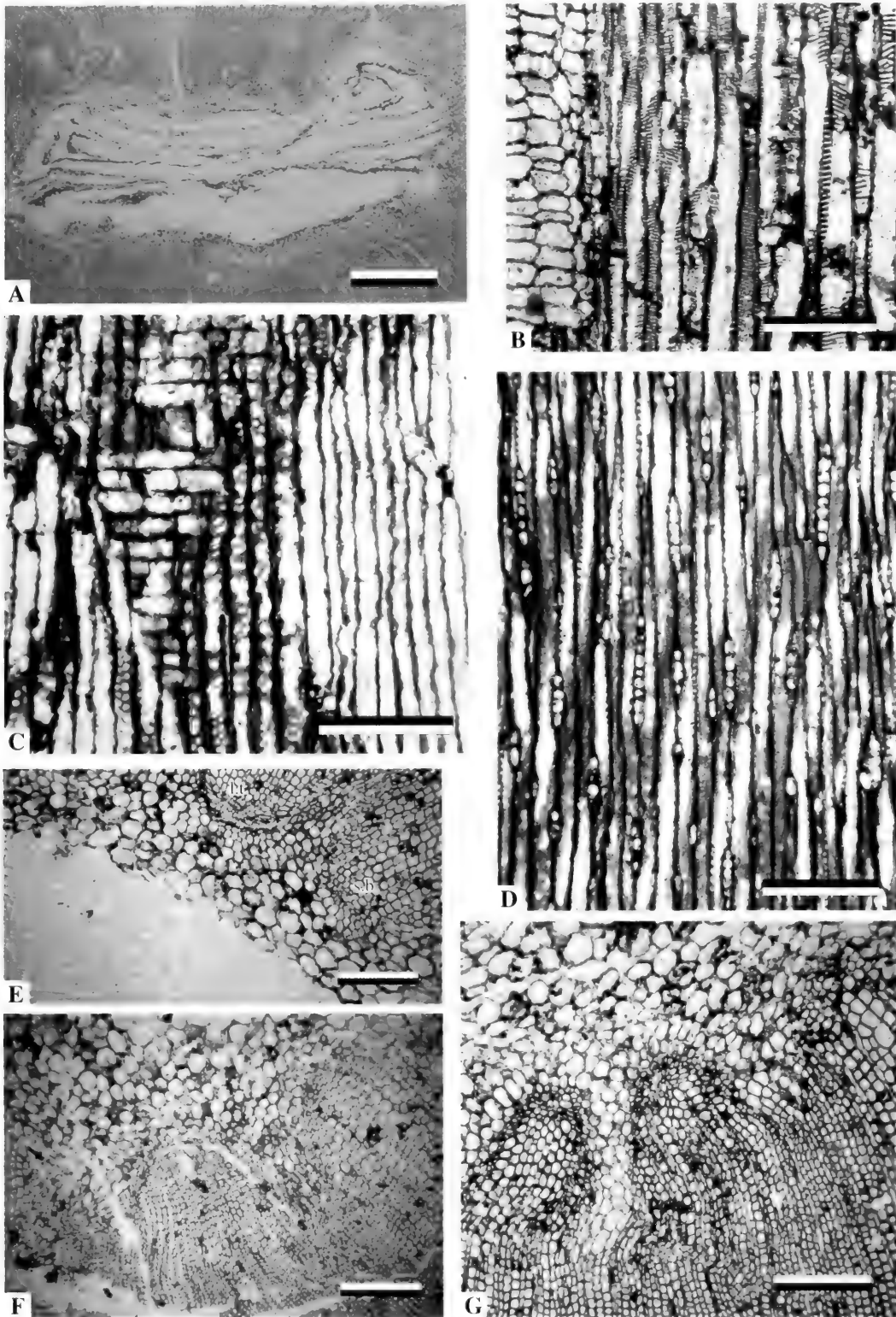
A. 横切面，示髓膜和髓腔，标尺30 mm；B. 径切面，示初生木质部管胞及射线薄壁细胞，标尺200 μm；C. 径切面，示次生木质部管胞壁上的纹孔，射线以及交叉场纹孔，标尺200 μm；D. 弦切面，射线高度，标尺200 μm；E. 横切面，示茎维管束 (s.b) 和一个中始式单叶迹 (l.t)，标尺400 μm；F. 横切面，示叶迹 (l.t) 已经开始分裂为双叶迹，标尺400 μm；G. 横切面，示一枚大的双叶迹，标尺400 μm
