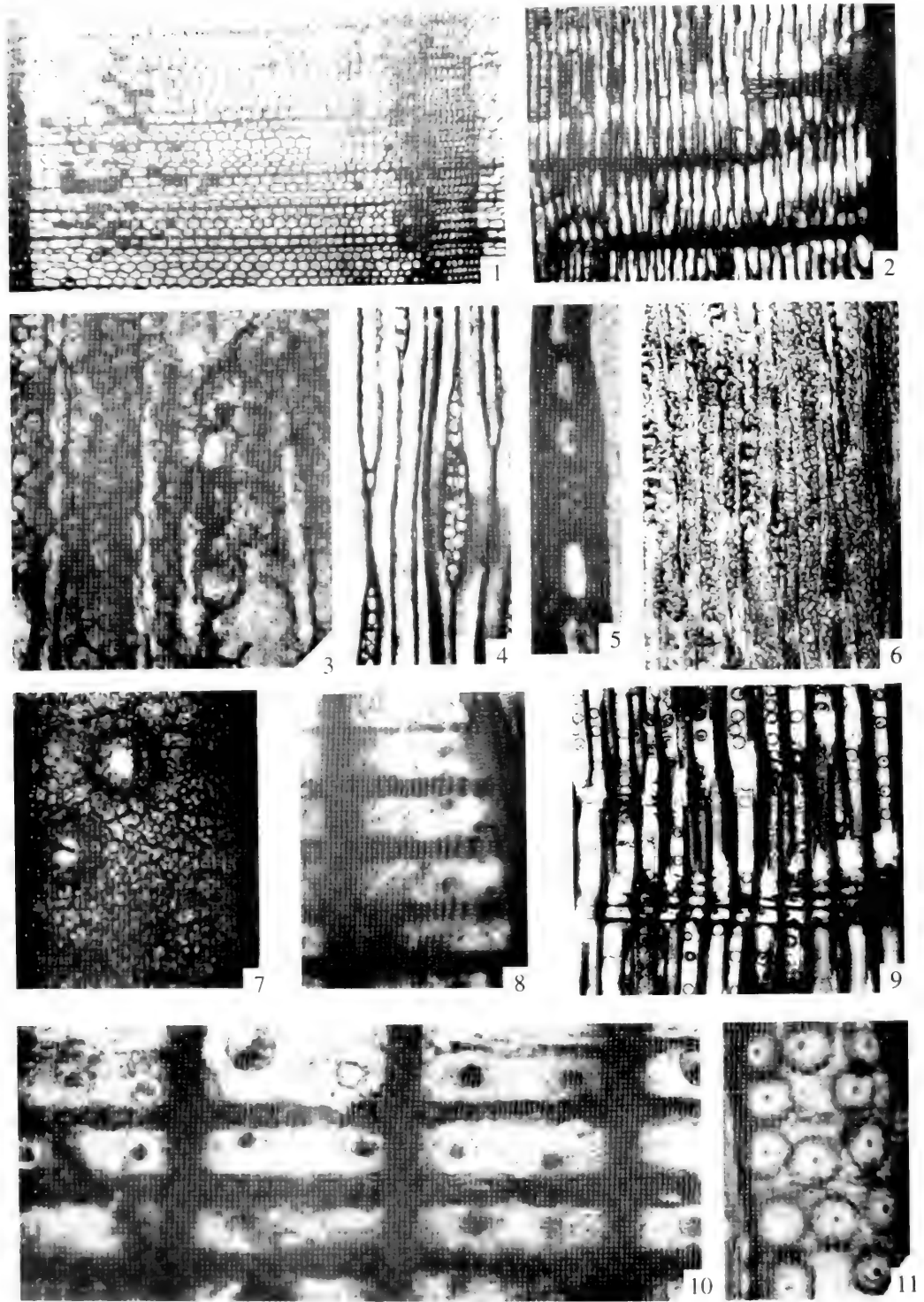
图 11 1 纵切面, \times 32 ; 2 径切面, 示早、晚材及髓线 \times 32 ; 7, 9, 11 径切面, 示管胞径壁的具缘纹孔 \times 100 ; 3, 6 弦切面, 示管胞壁上不规则的网纹加厚 \times 400 , \times 100 ; 4 弦切面, 示双列管胞 \times 100 ; 5 弦切面, 示射线细胞壁上的小孔 \times 400 ; 8, 10 径切面, 示交叉场纹孔及髓射线细胞壁横壁 \times 100
