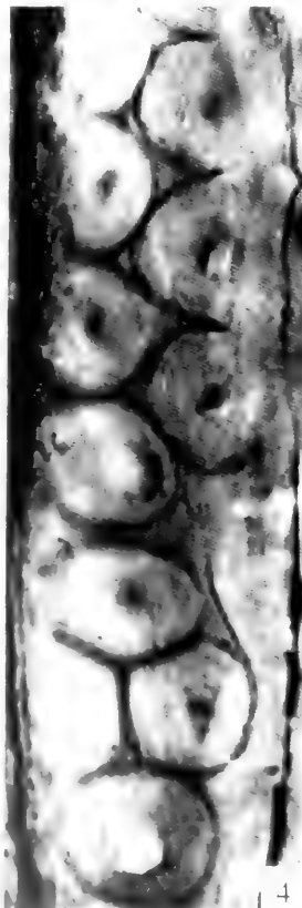
1 68; 2 横切面, 示早材交叉场纹孔 \times 350 ; 3 弦切面, 示射 350; 4 径切面, 示径向管胞壁具缘纹孔 \times 700 ; 5 175
