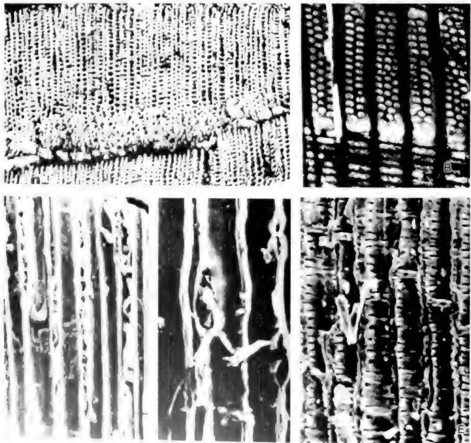
A. 径向切面, 示径壁纹孔和交叉场, \times 104 ; C. 弦切面, 扫描电镜照片, \times 104 ; D. 弦切面, 示射线细胞, 扫描电镜照片, \times 450 ; E. 弦切面, 示射线细胞, 扫描电镜照片, \times 450
