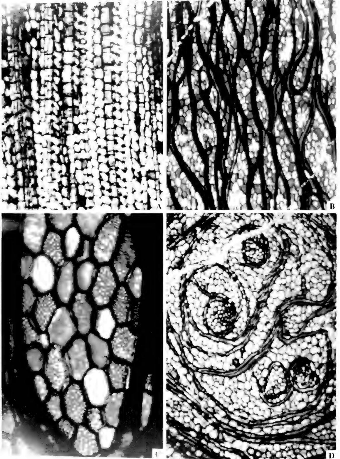
图 1. A. 皮层散在分布的深色细胞, \times 32 ; B-D. 弦切 C. 射线细胞上的各种形态的小孔或网纹; D. D. 158. 薄片编号: DFT-6 (标本与薄片保
