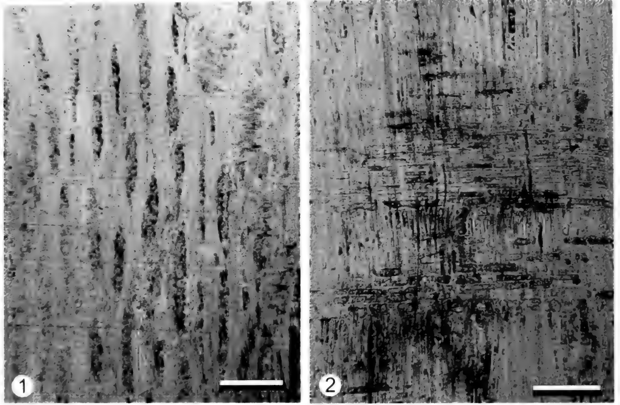
1 弦切面，示单列和多列射线，标尺400 \mu\text{m} ；2 径切面，示射线异型，标尺200 \mu\text{m} 。
