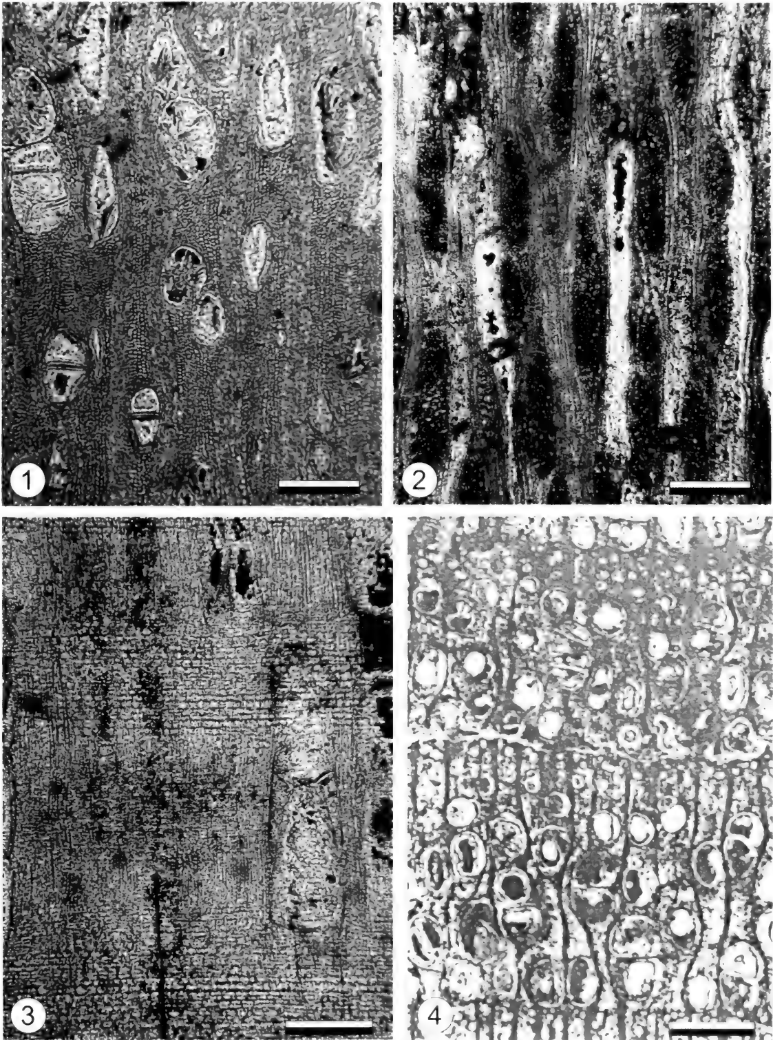
图版7-49 湖北石梓 Gmelina hubeiensis
