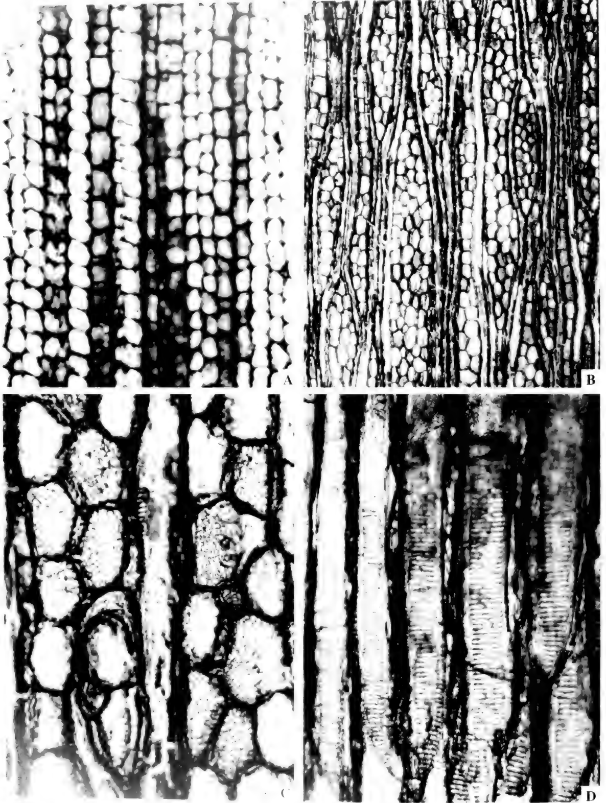
图 161 32. 薄片编号: DFT-17a B-C. 弦切面, 161. C. 木质部细胞为多角形, 侧壁加厚, 表壁多孔并具纹孔, 161; 薄片编号: DFT-17 (标
