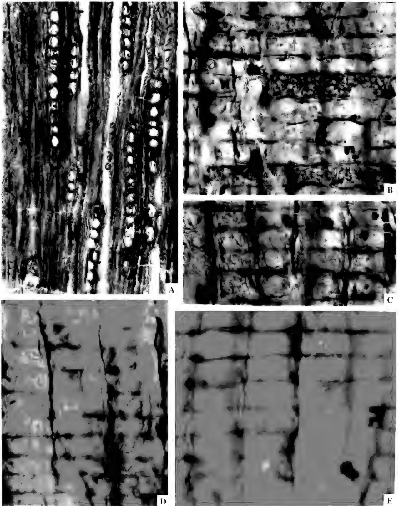
A. 纵切面，显示同心射线和简单具孔， \times 175 ；B-E. 径切面，示交叉场纹孔柏木型、云杉型，多数1-2个、多数1-2个、多数1-2个、多数1-2个，有的射线中充填深色物质， \times 350 ，标本编号：GJ6-22 石炭纪—二叠纪植物化石，南京地质古生物研究所
