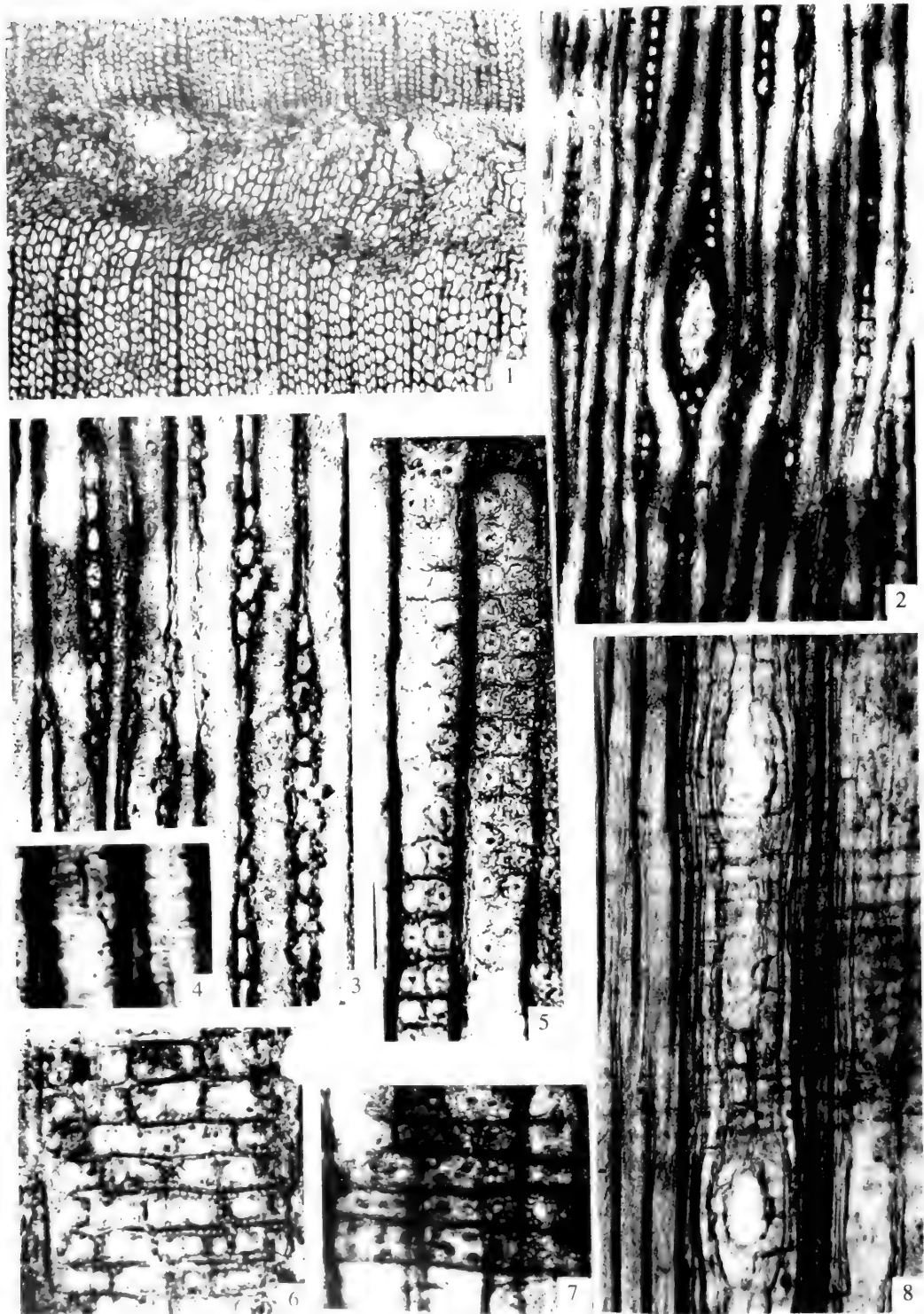
1 横切面，示生长轮、轴向正常树脂道 \times 68 ；2 弦切面，示木射线、横向创伤树脂道及纺锤形木射线 \times 175 ；3 弦切面，示木射线形态、三角形胞间隙及弦向壁纹孔 \times 350 ；4 径切面，示径向次生梯纹加厚 \times 700 ；5 弦切面，示径向射线具缘纹孔对生和树脂道 \times 350 ；6 径切面，交叉场纹孔松木型及射线细胞水平壁 \times 350 ；7 弦切面，示交叉场纹孔松木型 \times 700 ；8 径切面，示径向创伤树脂道 \times 68
