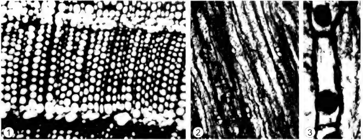
1 横切面, 示生长轮明显, 早材至晚材渐变, \times 90 ; 2 弦切面, 示射线高度, \times 120 ; 3 径切面, 示轴向木薄壁组织, \times 480 。
