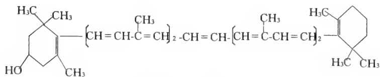
Cryptoxanthin m. 169°C
