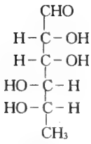
直链式
