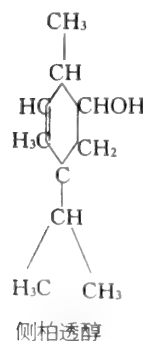
Thujon b. 200 ~ 202°C
