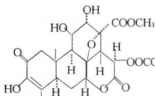
鸦胆子苦醇
