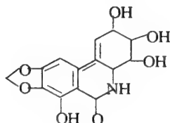
Lycoricidinol
