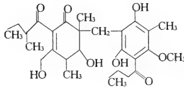
鹤草酚
