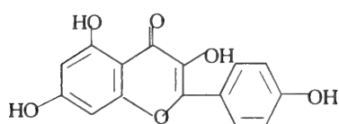
Kaempferol
