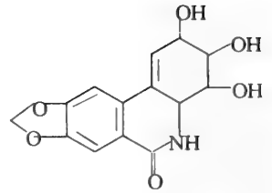
m. 214.5~5.5°C Lycoricidine
