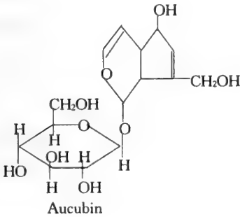
Aucubin
