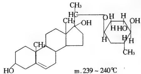
m. 239~240 ^{\circ} C Glycoside E(periplocae)
