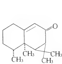
m. 100 ~ 101℃ Aristolone
