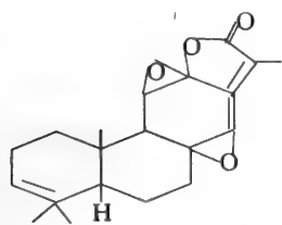
Jolkinolide
