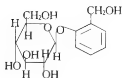
Salicin
