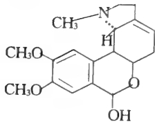
m. 198~200° Lycorenine
