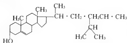
\Delta^7 -Campesterol m. 157 ~ 158°C
