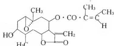
Heliangine m. 227 ~ 229°C
