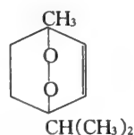
Ascaridole
