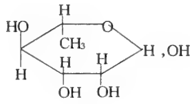
吡喃式
