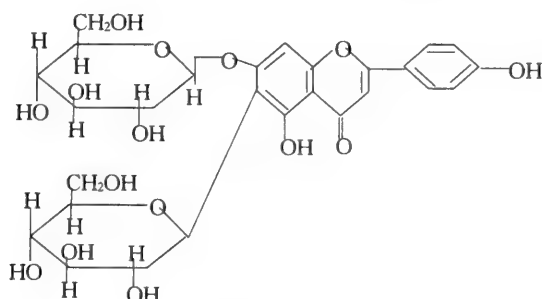
Saponarin
