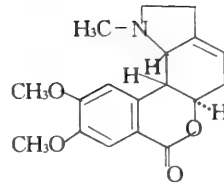
m. 175°C Homolycorin
