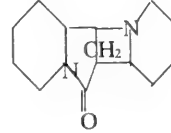
去氢毒藜素
