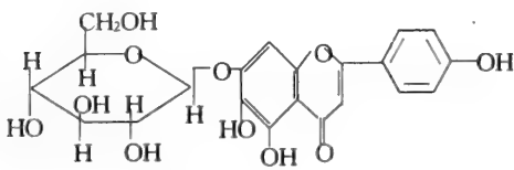
Plantaginin
