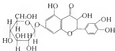
Quercimeritrin m. 247 ~ 249°C
