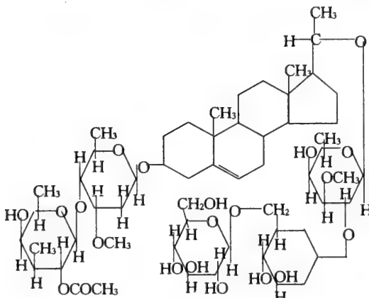
Glycoside H (periplocae) m. 182 ^{\circ} C
