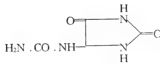
m. 238 ~ 240℃ Allantoin
