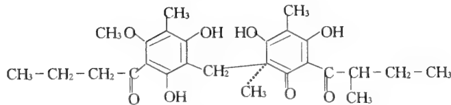
Agrimopholum
