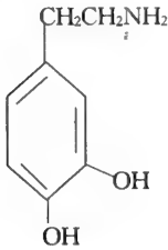
Dopamine
