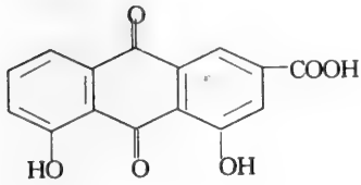
Rhein
