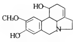
Norpluviine
