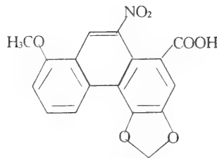
m. 287 ~ 292℃ (分解) Aristolochic acid
