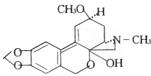
m. 210~211°C Tazettine
