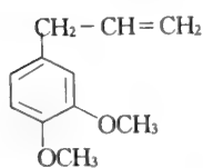
甲基丁香酚
