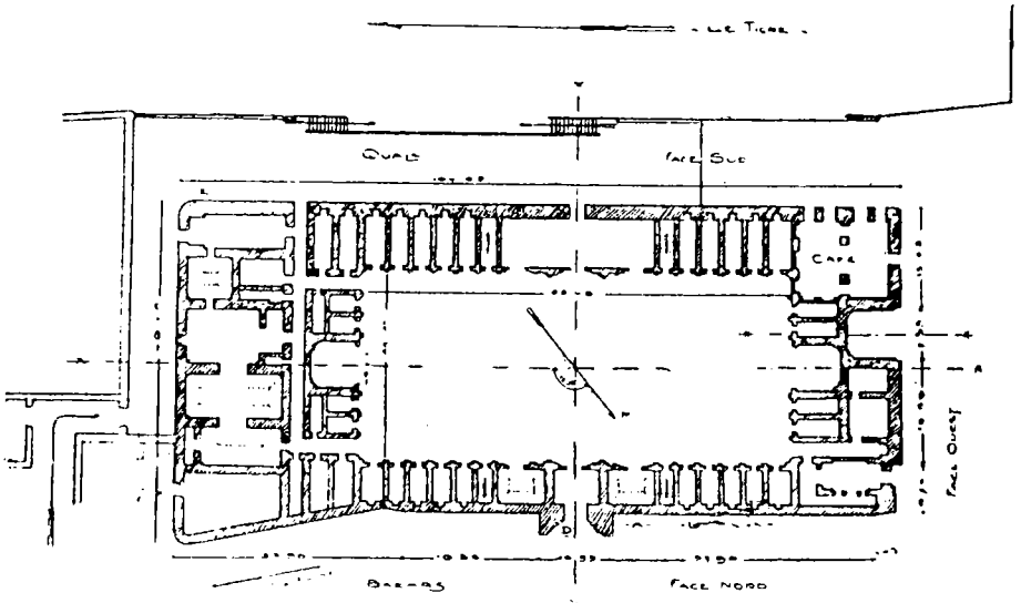
(الشكل 2) المستنصرية - مخطط الطبقة السفلى من المستنصرية (عن فيوله)
