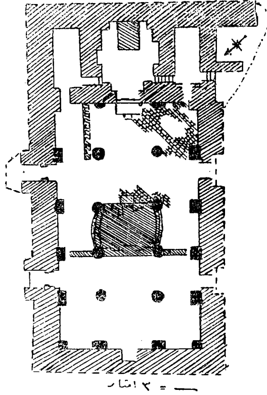
الشكل - 6 - مخطط الكنيسة المكتشفة في التل الحادي عشر بالحيرة (عن تلبت رايس)
