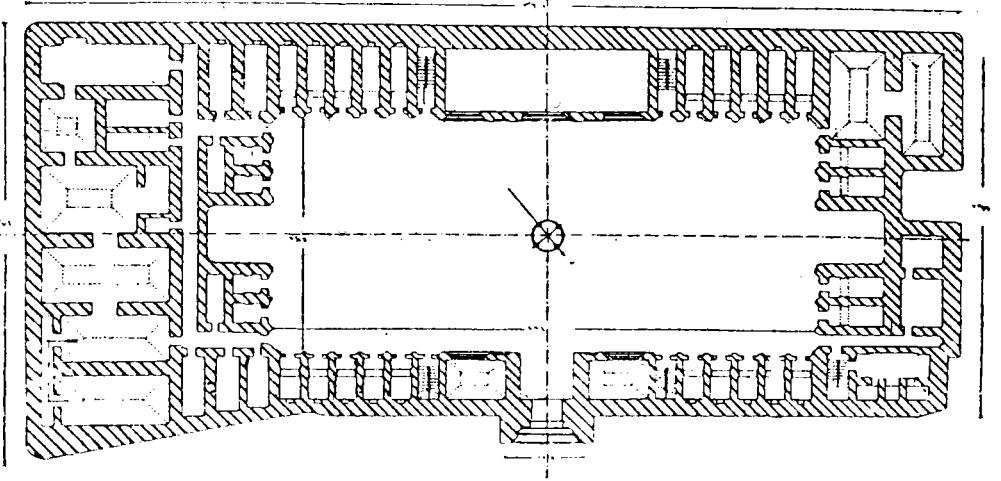
(الشكل 1) المستنصرية - مخطط الطبقة السفلى من المستنصرية
