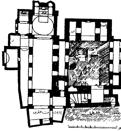
الشكل - 2 - مخطط كنيسة شمعون الصفا بالموصل (عن هرتسفلد).
