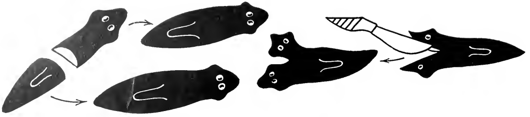
Fig. 9-7. Regeneration in planaria.
