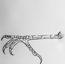
Fig. 6. Z. japonica . (1.).
