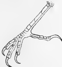
Fig. 7. Z. strenua . (1.).
