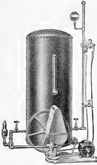
Fig. 1355-A Pump
