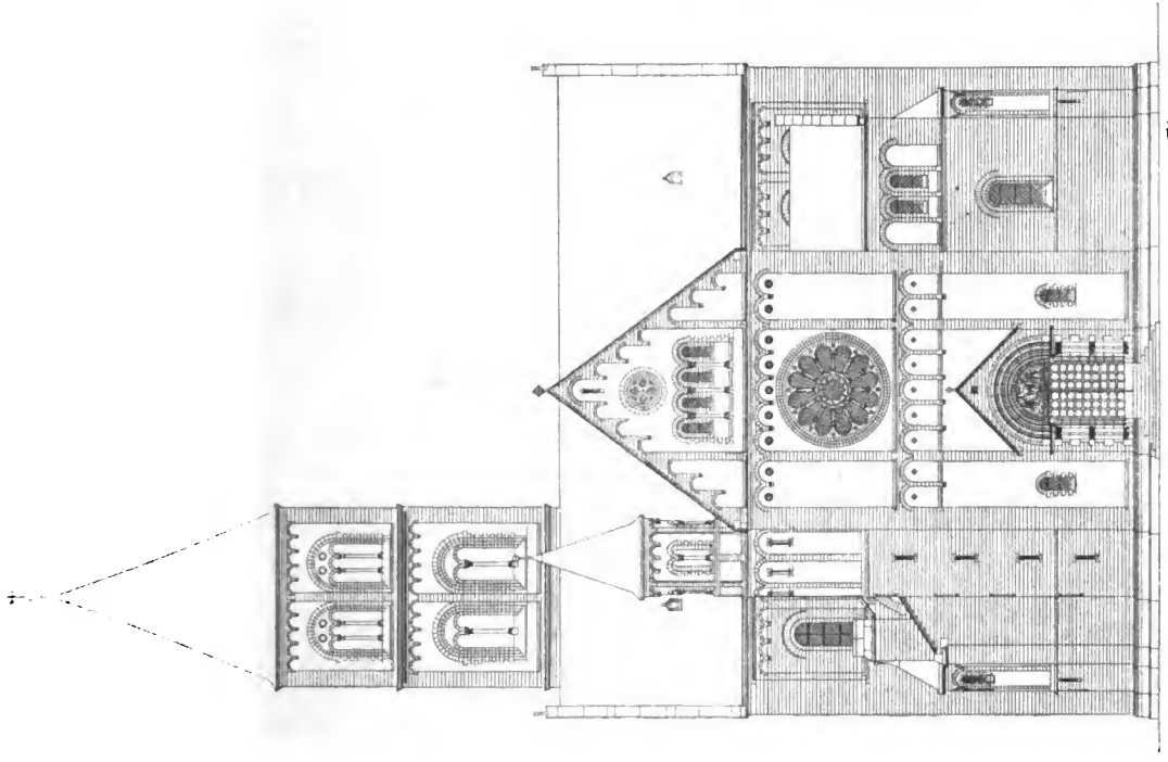
Giebelansicht.
