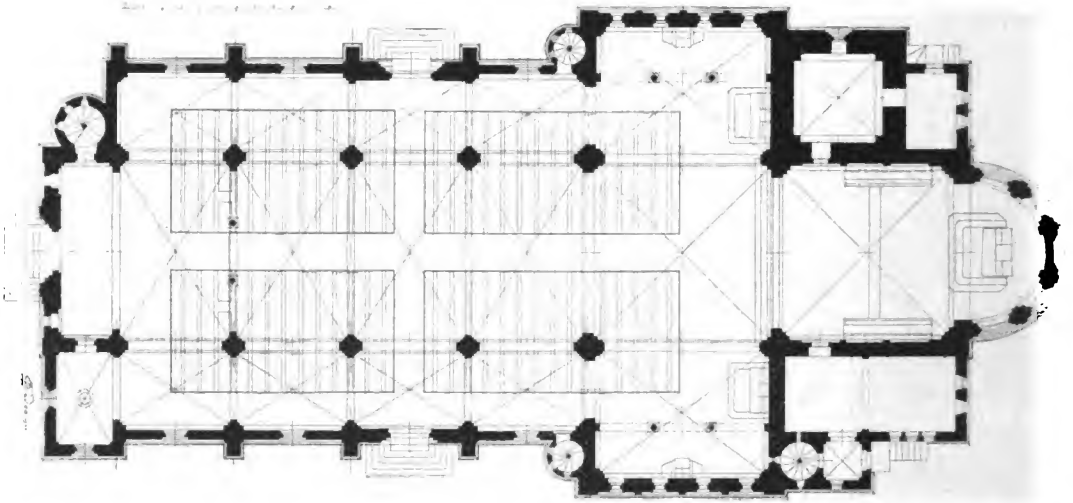
Grundriss.
