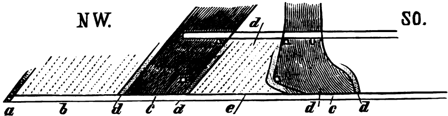
Profil eines Sattels der Braunkohlengrube „Präsident“.
