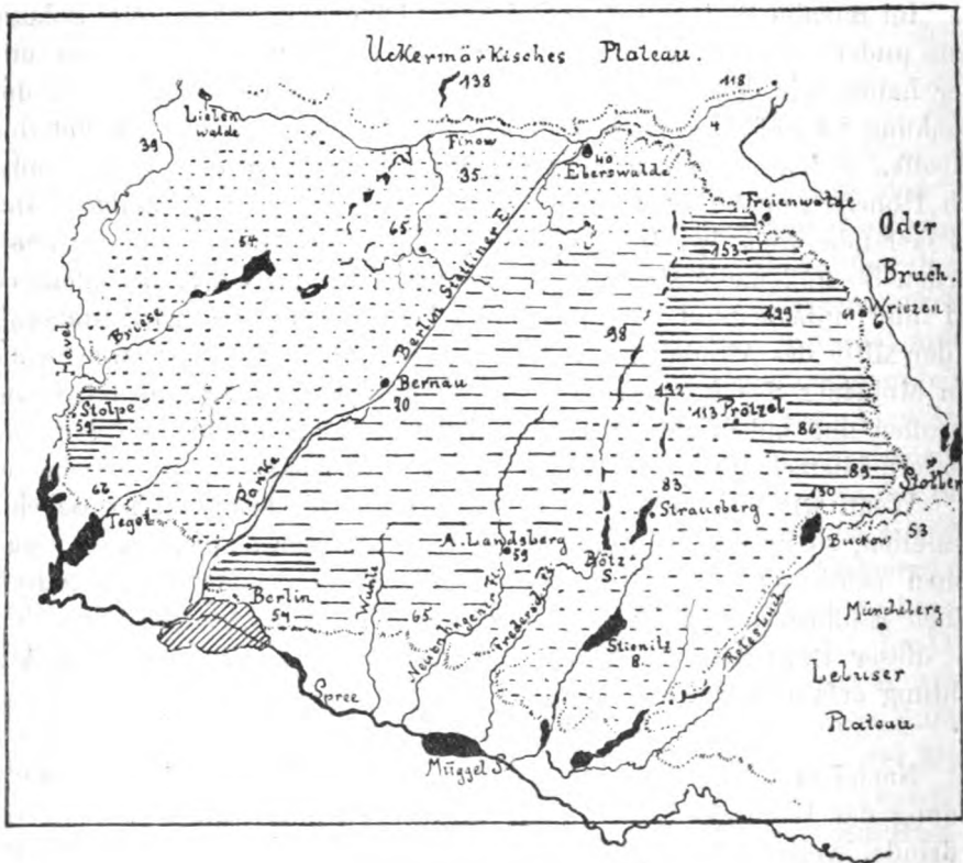
Geognostische Skizze des Barnim-Plateaus.
