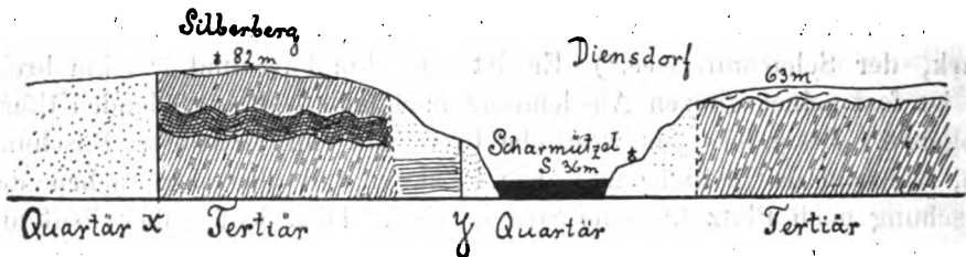
Schematisches Profil durch den Scharmützel-See bei Fürstenwalde.
