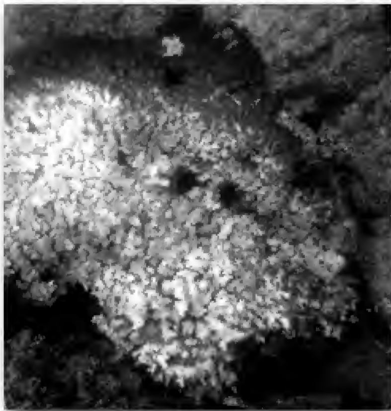
Figura 3. Una de las consecuencias de la bioerosión por esponjas es el debilitamiento del esqueleto de los corales, que se pueden desprender del arrecife. En la imagen, un coral del género Pocillopora desprendido del sustrato. Se puede apreciar el sofocamiento de los pólipos al volcarse la colonia (zona blanquecina).
