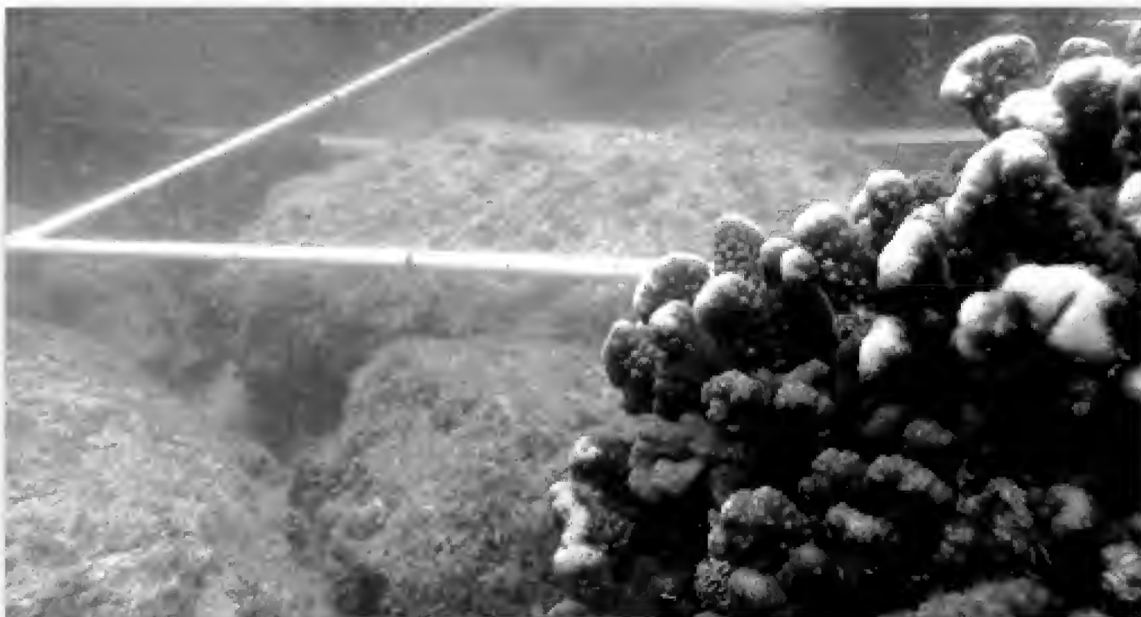
Figura 6. El arrecife de Playa Las Gatas ha soportado el efecto de las actividades humanas durante las últimas décadas. Actualmente sólo quedan remanentes de la estructura arrecifal original, creciendo sobre bloques de piedra de hasta dos metros de diámetro.
