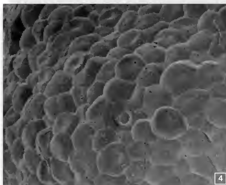
Figura 2. Detalle de las excavaciones hechas por esponjas bioerosionadoras en corales. Estas esponjas mantienen comunicación con el exterior abriendo orificios en el sustrato (1). Vista de las cámaras y galerías excavadas en el interior de un coral (2). Microfotografías de las marcas dejadas por las esponjas en el sustrato (3 y 4). 1
