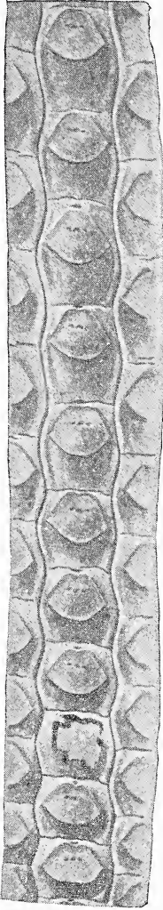
Fig. 6. Sigillarie, die durch Quersfurchen noch die Polstergrenzen zu erkennen giebt.
