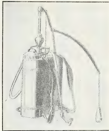
ナブサツク スプレーヤ Knapsack Sprayer
