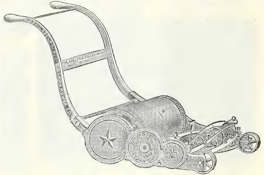
ローンモーター四號 Lawn Mower No. 4
