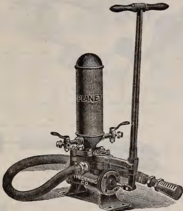
Fig. 610. Planet Pump.
