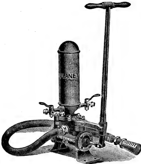
Fig. 610. Planet Pump.
