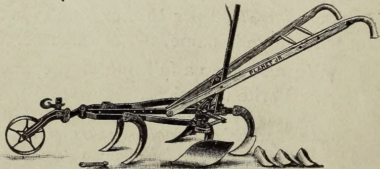
PLANET JR. No. 9. Horse Hoe.
