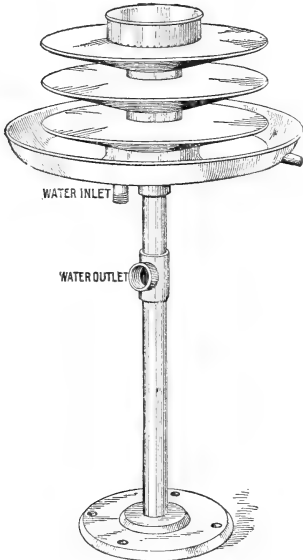
Cooler.
