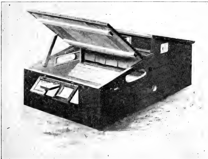
Out Door Brooder, Style A (Rear View.)
