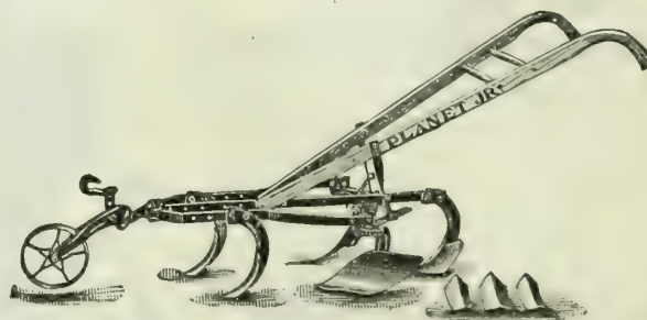
No. 4 Planet Jr. Horse Hoe
