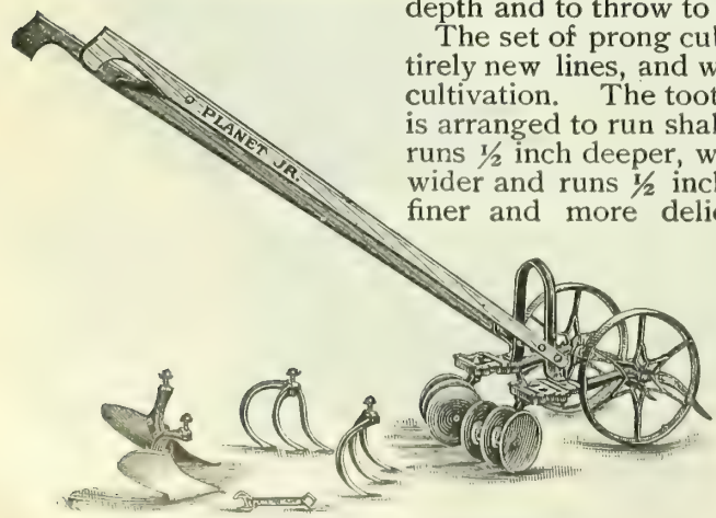
No. 14 Planet Jr. Wheel Hoe
