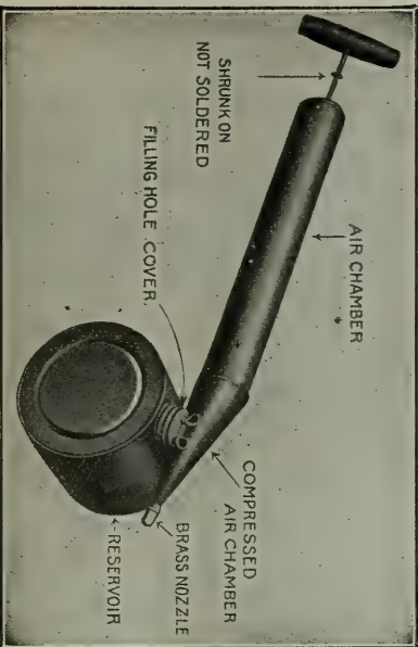
U. T. K. Continuous Sprayer
