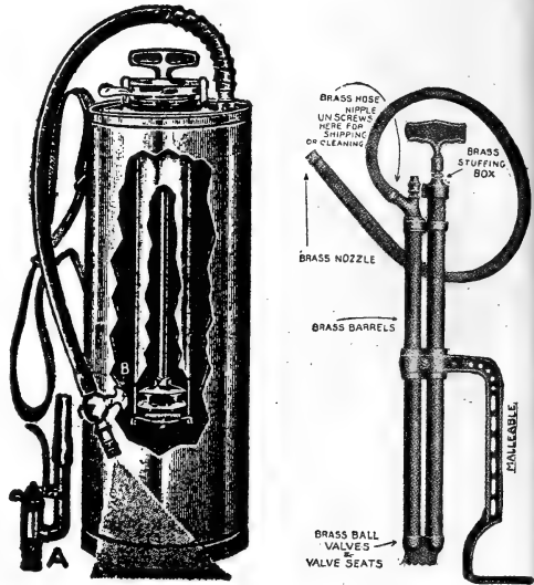
O. K. Bucket Pump.
