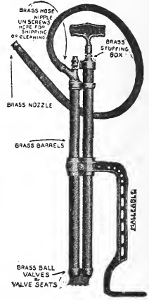
O. K. Bucket Pump
