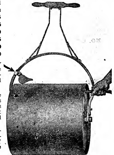
Dunham Lawn Roller
