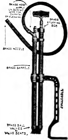
O. K. Bucket Pump
