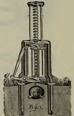
Olmstead Mole Trap
