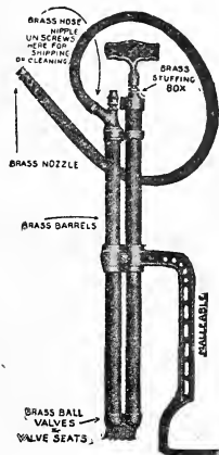
Price $5.00 O. K. Bucket Pump
